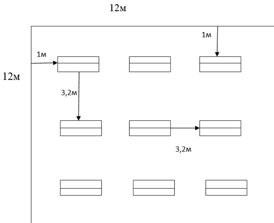
Рисунок 5 – План размещения светильников на потолке помещения
