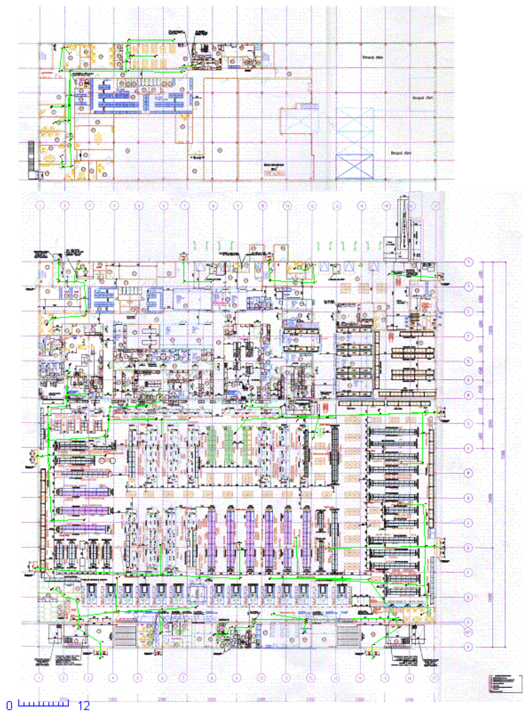
Рисунок А1 – Пути эвакуации
