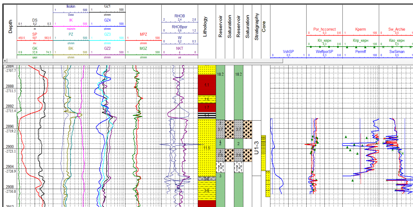
Рис. 4.8. Планшет с коррелированными кривыми скважины № 59
