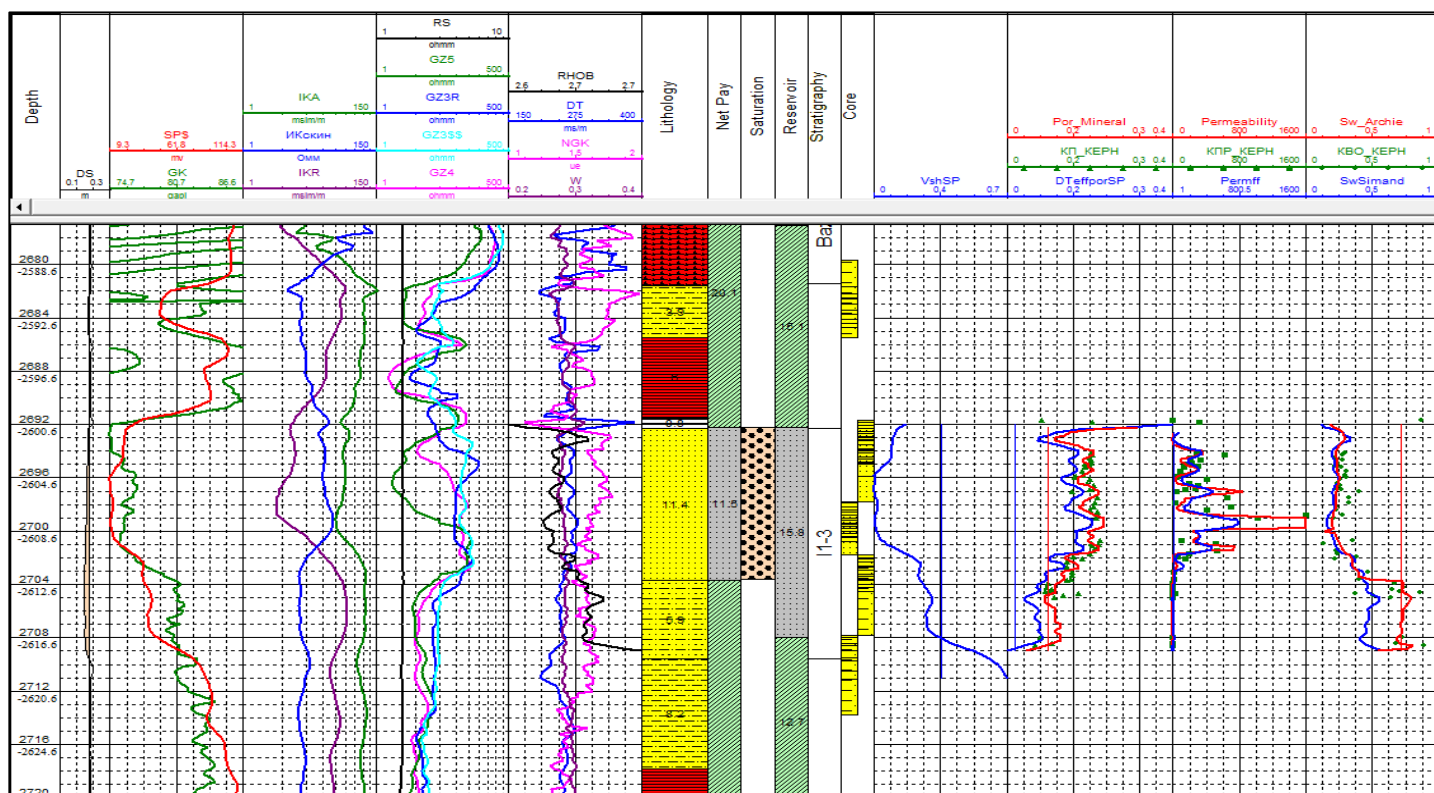
Рис. 4.6. Планшет с коррелированными кривыми скважины № 208
