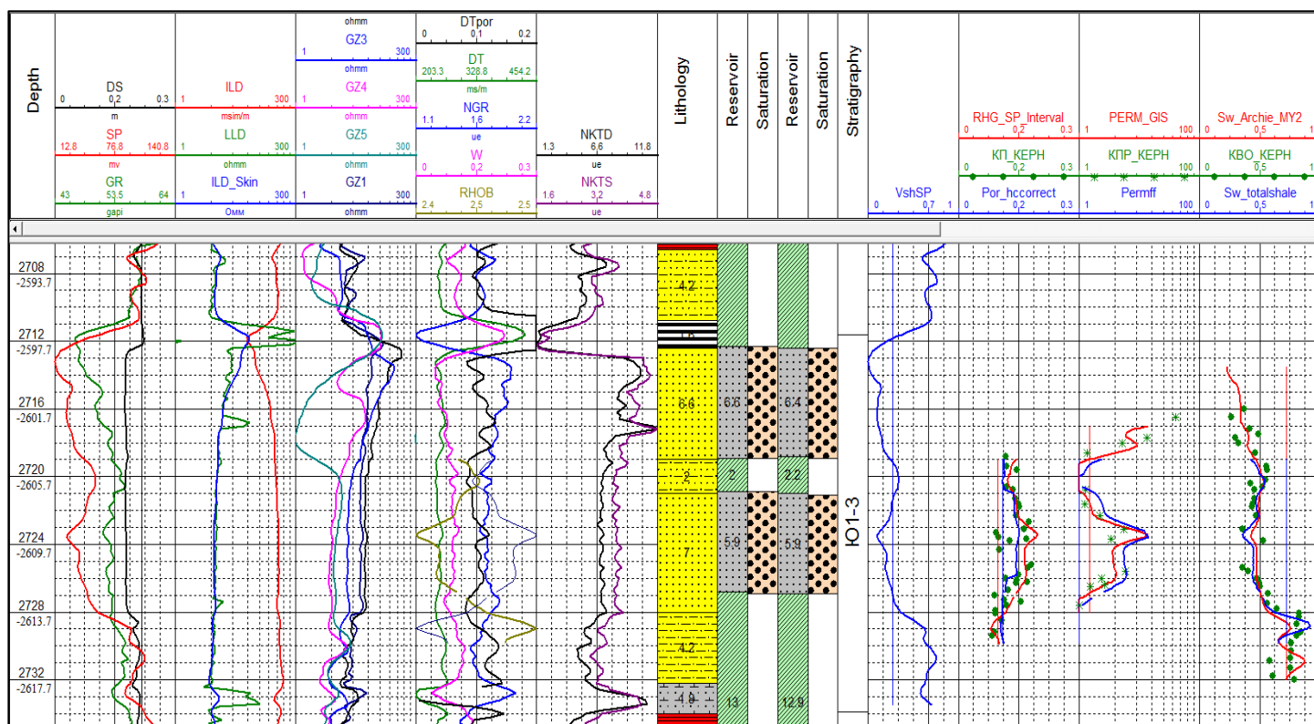
Рис. 4.7. Планшет с коррелированными кривыми скважины № 203
