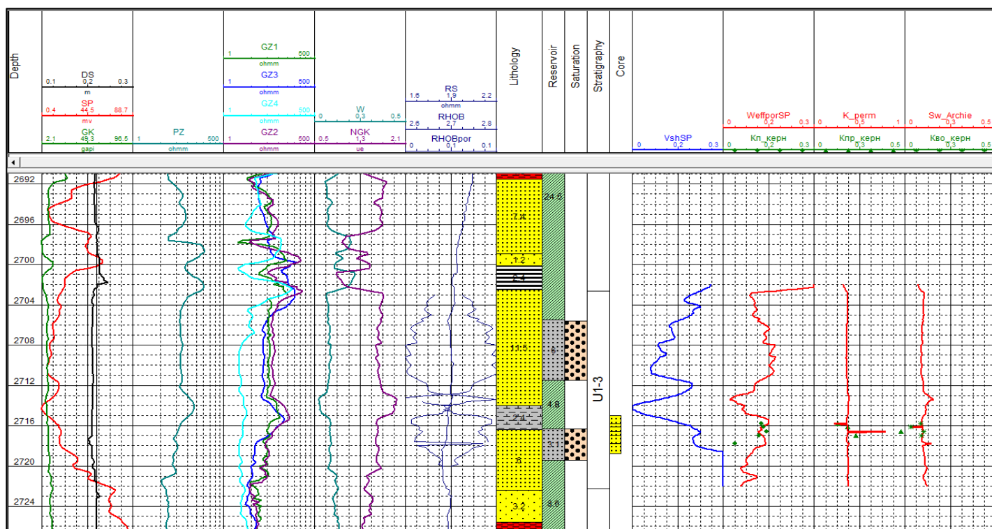
Рис. 4.11. Планшет с коррелированными кривыми скважины № 196
