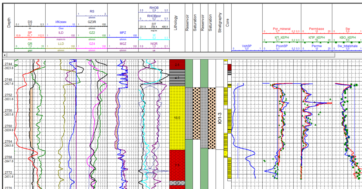
Рис. 4.1. Готовый планшет с коррелированными кривыми скважины № 220
