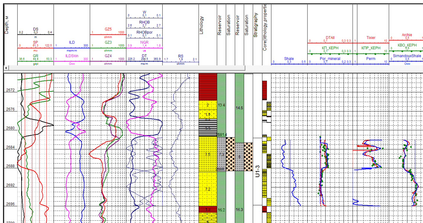
Рис. 4.3. Готовый планшет с коррелированными кривыми скважины № 197
