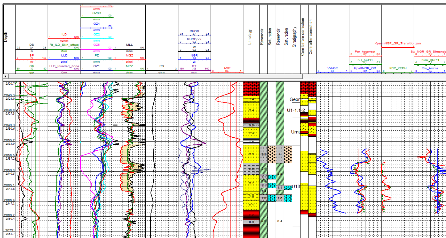
Рис. 4.9. Планшет с коррелированными кривыми скважины № 191
