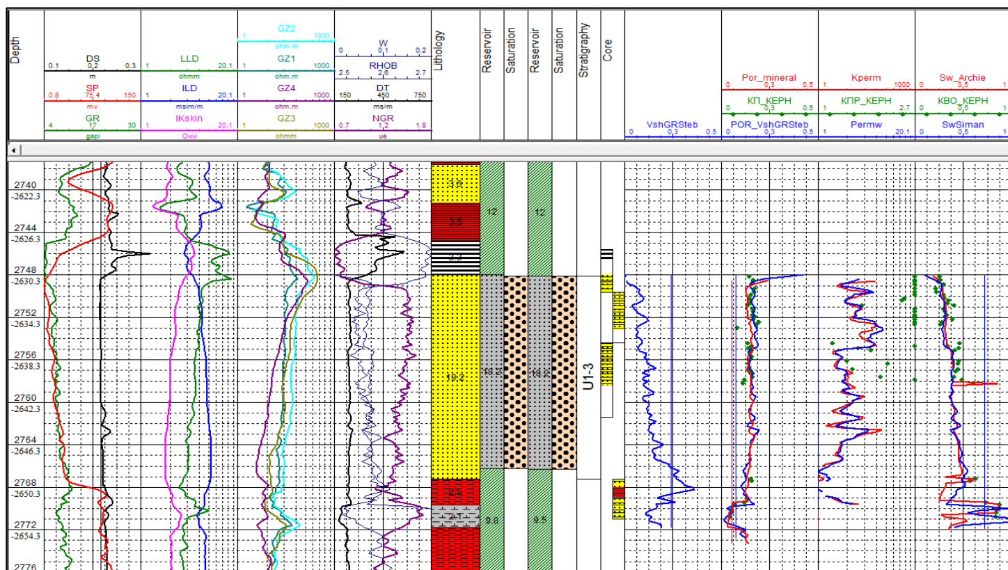
Рис. 4.2. Готовый планшет с коррелированными кривыми скважины № 223
