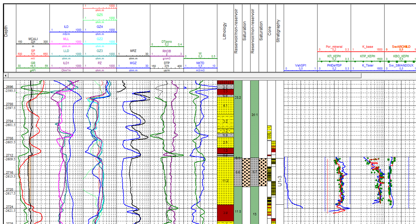
Рис. 4.4. Готовый планшет с коррелированными кривыми скважины № 218
