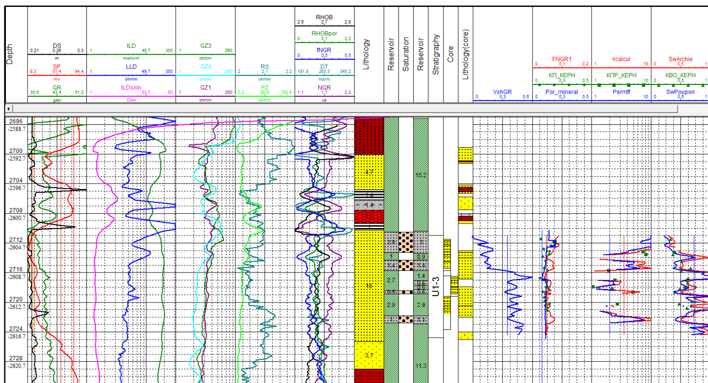
Рис. 4.5. Планшет с коррелированными кривыми скважины № 202
