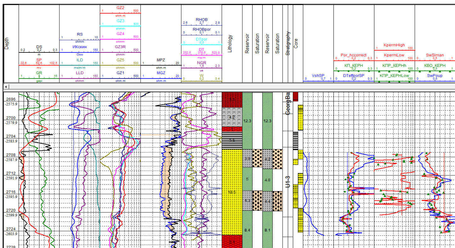
Рис. 4.10. Планшет с коррелированными кривыми скважины № 204
