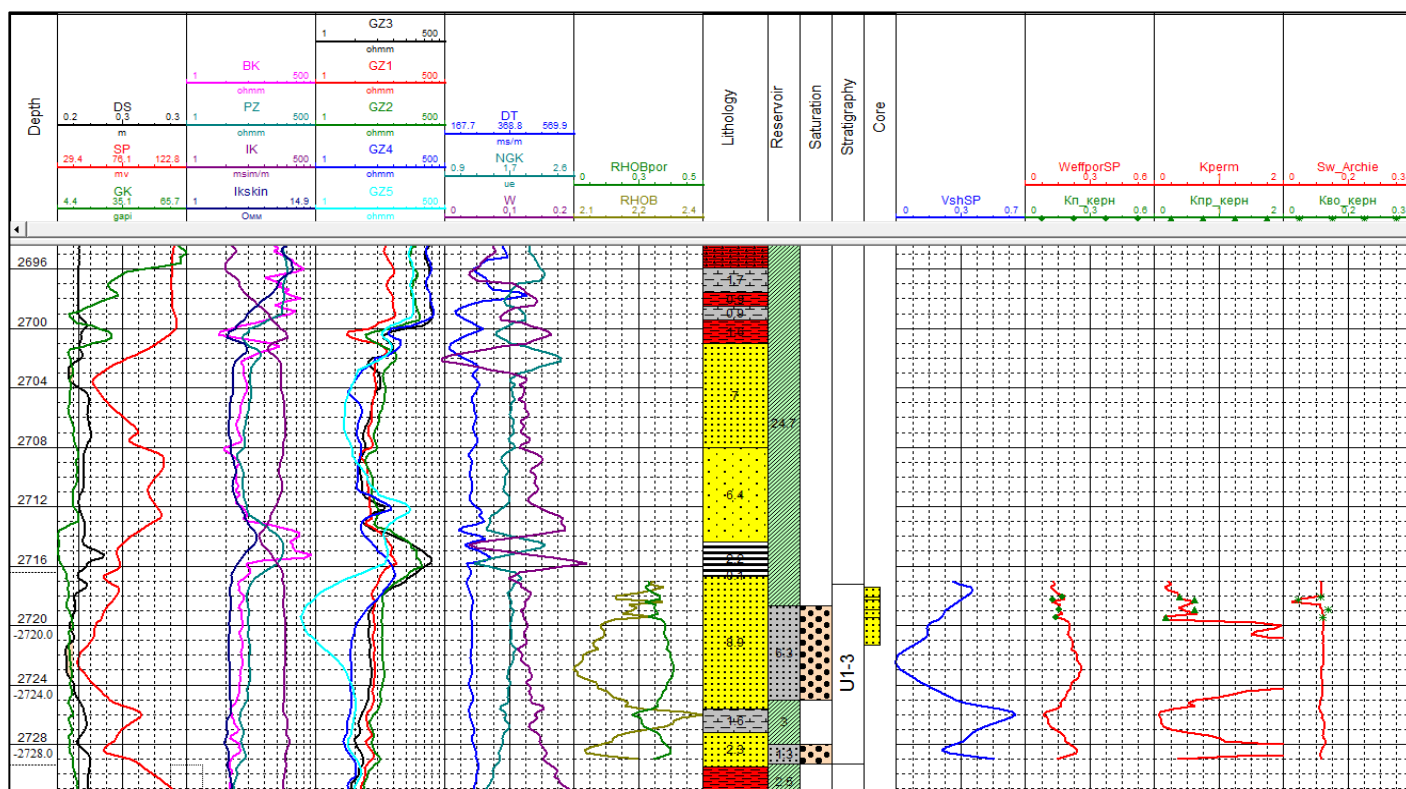
Рис. 4.12. Планшет с коррелированными кривыми скважины № 212
