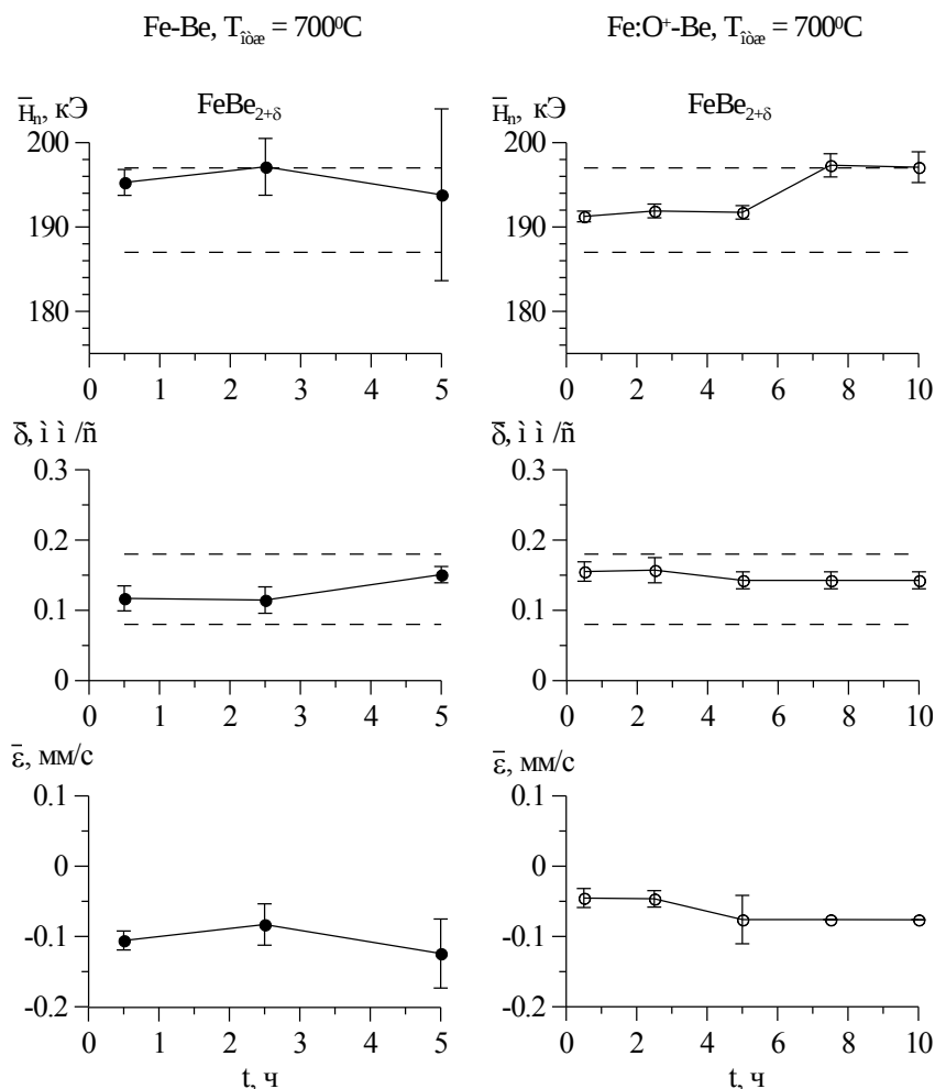
Рисунок 5 – Средние значения эффективных магнитных полей \bar{H}_n , сдвигов \delta и квадрупольных смещений \epsilon мессбауэровских спектров для фазы FeBe 2+δ в слоистых системах Fe-B- 57 Fe и Fe:O + -Be- 57 Fe в зависимости от времени изотермического отжига t_{отж}
