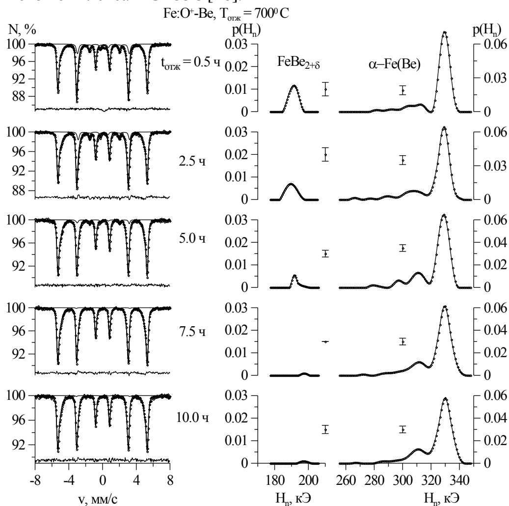
Рисунок 3 – Мессбауэровские спектры и результат восстановления функций распределения p(H_n) эффективных магнитных полей H_n на ядрах ^{57}\text{Fe} в системе \text{Fe:O}^+\text{-Be-}^{57}\text{Fe} ( t_{\text{отж}}=0,5 ч до 10,0 ч) после последовательных изотермических отжигов при температуре T_{\text{отж}} = 700^\circ\text{C}
