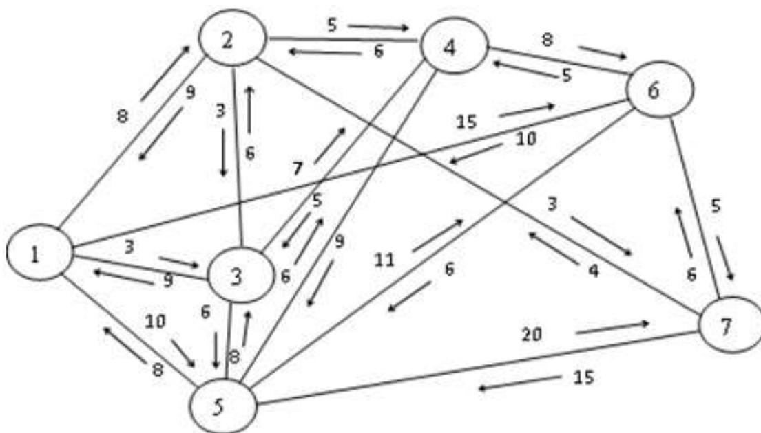
Рис. 1 Линейная сеть автомобильных дорог с циклом: 1 – исходный сборный эвакуационный пункт, 2-6 – промежуточные пункты, 7 – приемный эвакуационный пункт.
