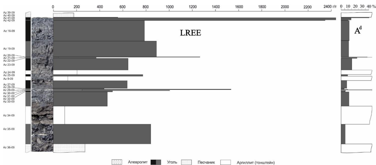
Рисунок 5. Распределение суммы легких редкоземельных элементов в разрезе пласта.
