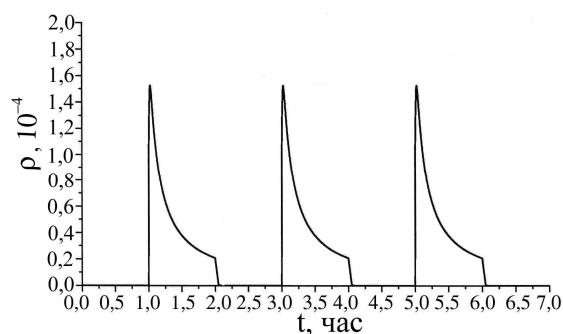
Рис. 20. Изменение реактивности для n(t) по регламенту б
