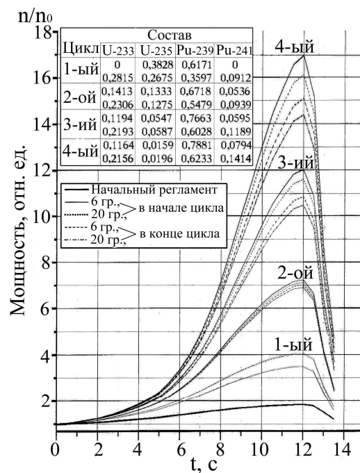
Рис. 15. Изменение мощности в различных циклах выгорания
