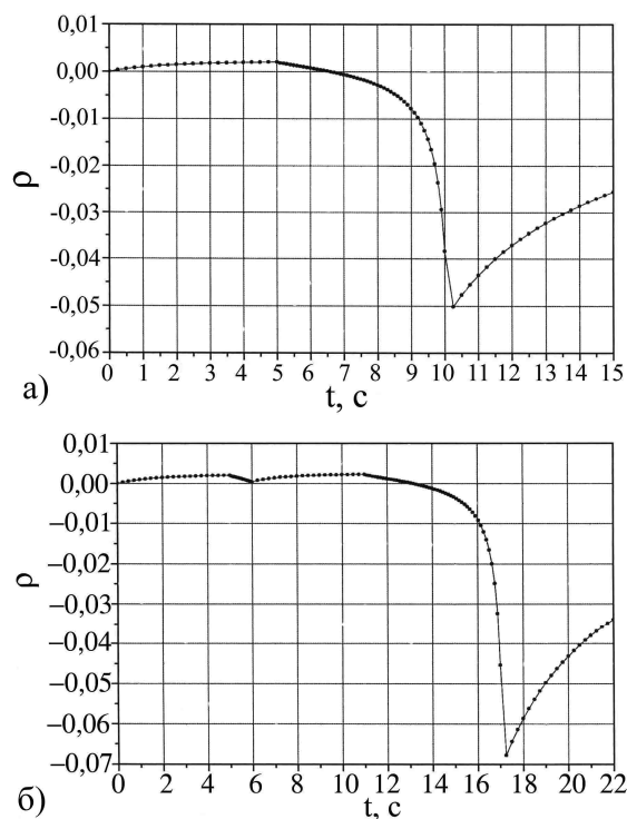
Рис. 19. Изменение реактивности для n(t) по регламенту: а) 1; б) 2
