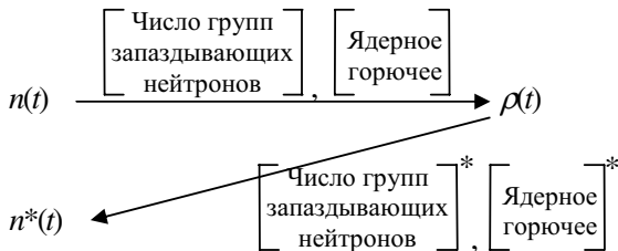
Рис. 8. Обратная задача
