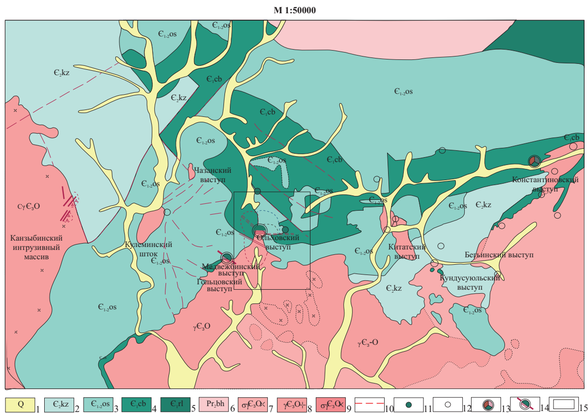
Рис. 1. Геологическая карта северной части Ольховско-Чибизежского рудного района: 1) современные аллювиальные отложения, глины сугленки, пески; 2) кизирская свита. Риолиты, туфы, линзы известняков; 3) осиновская свита. Аргиллиты, алевролиты, туфы кислого и среднего состава, туфопесчаники; 4) чибизежская свита. Известняки, прослои и линзы аргиллитов и туфов; 5) колпинская свита. Песчаники, алевролиты, сланцы; 6) кварц-хлоритовые, кварц-эпидот-хлоритовые сланцы; 7) диориты; 8) граниты; 9) гранодиориты, плагииграниты; 10) тектонические нарушения; 11) коренные месторождения золота, сульфидные залежи; 12) рудопроявления золота; 13) месторождения золота, жилы кварц-карбонатные с сульфидами и гематитом; 14) месторождения золота, жилы кварц-сульфидного состава; 15) контур участка работ
