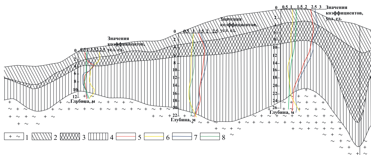
Рис. 2. Схематический геологический разрез. Зоны: 1) дресвяно-щебенистая; 2) охристо-каолиновая; 3) нижняя часть охристо-каолиновой зоны с повышенными содержаниями золота; 4) монтмориллонит-гидрослюдистая. Коэффициенты: 5) окисления; 6) выщелачивания; 7) ферритизации; 8) аллитизации
