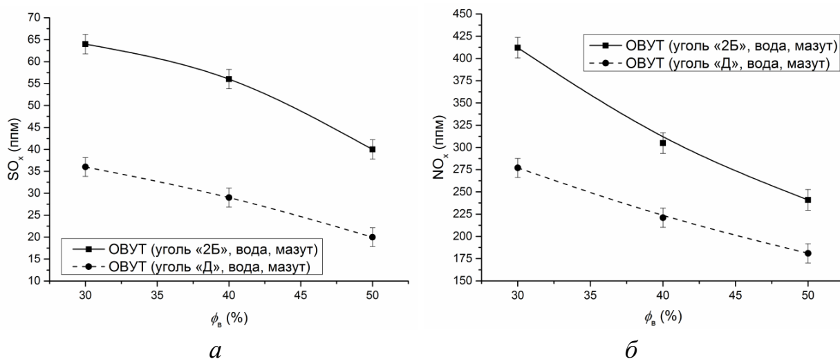
Рисунок 3.6. Экспериментальные зависимости [136] концентраций SO x (а), NO x (б) от содержания воды (φ в ) в суспензиях ОВУТ на основе мазута (10 %) при температуре в камере сгорания 800 °С
