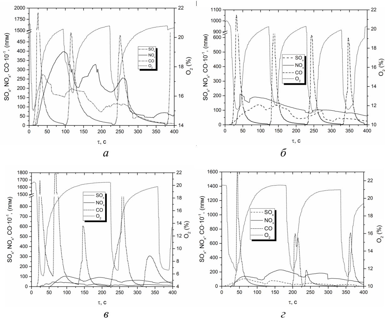
Рисунок 3.1. Тренды основных газообразных выбросов сжигания [135] угольной пыли ( а ), ВУТ ( б ) и ОВУТ на основе мазута ( в ) и турбинного масла ( г ) при температуре в камере сгорания 800 °С
