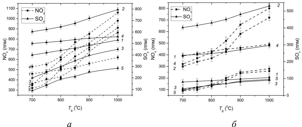
Рисунок 3.20. Зависимости [243] максимальных концентраций SO x и NO x от температуры при сжигании кеков (а) и ОВУТ (кек в исходном железном состоянии и 10 % мазута) (б): 1 – фильтр-кек «Т»; 2 – фильтр-кек «К»; 3 – фильтр-кек «Г»; 4 – фильтр-кек «СС»; 5 – фильтр-кек «Д»
