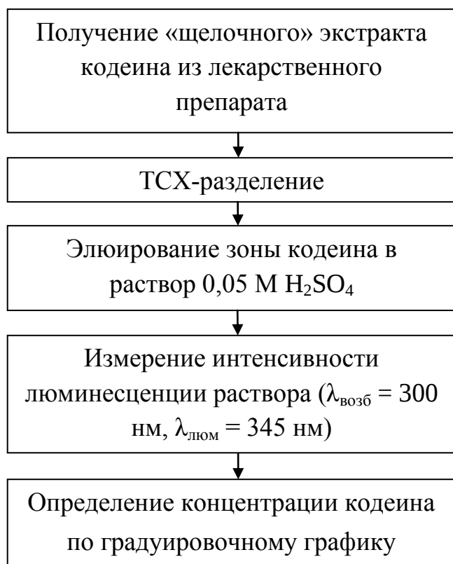
Рисунок 10. Схема методики люминесцентного определения кодеина в лекарственных препаратах
