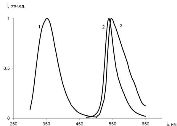
Рисунок 5. Нормированные спектры флуоресценции водных растворов кодеина (1), эозина (2), экстракта ионного ассоциата кодеина с эозином в толуоле (3)
