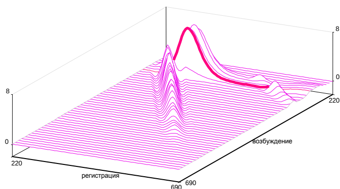
Рисунок 2. Трехмерный спектр люминесценции раствора кодеина ( C_{\text{код}} = 1 \text{ г/дм}^3 ; 0,05 \text{ М H}_2\text{SO}_4 )
