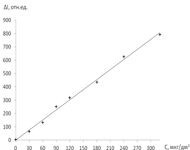
Рисунок 17. Градуировочный график экстракционно-флуориметрического определения кодеина в моче
