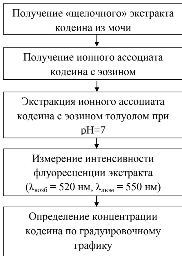
Рисунок 16. Схема методики экстракционно-флуориметрического определения кодеина в моче человека
