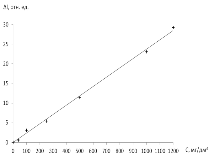
Рисунок 11. Градуировочный график люминесцентного определения кодеина в лекарственных препаратах
