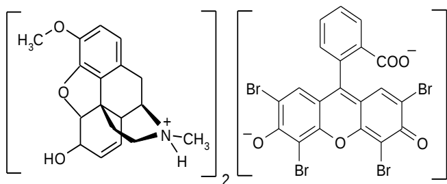
Рисунок 4. Ионный ассоциат кодеина с эозином
