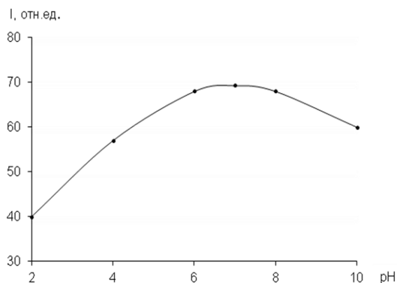
Рисунок 6. Зависимость интенсивности флуоресценции экстракта ионного ассоциата кодеина с эозином в толуоле от pH водного раствора ( C_{\text{код}} = C_{\text{эоз}} = 0,03 \text{ мг/дм}^3 , \lambda_{\text{в}} = 520 \text{ нм} )
