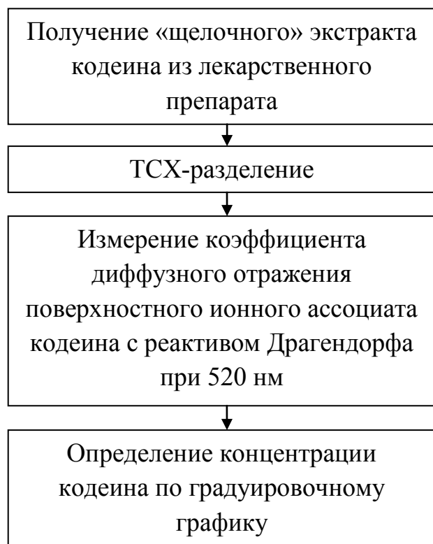
Рисунок 12. Схема методики определения кодеина в лекарственных препаратах методом спектрометрии диффузного отражения
