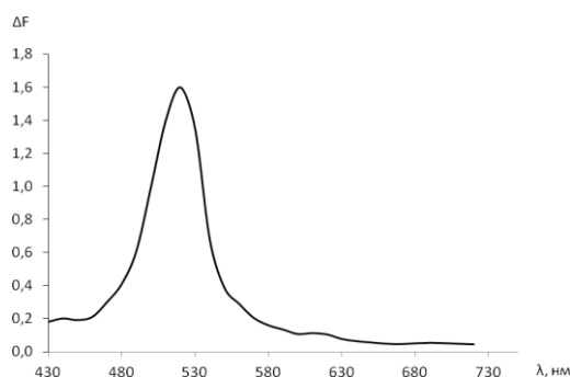
Рисунок 9. Спектр диффузного отражения поверхностного ионного ассоциата кодеина с реактивом Драгендорфа
