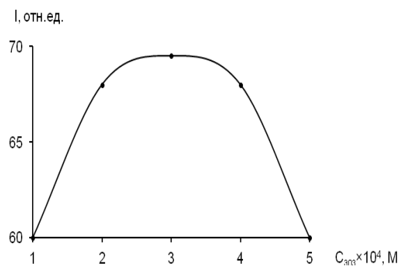
Рисунок 7. Зависимость интенсивности флуоресценции экстракта ионного ассоциата кодеина от концентрации эозина в водном растворе ( C_{\text{код}} = 1 \cdot 10^{-4} \text{ M} , \text{pH} = 7 , \lambda_{\text{в}} = 520 \text{ нм} )
