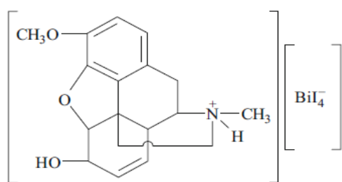
Рисунок 8. Ионный ассоциат кодеина с реактивом Драгендорфа
