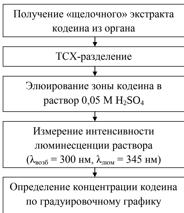
Рисунок 14. Схема методики люминесцентного определения кодеина в органах человека
