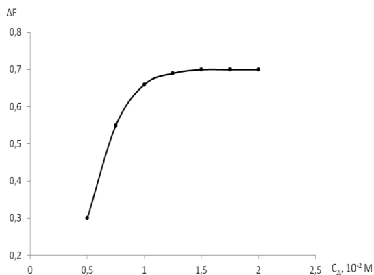
Рисунок 10. Зависимость \Delta F от концентрации реактива Драгендорфа ( C_d ), C_{\text{код}}=250 \text{ мг/дм}^3
