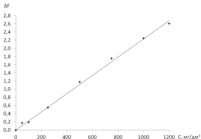
Рисунок 13. Градуировочный график определения кодеина в лекарственных препаратах методом спектрометрии диффузного отражения
