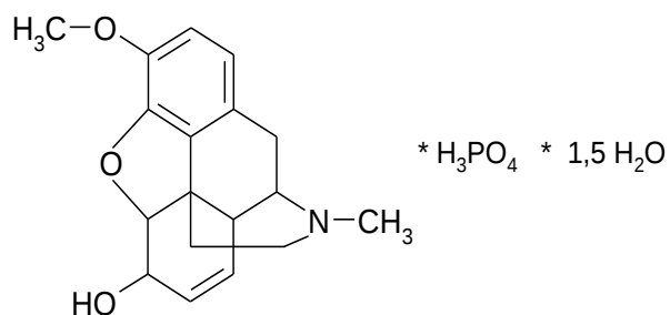
Рисунок 1. Структурная формула кодеина фосфата
