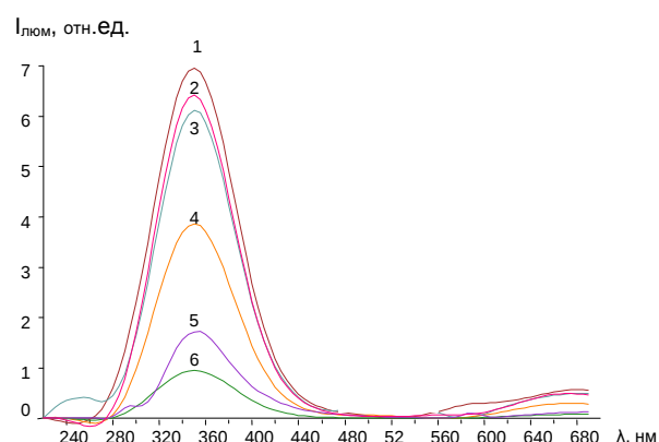
Рисунок 3. Спектры люминесценции растворов кодеина при различных pH среды ( \lambda_{\text{возб}} = 300 \text{ нм} , C_{\text{код}} = 1 \text{ г/дм}^3 ): pH =1 (1), 4 (2), 7 (3), 9 (4), 11 (5) и 13 (6)
