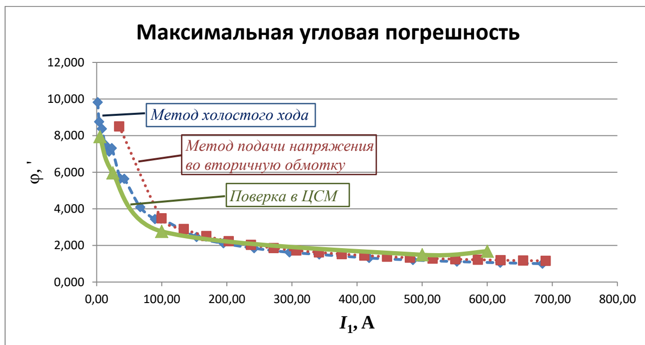
Рисунок 4 – Зависимости максимальной угловой погрешности от первичного тока, определенной косвенными методами и при поверке в ЦСМ.
