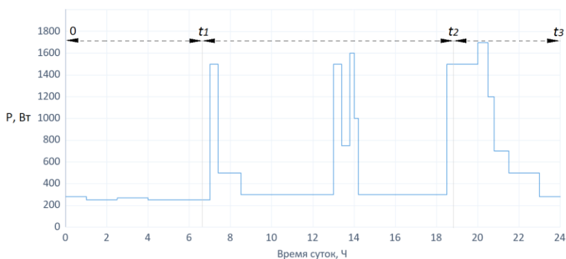
Рисунок 1 – Типовой график энергопотребления
