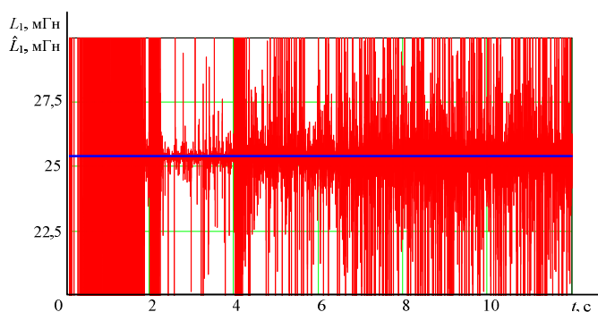
Рис. 4. Переходный процесс оценки эквивалентной индуктивности обмотки статора \hat{L}_1 , имеющий ярко выраженную дисперсионную составляющую
