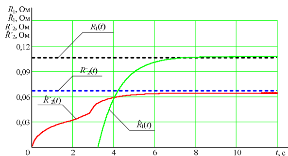
Рис. 1. Переходные процессы оценок активного сопротивления обмотки статора \hat{R}_1 и приведенного к статору активного сопротивления обмотки ротора \hat{R}_2
