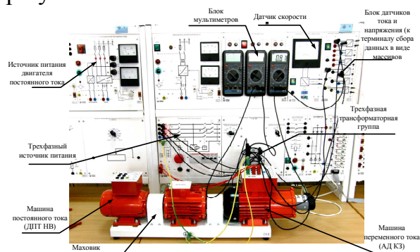
Рис. 7. Внешний вид экспериментальной установки для проверки работоспособности алгебраических методов идентификации асинхронных электродвигателей, питающихся напрямую от сети
