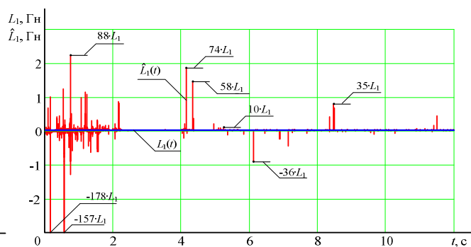
Рис. 5. Переходный процесс оценки эквивалентной индуктивности обмотки статора \hat{L}_1 , имеющий ярко выраженную импульсную составляющую
