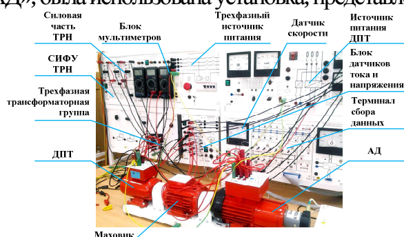
Рис. 8. Внешний вид экспериментальной установки ТРН-АД
