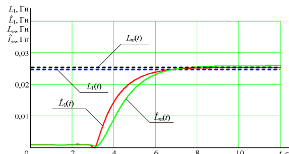
Рис. 2. Переходные процессы оценок эквивалентной индуктивности обмотки статора \hat{L}_1 и результирующей индуктивности, обусловленная магнитным потоком в воздушном зазоре асинхронного электродвигателя \hat{L}_m
