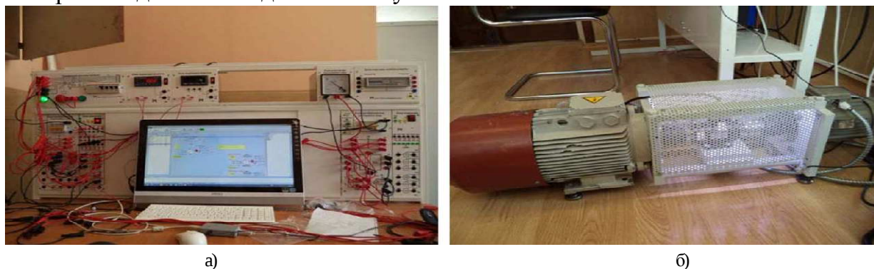
Рис. 9. Внешний вид экспериментальной установки для проверки работоспособности алгебраических методов идентификации асинхронных электродвигателей в составе электропривода, включенного по схеме ПЧ-АД
