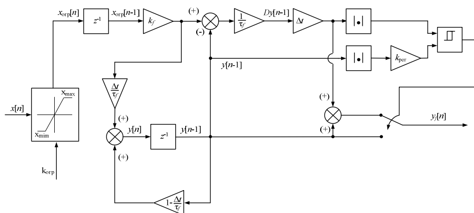
Рис. 6. Структурная схема разработанного нелинейного прогнозирующего фильтра
