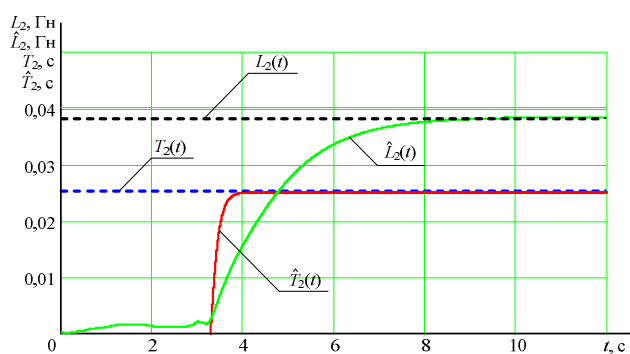
Рис. 3. Переходные процессы оценок постоянной времени ротора \hat{T}_2 и приведенной к статору эквивалентной индуктивности обмотки ротора \hat{L}_2
