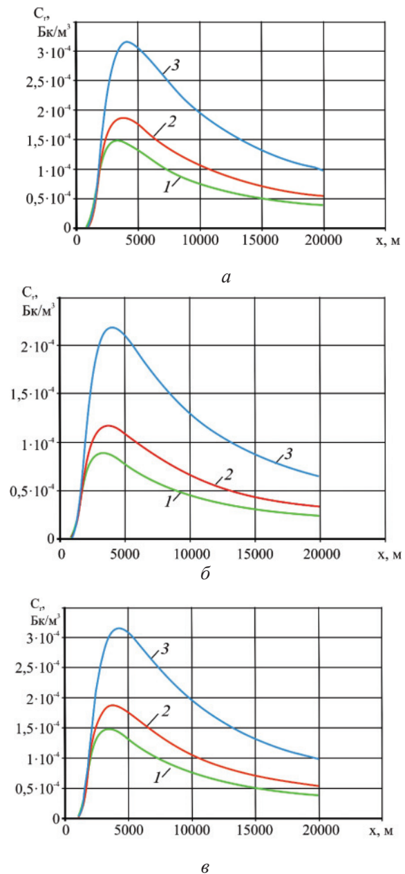
Рис. 6. Распределение концентрации йода (а), аэрозолей (б) и РБГ (в) в приземном слое (категория Е, z_0=40 см; t=+20^\circ\text{C} ; t_0=15^\circ\text{C} ; w_0=10 м/с) при разных скоростях ветра u : 1) 6; 2) 4; 3) 2 м/с
