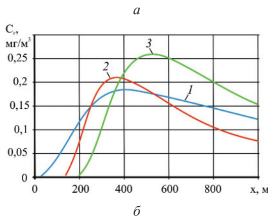
Рис. 3. Распределение приземной концентрации \text{SO}_2 , \text{NO}_2 вдоль оси факела при опасной скорости ветра, соответствующее благоприятным (а) и неблагоприятным (б) метеорологическим условиям: 2 и 3 – расчет по методике Пасквила ( z_0=10 и 1 см); 1 – расчет по методике MPP-2017
