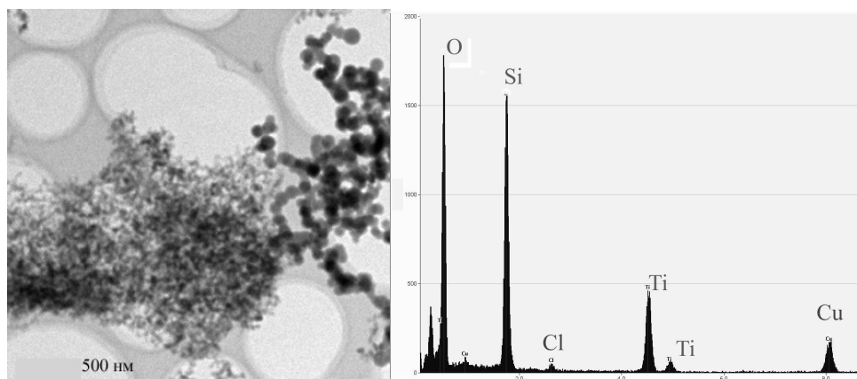
Рис. 5. Фотография, полученная на ПЭМ, и EDX-спектр порошка x \cdot \text{TiO}_2 + y \cdot \text{SiO}_2 . Большие и малые наночастицы вместе
