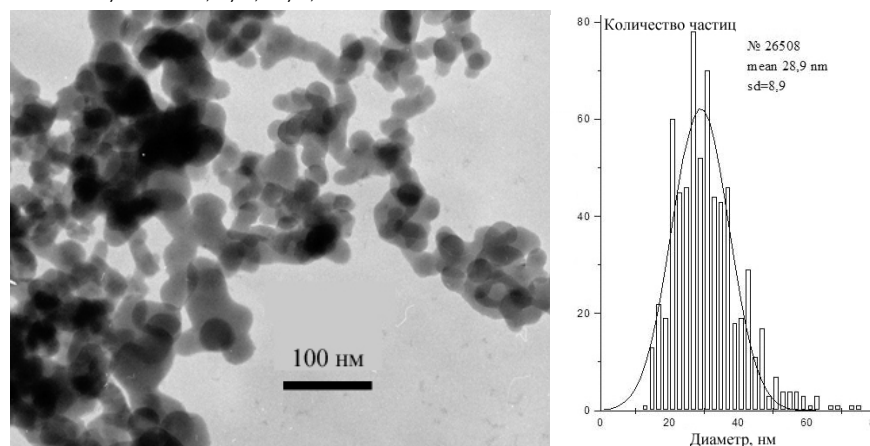
Рис. 4. Фотография и гистограмма распределения размеров порошка xTiO_2+ySiO_2 . Среднечисловой размер 29 нм
