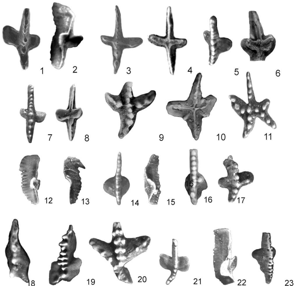
Рис. 9. Виды лохковских конодонтов из разреза Миндигулово. Все фигуры имеют увеличение \times 32 . 1, 2 – Lanea otoalpha Murphy & Valenzuela-Rios, 1999: 1 – вид сверху, Pa-элемент, 2 – вид снизу, Pa-элемент, обр. M-28; 3, 4 – Ancyrodelloides transitans (Bischoff & Sannemann), 1958: 3 – вид сверху, Pa-элемент, 4 – вид снизу, Pa-элемент, обр. M-448; 5, 6 – Lanea eleanorae (Lane & Ormiston, 1979): 5 – вид сверху, Pa-элемент, 6 – вид снизу, Pa-элемент, обр. M-25; 7, 8 – Lanea eoeleanorae Murphy & Valenzuela-Rios, 1999: 7 – вид сверху, Pa-элемент, 8 – вид снизу, Pa-элемент, обр. M-28; 9, 10 – Ancyrodelloides trigonicus Bischoff & Sannemann, 1958: 9 – вид сверху, Pa-элемент, 10 – вид снизу, Pa-элемент, обр. M-268; 11 – Ancyrodelloides kutscheri Bischoff & Sannemann, 1958, вид сверху, Pa-элемент, обр. M-278; 12 – Pandorinellina optima (Moskalenko, 1966), вид сбоку, Pa-элемент, обр. 17-7; 13 – Pandorinellina exigua philipi (Klapper, 1969), вид сбоку, Pa-элемент, обр. M-49; 14, 15 – Masaraella pandora morphotype alpha (Murphy, Matti & Wallizer, 1981): 14 – вид сверху, Pa-элемент, 15 – вид сбоку, Pa-элемент, обр. M-268; 16, 17 – Masaraella pandora morphotype beta (Murphy, Matti & Wallizer, 1981): 16 – вид сверху, Pa-элемент, обр. M-36, 17 – вид сверху, Pa-элемент, обр. M-452; 18 – Pelekysgnathus cf. guardarramensis Valenzuela-Rios, 1994, вид сверху, обр. M-49; 19 – Icriodus cf. angustoides alcoleae Carls, 1969, вид сверху, I-элемент, обр. M-49; 20 – Pedavis gilberti Valenzuela-Rios, 1990, вид сверху, I-элемент, обр. 02441; 21, 22 – Masaraella pandora morphotype zeta (Murphy, Matti & Wallizer, 1981): 21 – вид сверху, Pa-элемент, обр. 02441, 22 – вид сбоку, Pa-элемент, обр. 02441; 23 – Eognathodus cf. irregularis Druce, 1971, вид сверху, Pa-элемент, обр. 02456
