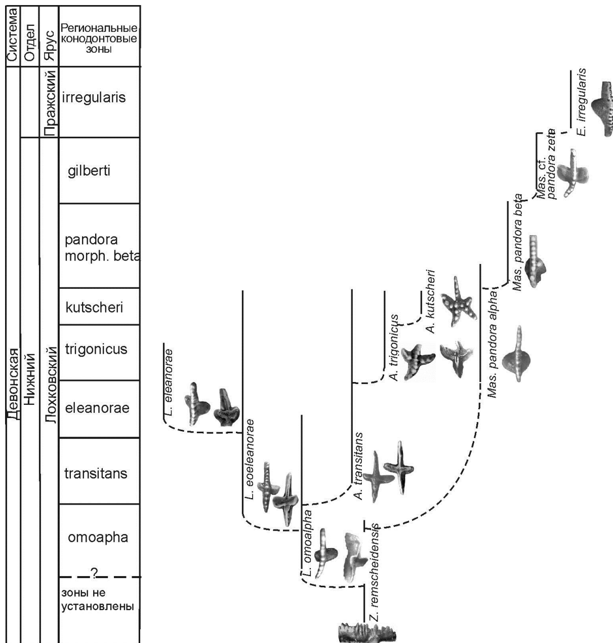
Рис. 10. Филогенетическая последовательность таксонов Ancyrodelloides , Lanea , Masaraella (в соответствии со схемами эволюции [24, 29, 32]). Пример сокращений – на рис. 6. Рисунок заимствован из [28] с изменениями
