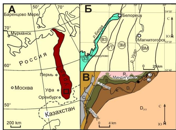
Рис. 1. А) Местоположение района исследований; Б) схема структурно-формационного районирования палеозойских отложений Южного Урала (фрагмент Лесенда, 1998). Структурно-формационные зоны отмечены заглавными буквами в кружках: 33 – Западно-Зилаирская; B3 – Восточно-Зилаирская; UP – Уралтауская; 3М – Западно-Магнитогорская; В) фрагмент геологической карты по материалам В.А. Шефера и др., 2001 (рукоп.) и Ю.Г. Князева и др., 2008 (рукоп.) с расположением изученных обнажений № 2 и 3 в разрезе Миндигулово. Заимствовано из [5] Fig. 1. А) Location maps of the studied area; Б) scheme of structural zoning of the Urals (fragment from Legend 1998). Structural zones are marked with capital letters in circles: 33 – West-Zilair Zone, B3 – East-Zilair Zone, UP – Uraltau Zone, 3M – West-Magnitogorsk Zone; В) geological map fragment of the area under study according to V.A. Shefer et al. 2001 (unpublished) and Yu.G. Knyazev et al. 2008 (unpublished) with marked location of outcrops no. 2 and 3 in Mindigulovo section. Adopted from [5]
