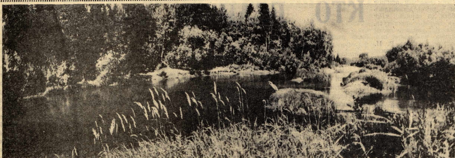
ОСЕНЬ. Фотоэтиюд В. Аникина.
