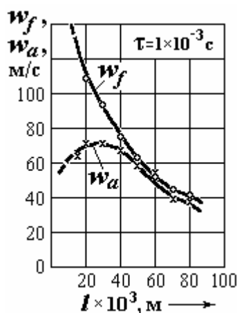
Рис. 6. Изменение скорости движения топлива и воздуха по длине струи
