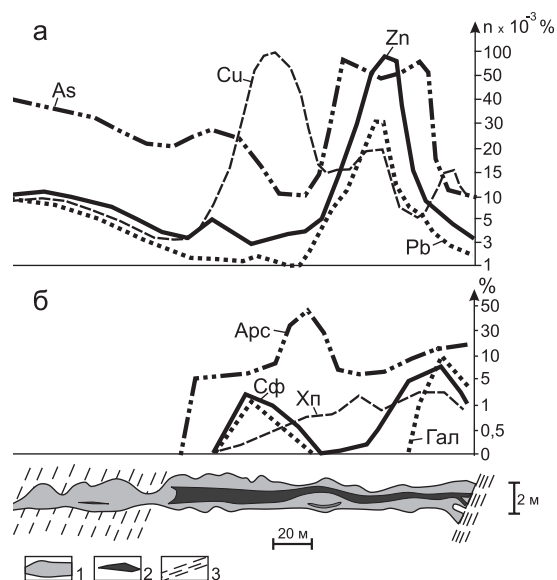
Рис. 2. Вынос халькофильных элементов из внутренней зоны березитов на участках сопряженного отложения сульфидов в жиле (Центральное месторождение, жила Тысячная, горизонт +336 м): 1) околожильные березиты; 2) кварцево-сульфидные линзы; 3) зоны повышенной проницаемости; а) распределение элементов в березитах; б) концентрация сульфидов в жиле: арсенопирита (Арс), халькопирита (Хп), сфалерита (Сф), галенита (Гал)
