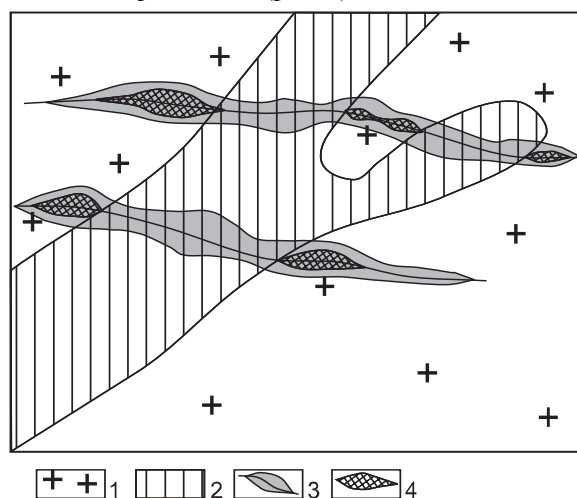
Рис. 1. Схема пространственных взаимоотношений площадных предрудных метасоматитов и золотоносных кварцево-сульфидных жил: 1) слабо измененные гранитоиды; 2) зоны повышенной проницаемости с площадными предрудными метасоматитами; 3) рудовмещающие трещины с березитами; 4) кварцево-сульфидные линзы
