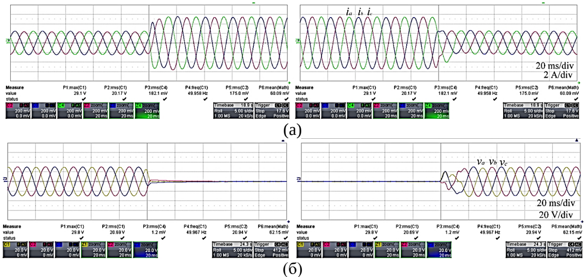
Рис 14. (а)Ток и(б) напряжение нагрузки до трёхфазного КЗ, в течение трёхфазного КЗ и после.
