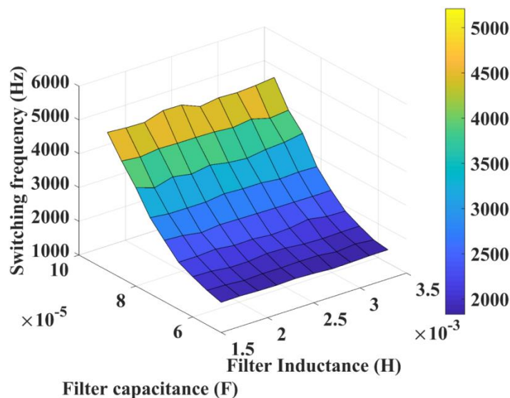
Рис. 9. Изменение f_s УПМ при вариациях параметров LC-фильтра.
