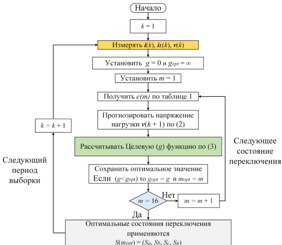
Рис. 3. Блок-схема алгоритма прогнозирующего управления АИН
