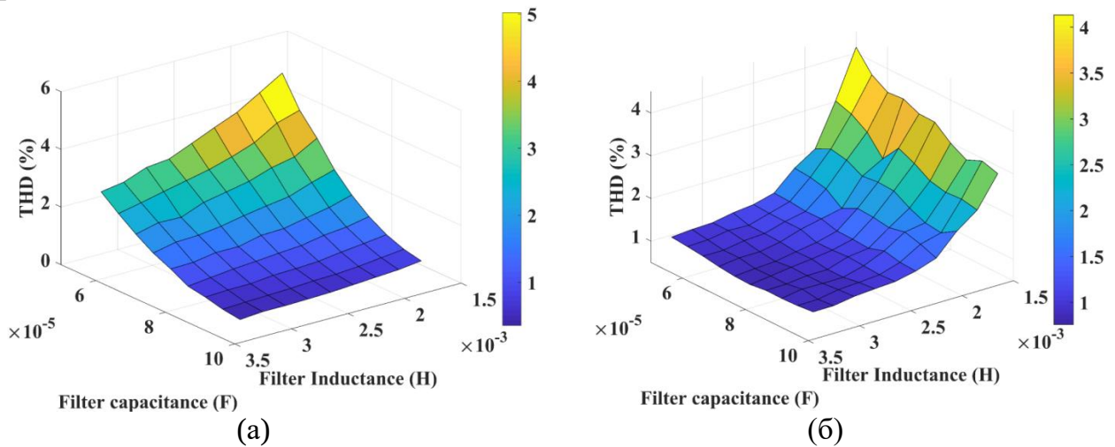
Рис. 8. Изменение %КНИ при вариациях параметров LC-фильтра (а)УПМ (б) ПИД.
