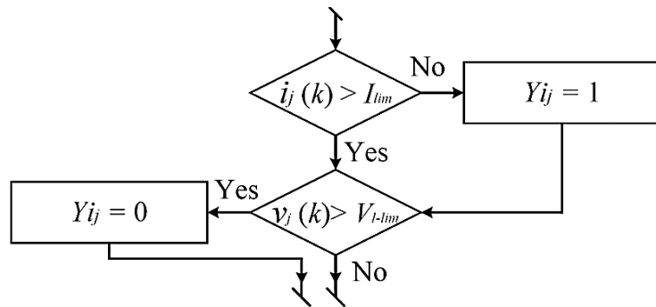
Рис. 10. Часть алгоритма обнаружения КЗ в предлагаемом алгоритме УПМ
