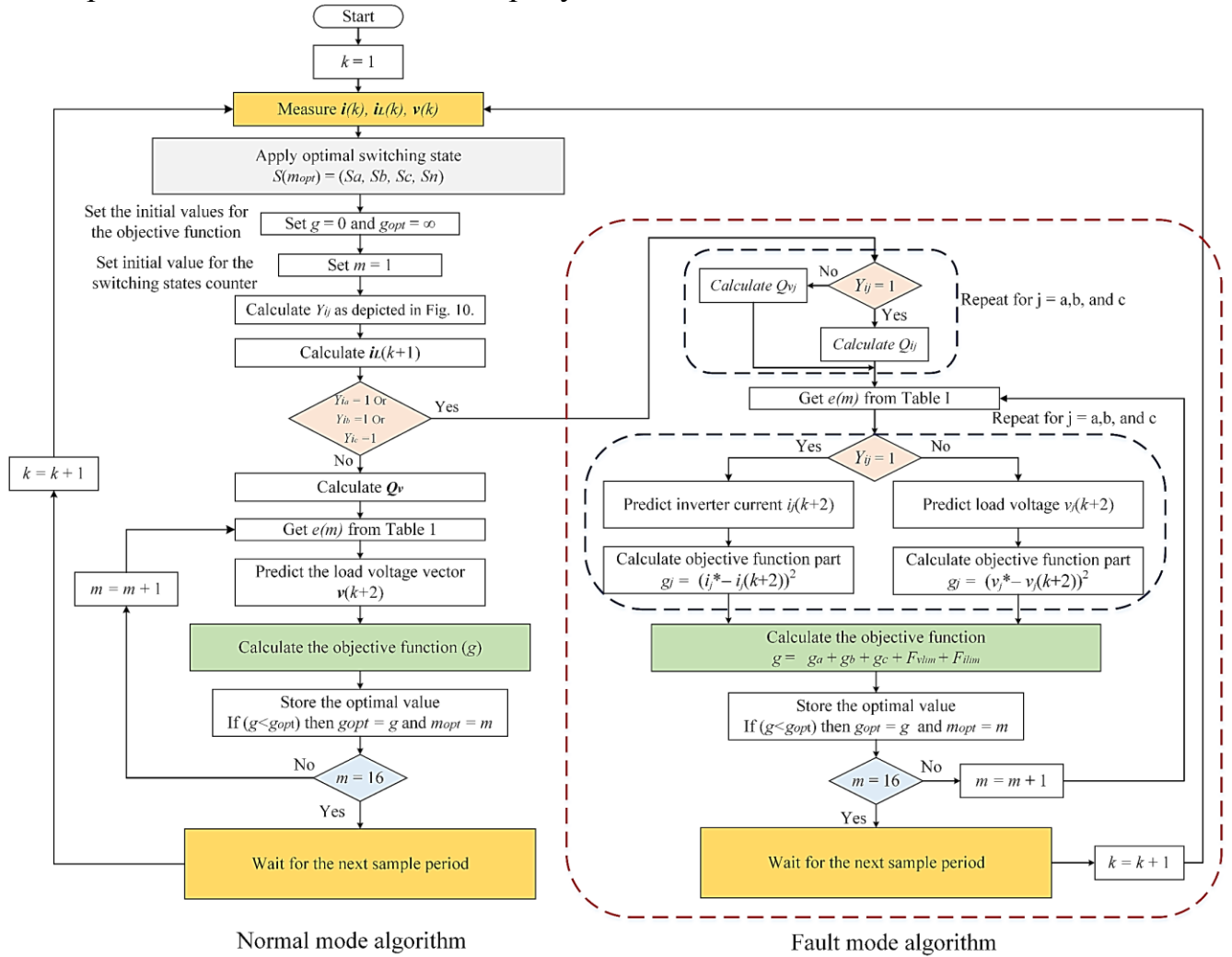
Рис. 11. Блок-схема оптимизированного предложенного алгоритма УПМ
