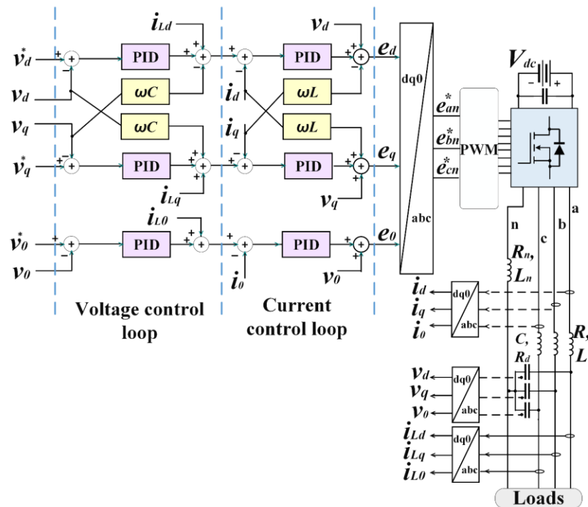
Рис. 4. Топологическая схема СЭС при управлении АИН на основе ПИД-регуляторов
