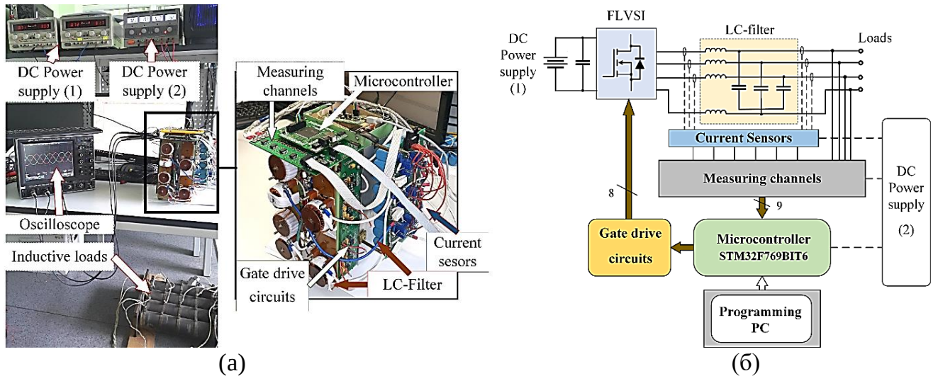
Рис. 12. Экспериментальная установка (а) и ее функциональная схема (б)
