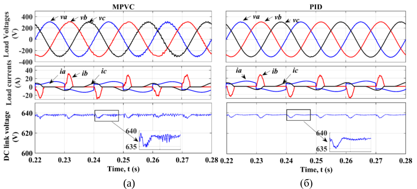
Рис. 6. Результаты моделирования СЭС (несбалансированные нелинейные нагрузки) при (а) УПМ и (б) ПИД
