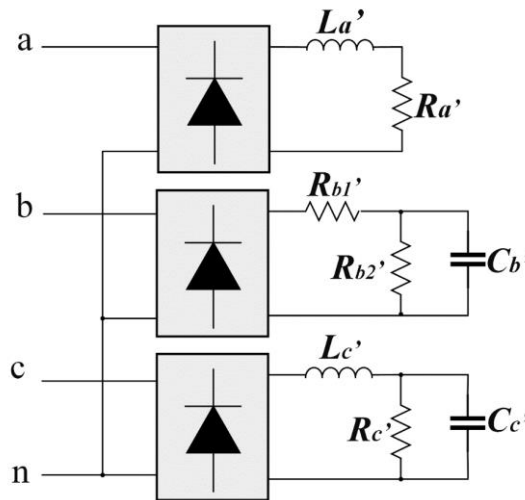
Рис. 5. Топология однофазных нагрузок СЭС, используемых в моделировании.
