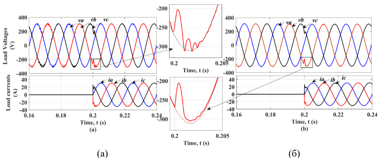
Рис. 7. Напряжения и токи нагрузки СЭС при динамическом режиме для (а) УПМ и (б) ПИД
