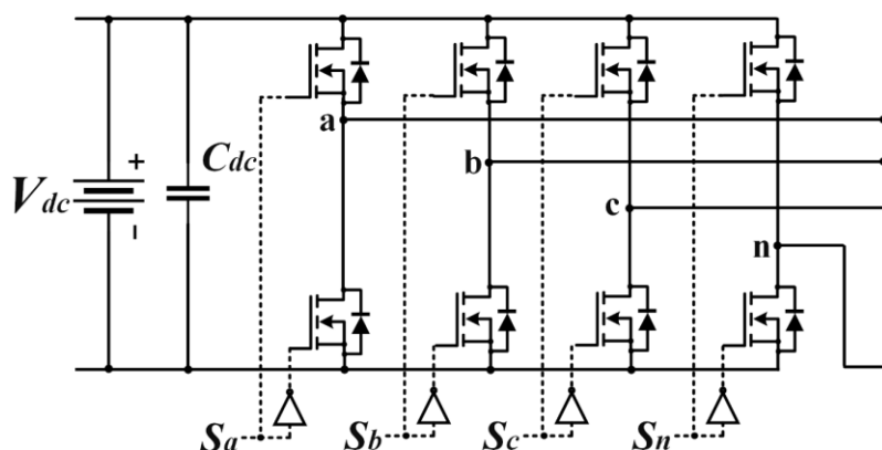
Рис. 1. Топология трёхфазного АИН с четвёртой стойкой
