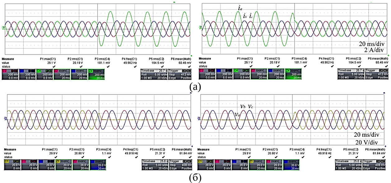
Рис 13. (а)Ток и(б) напряжение нагрузки до однофазного КЗ, в течение однофазного КЗ и после.
