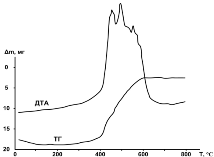
Рис. 7 Дериватограмма НП Al: m = 50 мг, скорость нагрева – 10^\circ/\text{мин} , атмосфера – воздух, тигель – платина.
