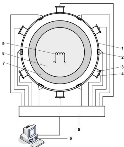
Рис. 1. Схема устройства для синхронного измерения температуры и яркости свечения горящих материалов. 1 – кольцо, выполненное из оптически прозрачного кварца; 2 – термопара, выполненная из сплавов ВР5/ВР20; 3 – цилиндр, выполненный из непрозрачного материала; 4 – фоторезистор ФСК-1; 5 – согласующее устройство; 6 – компьютер; 7 – подложка; 8 – навеска конической формы; 9 – нихромовая спираль
