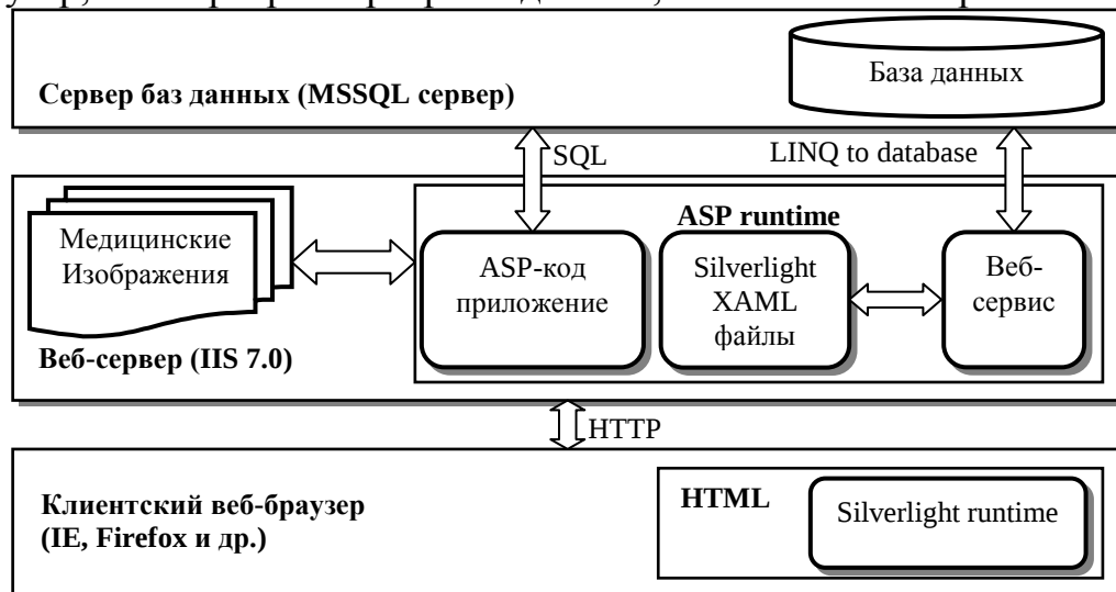
Рис. 7. Трехзвенная архитектура системы
