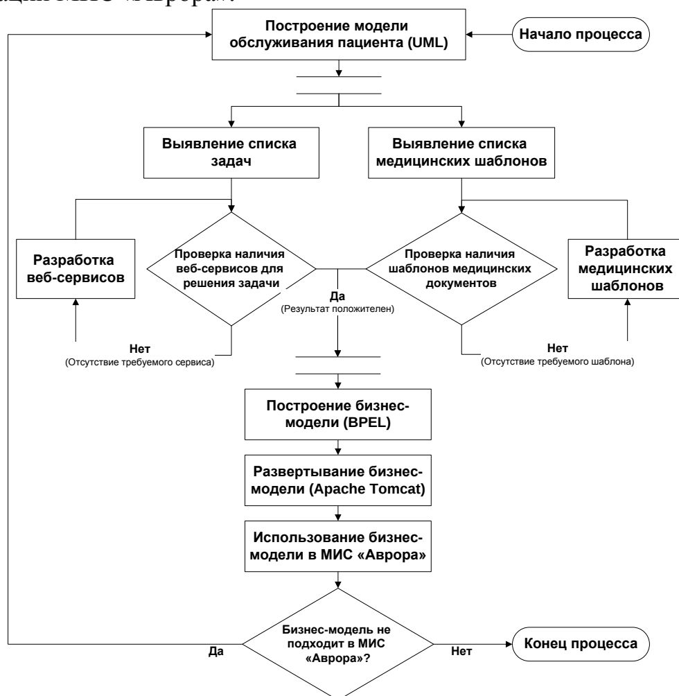
Рис. 1. Алгоритм для задачи динамической конфигурации МИС
