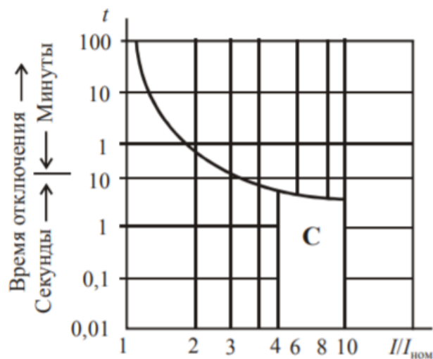
Рисунок 1.3 – ВТХ для типа С [4]
