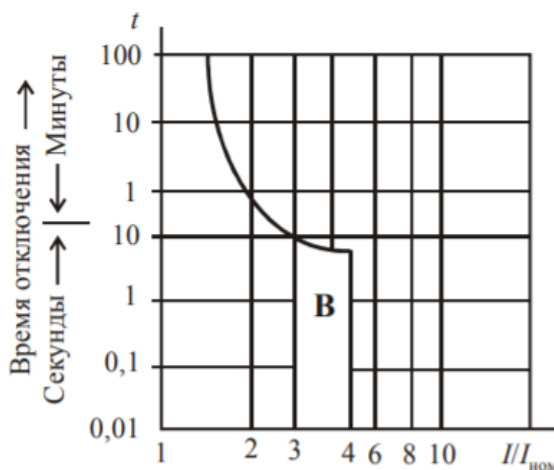
Рисунок 1.2 – ВТХ для типа В [4]
