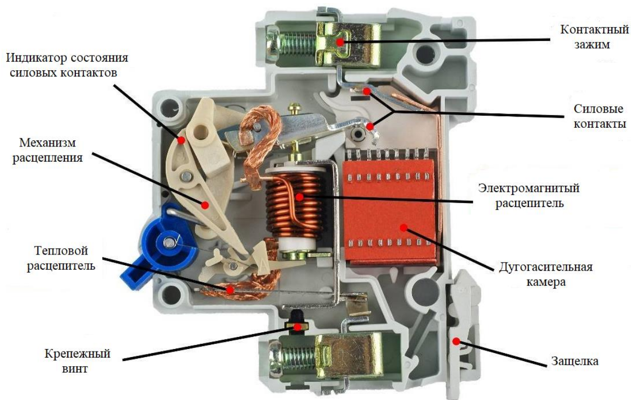
Рисунок 1.1 – Устройство автоматического выключателя [1]
