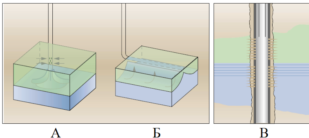
Рисунок 3 – Механизм обводнения пластовой водой: а) – конусообразование; б) – языкообразование; в) – подъём ВНК к интервалу перфорации [5]
