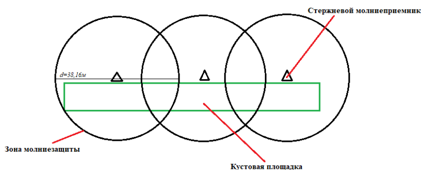
Рисунок 36 – Схема расстановки молниеотводов на кустовой площадке месторождения «Х»
