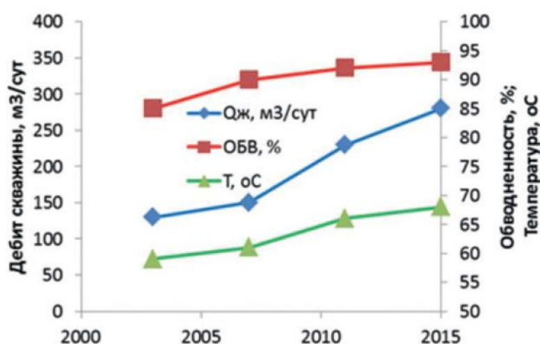
Рисунок 10 – Характерные изменения во времени дебита, обводнённости и температуры на устье добывающей скважины одного из месторождений Западной Сибири [11]
