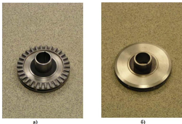
Рисунок 32 – Импеллеры ступеней ЭЦН: а) центробежно-вихревой; б) - центробежный
