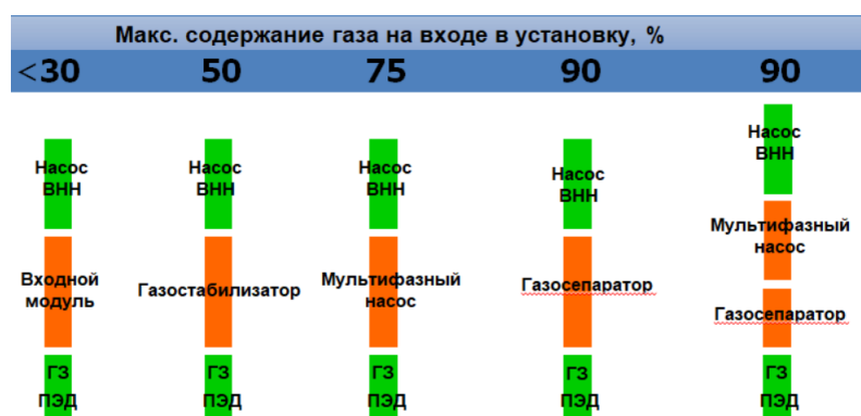
Рисунок 33 – Комплектации установок для работы с высоким газовым фактором
