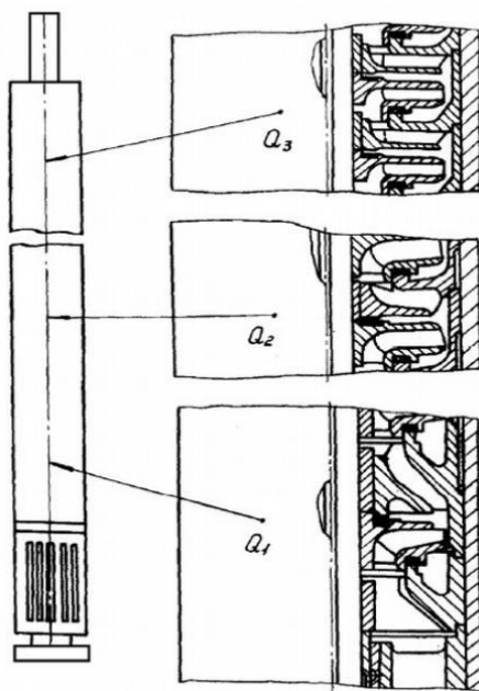
Рисунок 31 – Схема «конического» насоса
