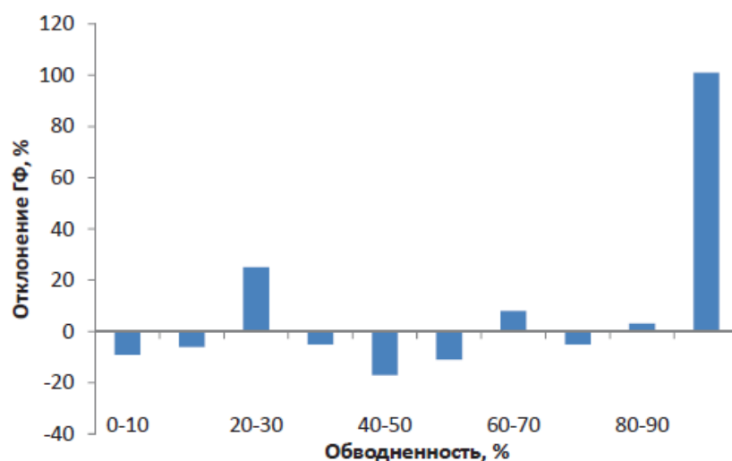
Рисунок 6 – Отклонение значений газового фактора от проектных в зависимости от степени обводнённости одного из нефтедобывающих предприятий Западной Сибири [11]
