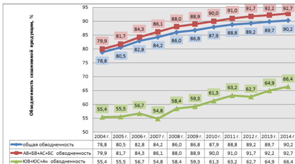
Рисунок 8 – Динамика обводнённости добывающих скважин ООО «ЛУКОЙЛ – западная Сибирь» за период 2004 – 2014гг. [10]
