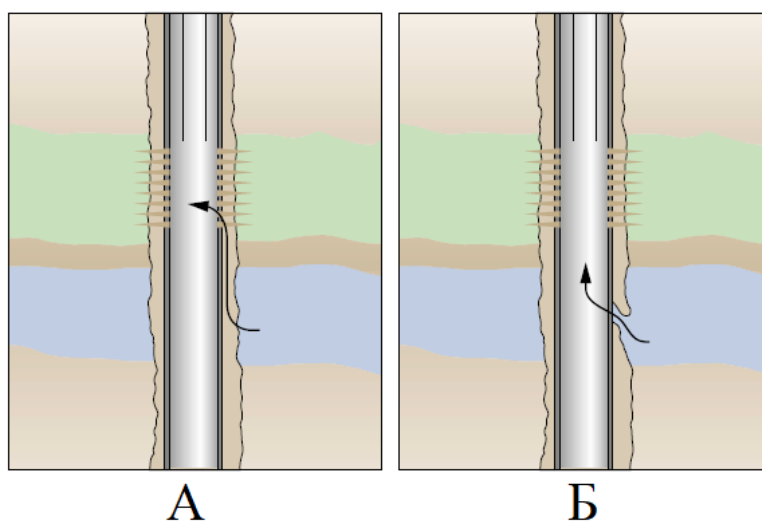
Рисунок 4 – Механизм обводнения в результате технических проблем: а) – заколонный переток; б) – негерметичность эксплуатационной колонны [5]
