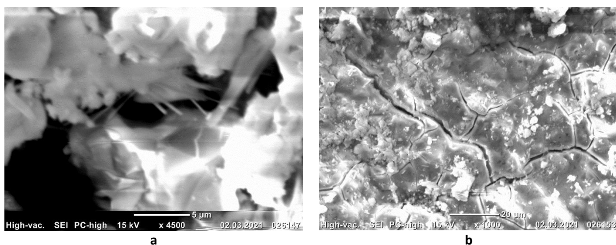
Рисунок 7 – Электронный микроснимок поровой структуры композита с 30 % (a) и 40 % (b) карбида кремния
