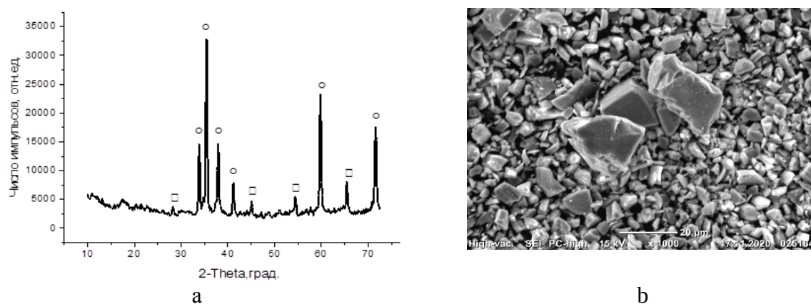
Рисунок 3 – Рентгенограмма (а) и электронный микроснимок (b) смеси арсенида галлия и карбида кремния
