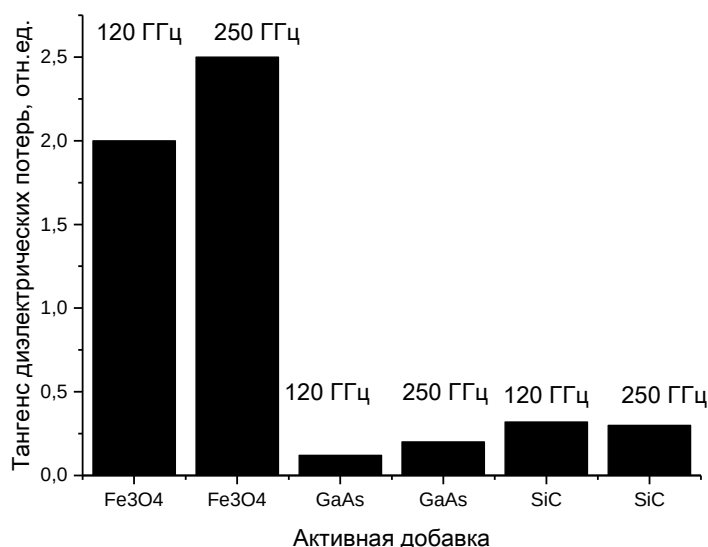
Рисунок 11 – Тангенс диэлектрических потерь образцов с добавками на частотах 120 и 250 ГГц
