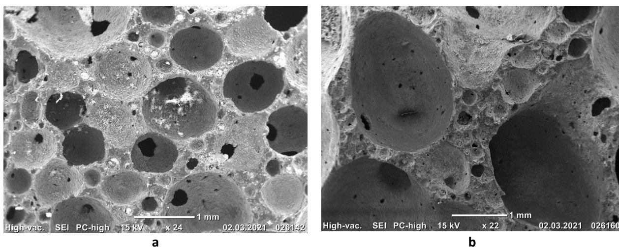
Рисунок 8 – Электронный микроснимок поровой структуры композита с 10 % (a) и 40 % (b) карбида кремния
