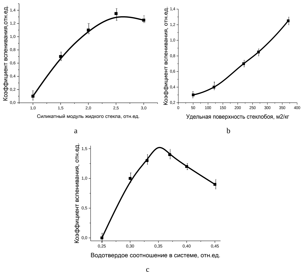
Рисунок 5 – Зависимость коэффициента вспенивания композиции от модуля жидкого стекла (а), удельной поверхности стеклопорошка (б), водотвердого соотношения фаз (с)
