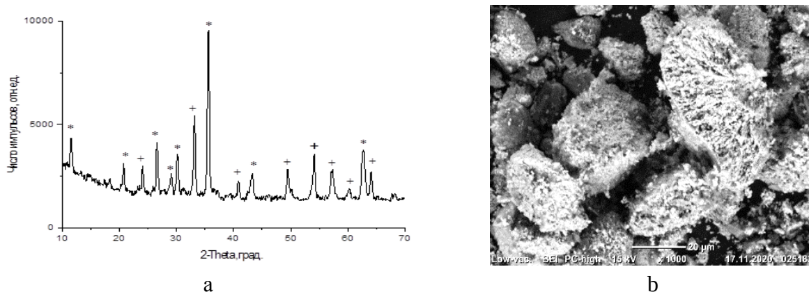
Рисунок 4 – Рентгенограмма (а) и электронный микроснимок (b) \text{Fe}_3\text{O}_4 (пиритные огарки)
