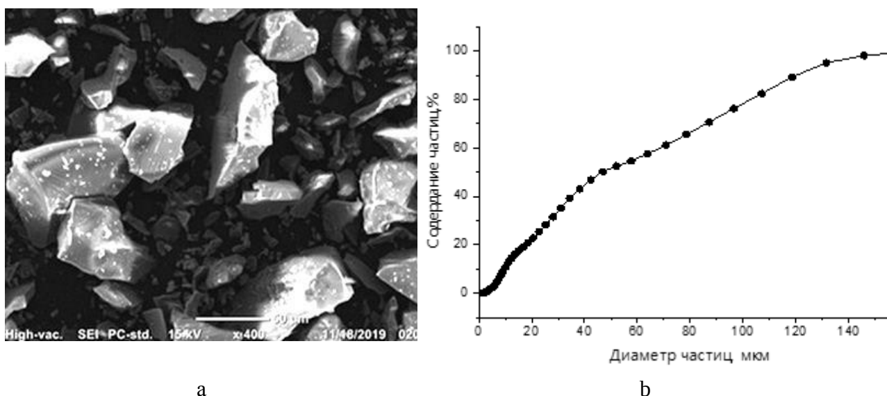
Рисунок 1 – Электронный микроснимок частиц стекла (а) и распределение частиц по размерам (б) после измельчения в планетарной мельнице
