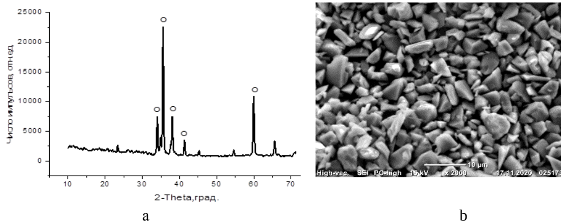
Рисунок 2 – Рентгенограмма (а) и электронный микроснимок (b) карбида кремния
