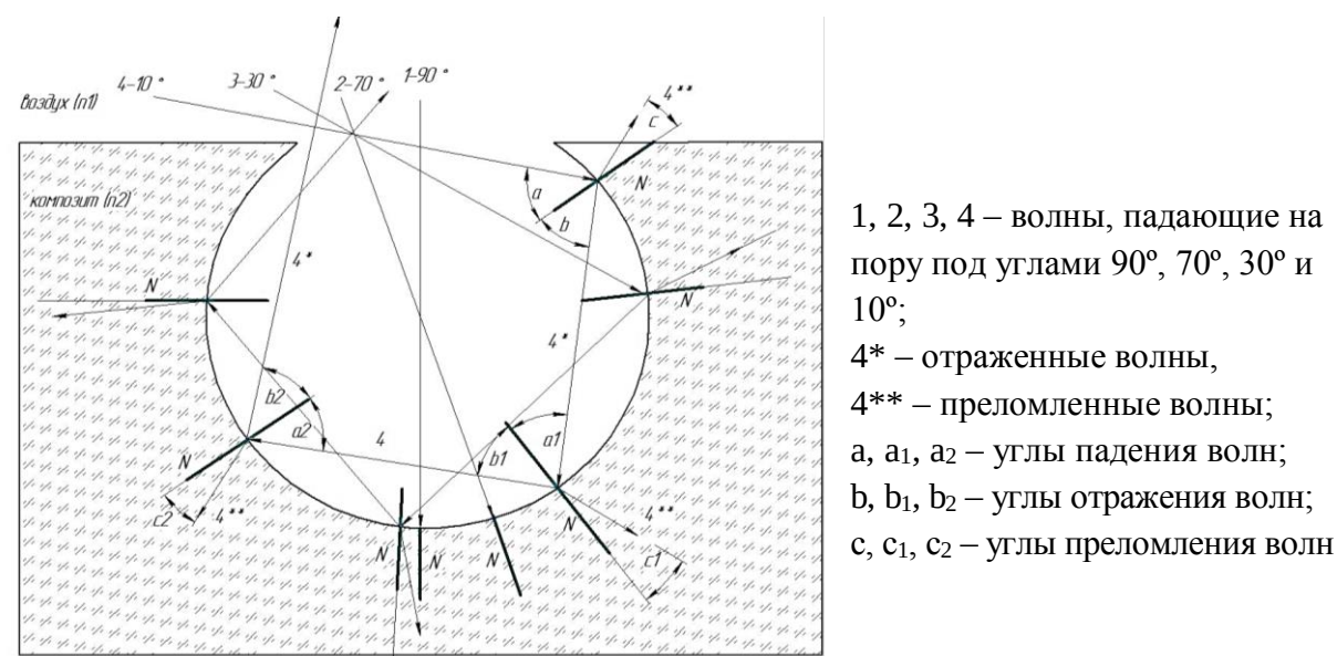
Рисунок 9 – Схема траекторий электромагнитных волн, падающих на поверхностную пору композита, вскрытую на 20 %: n_1 и n_2 – показатель преломления среды и композита; N – нормаль к отражающей поверхности раздела фаз
