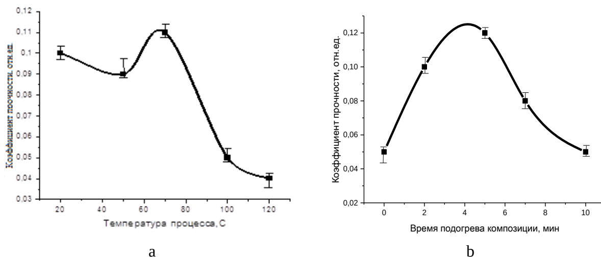
Рисунок 6 – Зависимость коэффициента прочности от: а – температуры процесса вспенивания; б – времени предварительного подогрева наполнителя и матрицы
