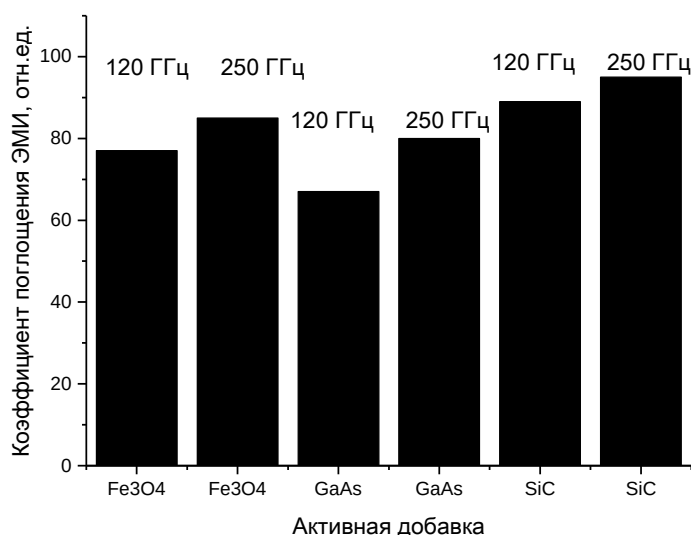
Рисунок 12 – Коэффициент поглощения электромагнитной волны для образцов с активными добавками на частотах 120 и 250 ГГц
