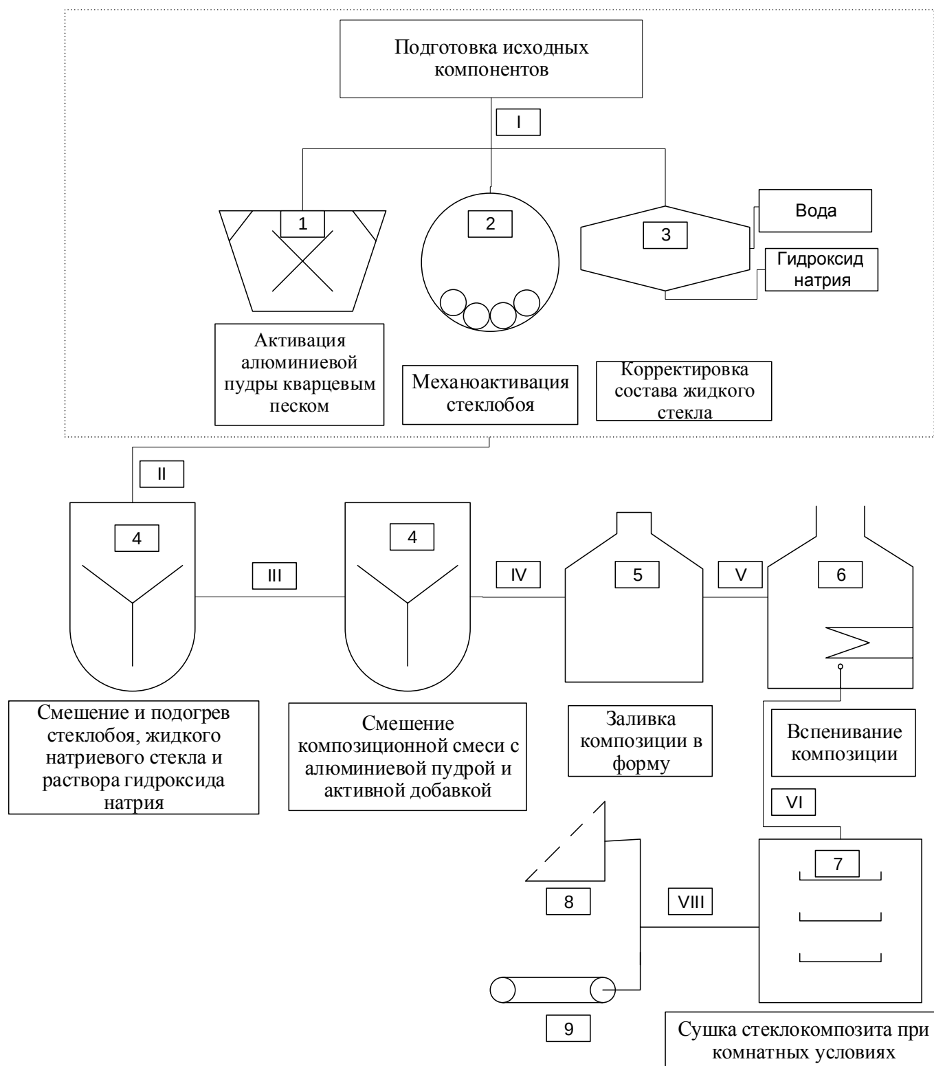
Рисунок 13– Технологическая схема получения пористого стеклокомпозита: 1 – шаровая мельница, 2 – активатор, 3 – емкость с мешалкой, 4 – смеситель лопастной с функцией подогрева, 5 – форма для вспенивания, 6 – сушильный шкаф, 7 – стеллаж, 8 – станок дисковой или струнной резки, 9 – линия упаковки и транспортировки
