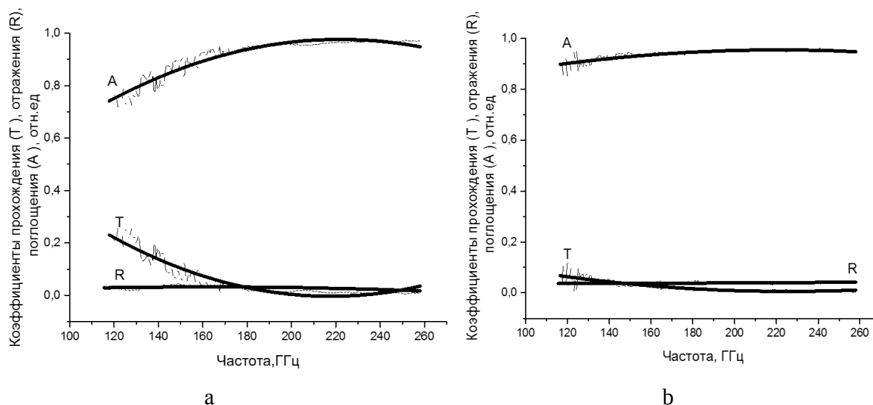
Рисунок 10 – Зависимость коэффициентов прохождения (Т), отражения (R), поглощения (А) от частоты для стеклокомпозита со средним размером пор: а – 1,2 мм; б – 3,1 мм
