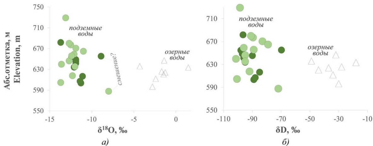
Рис. 4. Соотношение изотопного состава кислорода (а) и водорода (б) воды с гипсометрическим положением водных объектов района Торейских озёр (условные обозначения – на рис. 2)
