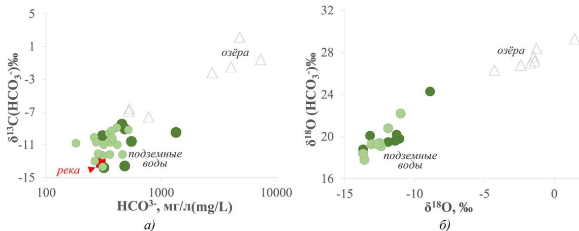
Рис. 5. Зависимость \delta^{13}\text{C}(\text{HCO}_3^-) природных вод района Торейских озёр от содержания \text{HCO}_3^- (а) и \delta^{18}\text{O}(\text{HCO}_3^-) от \delta^{18}\text{O} (б) (условные обозначения – на рис. 2)
