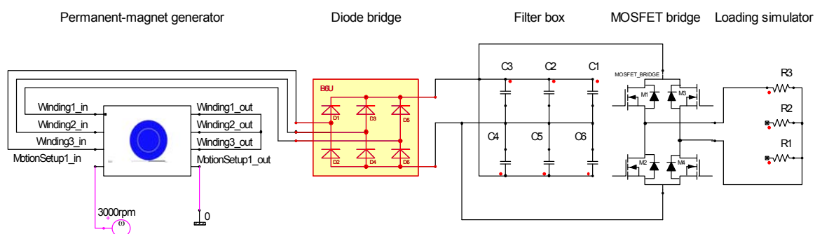
Рис. 6. Комплексная математическая модель скважинной аппаратуры телеметрической системы
