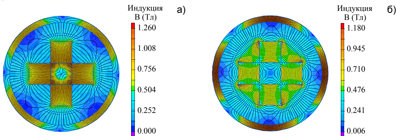
Рис. 4. Распределение магнитного поля при аксиальном (а) и тангенциальном (б) намагничивании (внешний диаметр магнитопровода статора 54 мм)
