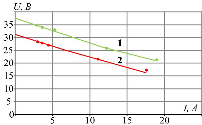
Рис. 11. Внешние характеристики макетов скважинного генератора.
