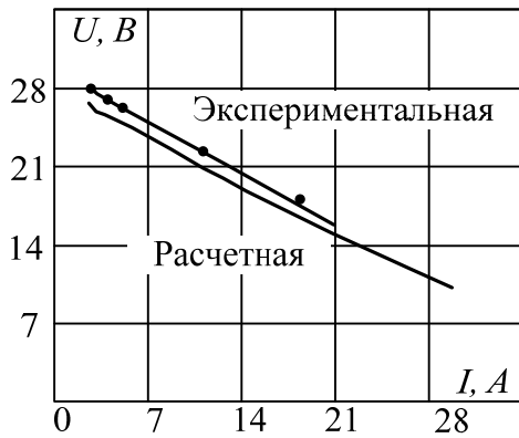
Рис. 10. Внешние характеристики скважинного генератора
