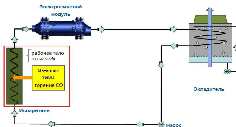
Рисунок.2. Паровой цикл установки
