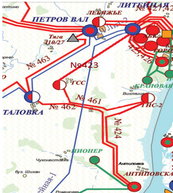
Рисунок 2. Предложенная схема.
