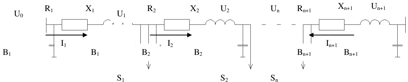
Рисунок 2. Схема замещения.
