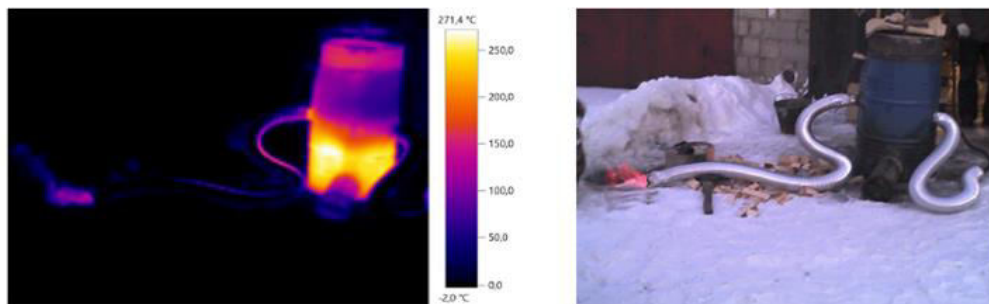
Рисунок.3 Газогенератор. Термограммы
