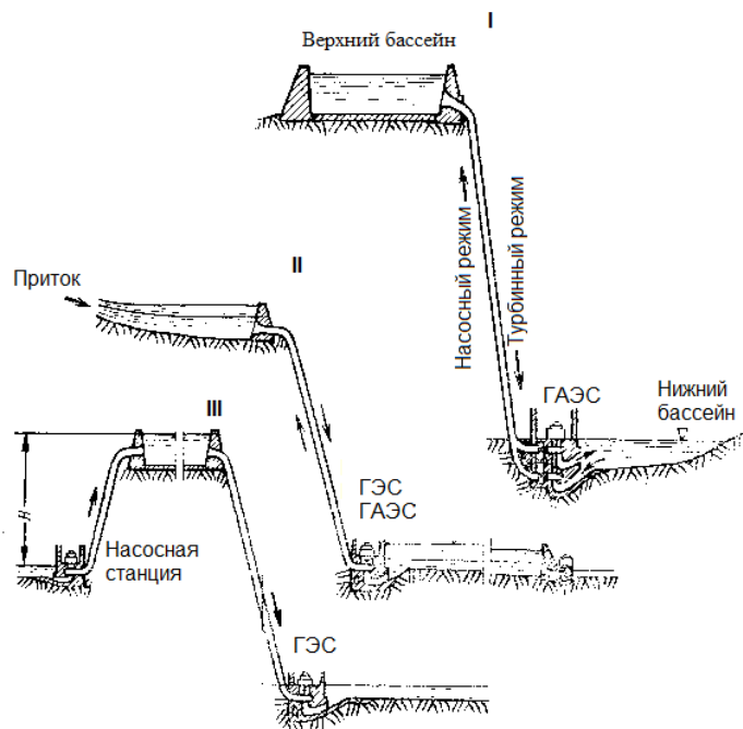
Рисунок 2. Схемы ГАЭС
