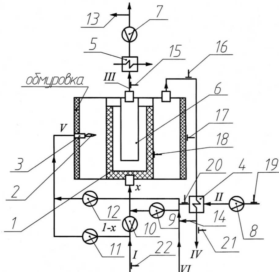
Рисунок 1. Принципиальная схема эндотермического генератора с газовым обогревом: 1 – реторта с катализатором; 2 – камера сгорания; 3 – газовые горелки; 4 – трубчатый пальчиковый рекуператор двойной циркуляции; 5 – охладитель; 6 – рекуператор; 7 – ротаметр расхода продуктов конверсии; 8 – ротаметр расхода общего воздуха; 9 – шайба расхода пара на конверсию; 10 – ротаметр расхода метана на конверсию; 11 – ротаметр расхода метана на обогрев реторты; 12 – ротаметр расхода воздуха на обогрев реторты; 13 – отбор продуктов конверсии на анализ; 14 – отбор продуктов сгорания на анализ; 15 – датчик контроля температуры продуктов конверсии; 16 – датчик контроля температуры отходящих дымовых газов на
