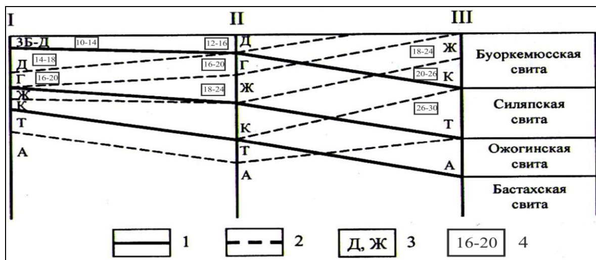
Рис. 3. Схематический разрез изменения метаморфизма и метаноносности углей Зырянского бассейна по угленосным районам: 1– граница между свитами, 2 – граница зон метаморфизма, 3 – марки углей. Угленосные районы: I – Индигиро-Селенняхский, II – Мятисский, III – Зыряно-Селяпский районы: 1– граница между свитами, 2 – граница зон метаморфизма, 3 – марки углей, 4 – прогнозная метаноносность угольных пластов, м 3 /т.с.б.м
