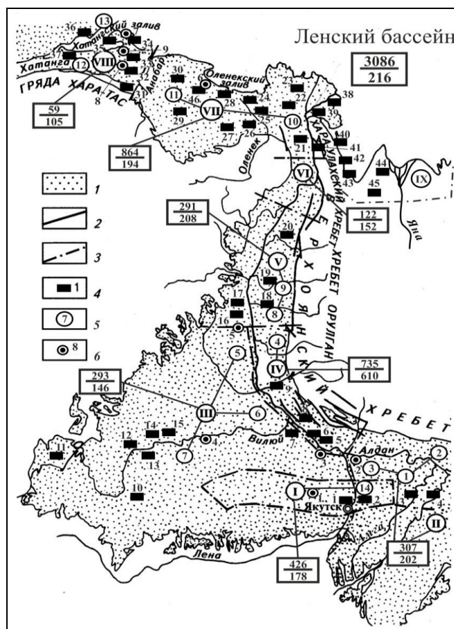
Рис. 5. Схема распределения перспективных для извлечения ресурсов метана в Ленском бассейне: 1 – продуктивные юрско-меловые угленосные отложения, 2 – основные разломы, 3 – границы угленосных районов (римские цифры в кружках): I – Якутско-Кангаласский; II – Нижне-Алданский; III – Вилюйский; IV – Сангарский; V – Жиганский; VI – Булунский; VII – Оленекский; VIII – Анабаро-Хатангский. IX – Лаптевско-Янский бассейн. 4 – основные угольные месторождения: Ленский бассейн: 1 – Кангаласское, 2 – Хапчагайское; 3 – Харбалахское (Амгинское), 4 – Джебарики-Хайское, 5 – Белогорское; 6 – Сангарское, 7 – Тас-Тумусское, 8 – Люнкюбейское, 9 – Леписское, 10 – Кемпендйское, 11 – Пятачковое, 12 – Октябрьское, 13 – Нижне-Нюрбинское, 14 – Чапандинское, 15 – Кировское, 16 – Уаттахское, 17 – Жиганское, 18 – Бегиджянское, 19 – Соболахское, 20 – Джарджанское, 21 – Мастахское, 22 – Верхне-Огонер-Юряхское, 23 – Чай-Тумусское, 24 – Тыллахское, 25 – Западно-Улахан-Юряхское, 26 – Турахское, 27 – Таймылырское, 28 – Тыллахское, 29 – Буолкалахское, 30 – Улахан-Юряхское, 31 – Маяк, 32 – Тигянское, 33 – Ильинское, 34 – Юрюнг-Тумусское (Нордвикское), 35 – Костистое, 36 – Сеньковское, 37 – Сындаское, 46 – Чарчыкское. Лаптевско-Янский бассейн: 38 – Быковское, 39 – Булункаан, 40 – Хорогор, 41 – Кенгдейское, 42 – Согинское, 43 – Хопто, 44 – Куларское, 45 – Омолдойское. 5 – угленосные площади подсчета ресурсов метана (арабские цифры в кружках: 1 – Амгинская, 2 – Хандыгская, 3 – Лено-Алданская, 4 – Дянышская, 5 – Бахынайская, 6 – Линда-Вилюйская, 7 – Верхне-Вилюйская, 8 – Бегиджянская, 9 – Соболахская, Менкеренская, 10 – Чай-Тумусская, 11 – Чарчыкская, 12 – Сындаская, 13 – Хатангская, Бегичевская. 6 – опорные структурные скважины. В квадратах: метаноресурсные показатели: в числителе – перспективные для извлечения ресурсы метана, млрд м 3 , в знаменателе – плотность ресурсов, млн м 3 /км 2
