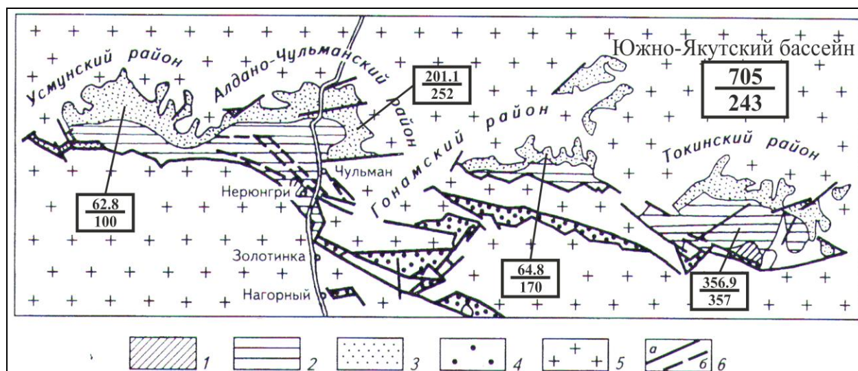
Рис. 6. Схема распределения перспективных для извлечения и промышленного использования ресурсов метана Южно-Якутского бассейна: 1 – нижнемеловые отложения, 2 – средне-верхнеюрские отложения, 3 – нижнеюрские отложения, 4 – юрские отложения нерасчлененные, 5 – архейский фундамент, 6 – основные разломы: установленные (а), предполагаемые (б). В кружках: метаноресурсные показатели: в числителе перспективные для извлечения ресурсы метана, млрд м 3 , в знаменателе плотность распределения, млн м 3 /км 2
