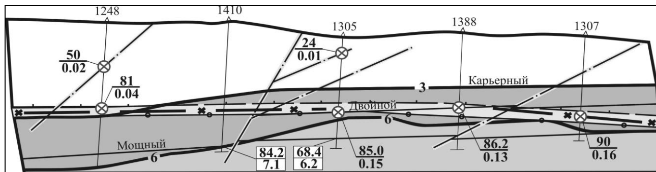
Рис. 4. Схематический геолого-газовый разрез по зоне «сухих» таликов Беринговского бассейна: в кружках – свободные метанопроявления: в числителе \text{CH}_4 в %, в знаменателе \text{CH}_4 в \text{м}^3/\text{мин} ; в квадратах – метаноносность угольных пластов: в числителе \text{CH}_4 в %, в знаменателе \text{CH}_4 в \text{м}^3/\text{т.с.б.м.} ; (–6–) – изогаз метана \text{м}^3/\text{т.с.б.м.} ; светло серым цветом выделена залежь свободного газа в зоне сухих таликов с концентрациями метана 81–95 % и давлением газа 0,25 МПа. Масштаб 1 : 5000
