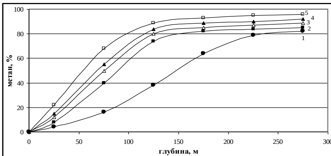
Рис. 2. Изменение средних концентраций метана в угольных пластах месторождений Анадырского (1, стадия метаморфизма угля O_3-I-II ), Аркагагинского (2, I-II ), Беринговского (3, I-III-IV ), Омсукчанского (4, VII-X ) и Зырянского (5, I-X ) углегазоносных бассейнов в зависимости от глубины их залегания
