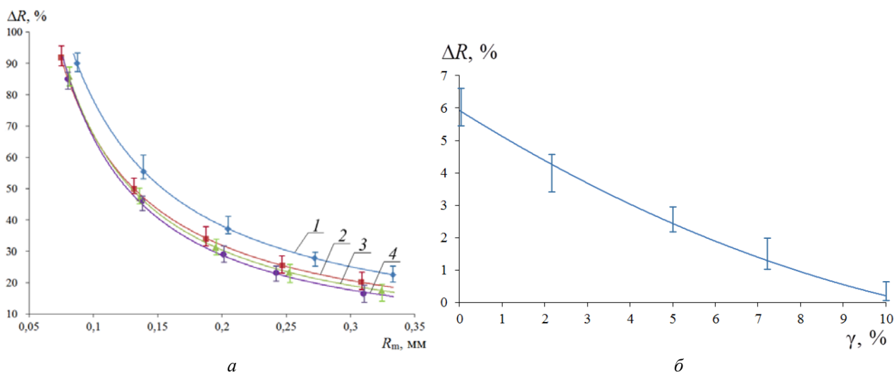
Рис. 8. Зависимости ( T_w=300 К, T_g=1100 К) параметра \Delta R от примесей солей в воде \gamma для полидисперсного потока (а) и одиночных капель (б): 1 – при \gamma=0 %, 2 – при \gamma=2,5 %, 3 – \gamma=5 %, 4 – \gamma=10 %
