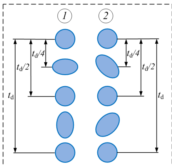
Рис. 2. Условные изображения капель жидкости при реализации первого (1) и второго (2) «режимов деформации»
