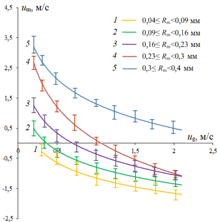
Рис. 11. Зависимости ( T_w=300 К, T_g=1100 К) скоростей каплей жидкости u_m от значений u_g
