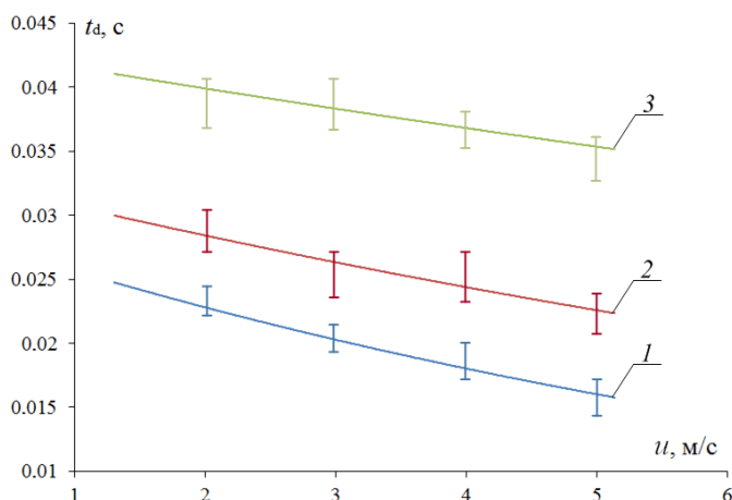
Рис. 5. Зависимости времен t_d от скоростей капель при различных значениях d_0 ( T_w=300 К, T_g=300 К): 1 - для d_0 \approx 3,4 мм; 2 - для d_0 \approx 4,6 мм; 3 - для d_0 \approx 5,8 мм
