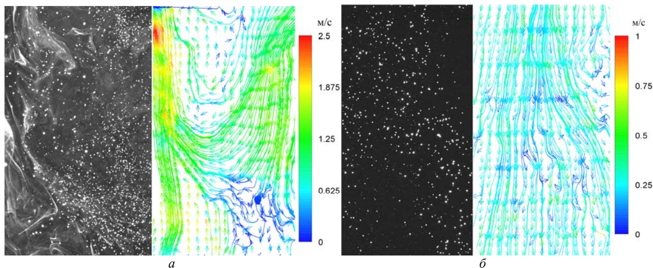
Рис. 10. Видеограммы ( T_w=300 К, T_g=1100 К) каплей жидкости и скорости «трассирующих» частиц на входе (а) и выходе (б) из канала с высокотемпературными газами при u_g=1 м/с, u_m=1,5 м/с
