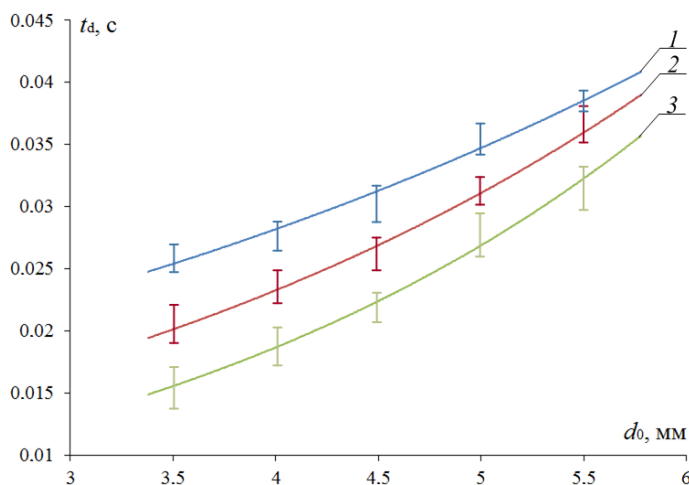
Рис. 4. Зависимости времен t_d от размеров капель при различных значениях u ( T_w=300 К, T_g=300 К): 1 - для u \approx 1,3 м/с; 2 - для u \approx 2,9 м/с; 3 - для u \approx 4,7 м/с
