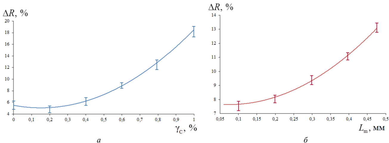
Рис. 9. Зависимости ( T_w=300 К, T_g=1100 К) параметра \Delta R от относительной массовой концентрации углеродистых частиц \gamma_c для капель с R_d = 3 мм и L_m = 50\text{--}70 мкм (а), от размеров включений L_m при \gamma_c=0,5 %
