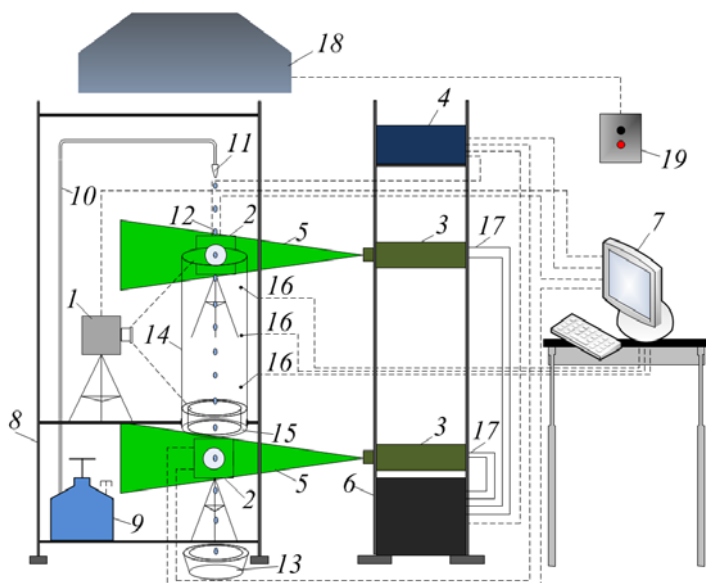
Рис. 1. Схема экспериментального стенда: 1 – видеокамера; 2 – кросскорреляционная камера; 3 – двойной твердотельный импульсный лазер; 4 – синхронизатор ПК, кросскорреляционной камеры и лазера; 5 – световой «нож»; 6 – генератор лазерного излучения; 7 – ПК; 8 – штатив; 9 – ёмкость с рабочей жидкостью; 10 – канал подачи рабочей жидкости; 11 – дозатор / распылитель; 12 – капли рабочей жидкости; 13 – уловитель; 14 – цилиндр из жаростойкого светопрозрачного материала; 15 – полый цилиндр, во внутреннее пространство которого залита горючая жидкость; 16 – термопары; 17 – канал движения охлаждающей жидкости лазера; 18 – нагнетательная система; 19 – пульт включения/отключения нагнетательной системы.
