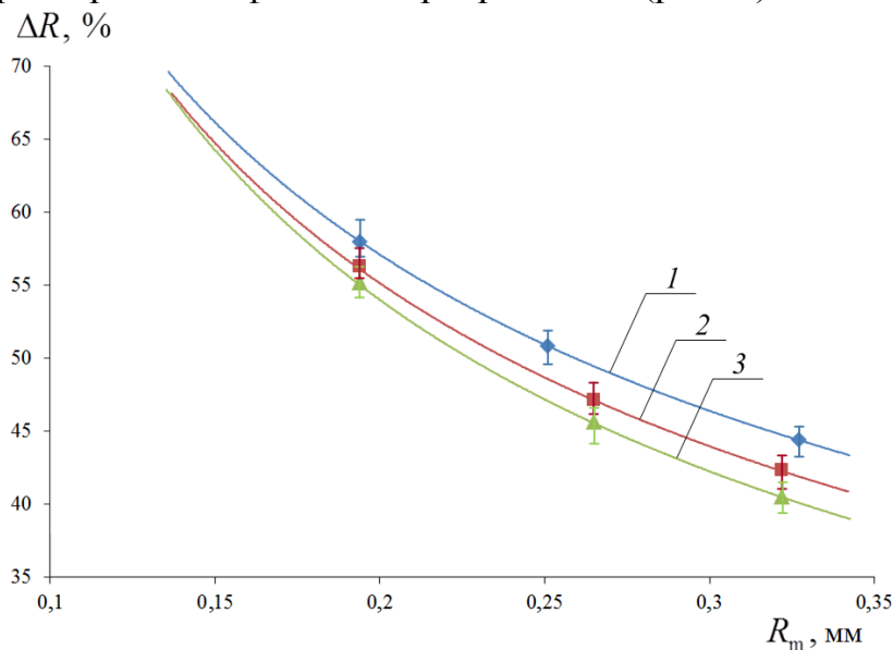
Рис. 7. Зависимости параметра \Delta R от начальных размеров капель распыленной жидкости R_m для различных начальных скоростей u_m : 1 – u_m=0,8 м/с, 2 – u_m=1,1 м/с, 3 – u_m=1,4 м/с
