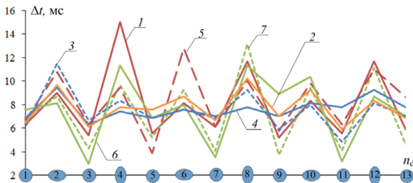
Рис. 3. Времена переходов от одной формы капель воды ( d_0 = 5.3 мм) к другой при их различных температурах и условиях теплообмена с газовой средой: при умеренных температурах газов 1 – T_w=363 К, 2 – T_w=333 К, 3 – T_w=313 К, 4 – T_w=298 К, 5 – «холодный» воздух ( T_g=285 К) и T_w=298 К, 6 – высокотемпературные газы ( T_g=1100 К) и T_w=298 К, 7 – при T_g=1100 К и T_w=363 К
