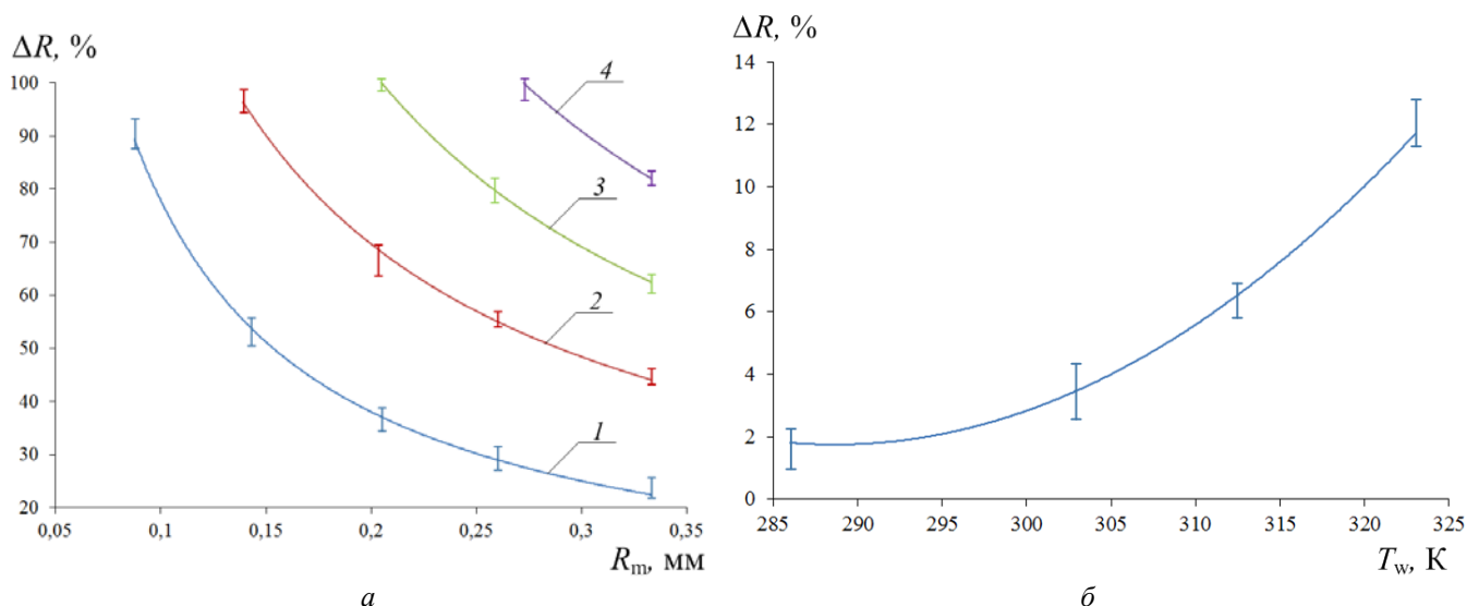
Рис. 6. Зависимости ( T_g=1100 K) параметра \Delta R от начальной температуры воды T_w для полидисперсного потока (а) и одиночных капель (б): 1 – T_w=293 K, 2 – T_w=303 K, 3 – T_w=313 K, 4 – T_w=323 K
