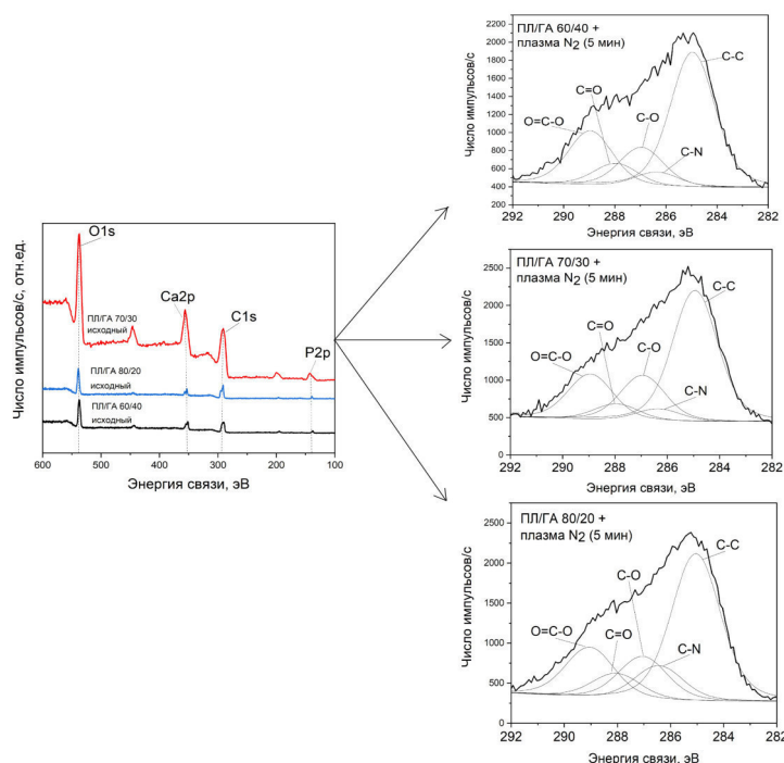
Рис. 1. РФЭ-спектры для композитов ПЛГА 60/40, 70/30, 80/20 до и после обработки плазмой дугового разряда в потоке азота в течении 5 мин
