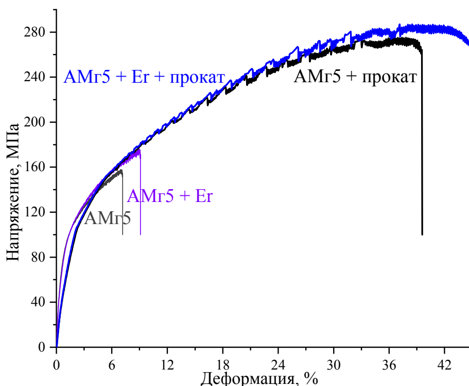
Рис. 1. Деформационные кривые полученных сплавов до и после деформационной обработки
