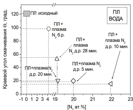
Рис. 2. Изменение значений краевого угла смачивания от концентрации азота после плазменного воздействия на поверхности скаффолдов на основе ПЛ при контакте с водой
