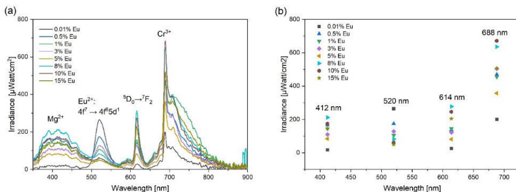
Рис. 2. (а) спектр импульсной катодолюминесценции образцов \text{MgAl}_2\text{O}_4 керамики, активированных ионами \text{Eu}^{3+} переменной концентрации; (б) значения максимальной интенсивности для различных полос излучения
