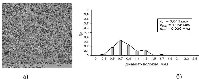
Рис.2. а) СЭМ-изображение скаффолда на основе ПЛ/ГФИП ( C=5\% ); б) распределение диаметра волокон полученного материала
