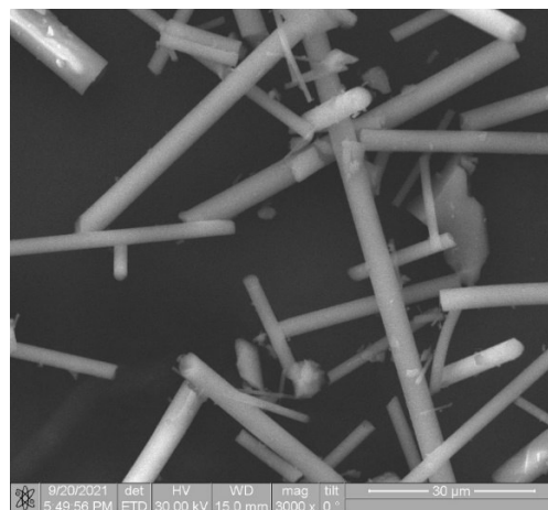
Рис. 3. РЭМ-изображение базальтовых волокон
