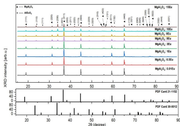
Рис. 1. Рентгеновские дифрактограммы образцов \text{MgAl}_2\text{O}_4 : x\text{Eu} керамики
