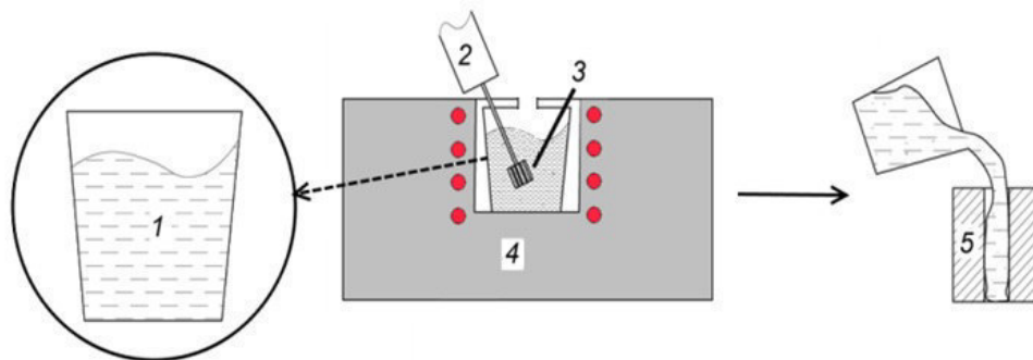
Рис. 1. Схема литья сплавов: 1 – расплав, 2 – механический смеситель, 3 – лигатура, 4 – печь, 5 – кокиль
