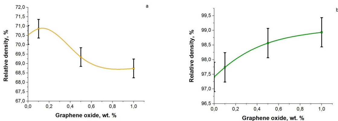
Рис. 2. Зависимость относительной плотности образцов от концентрации оксида графена (а) до спекания; (б) после спекания при температуре 1650°C
