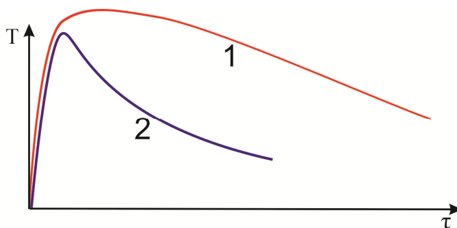
Рис. 1. Типичные температурные профили: 1-естественная, 2- спутная фильтрация
