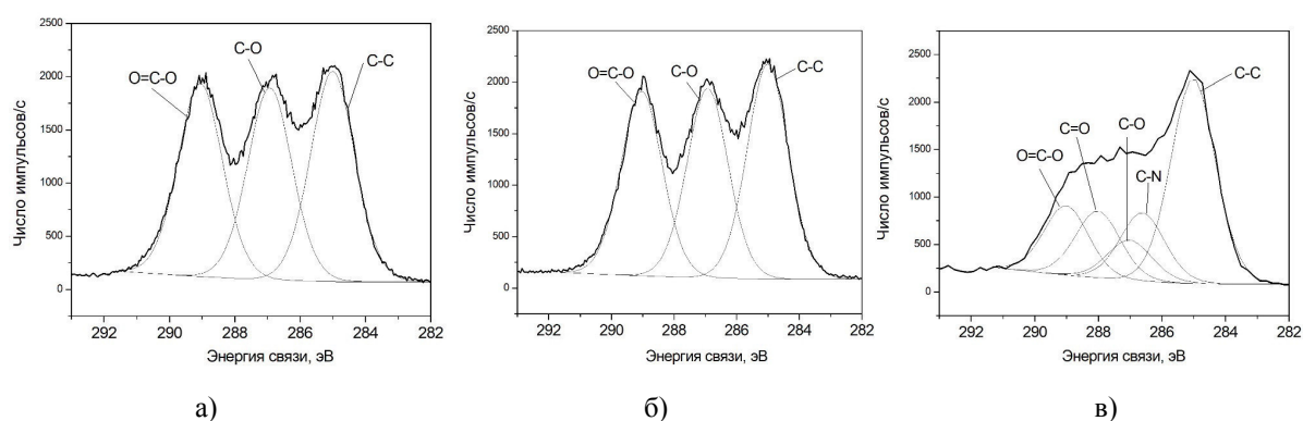
Рис. 1. РФЭС-спектры скаффолдов а) исходного ПЛ; б) ПЛ, обработанного плазмой азота барьерного разряда; в) ПЛ, обработанного плазмой азота дугового разряда (5 минут)
