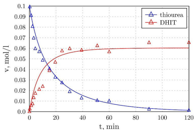
Рис. 2. Кинетические кривые синтеза ДГИТ: треугольники — экспериментальные данные, линия — расчет по модели с найденными коэффициентами
