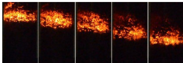
Рис. 2. Распространение фронта горения в режиме спутной фильтрации в азоте при параметрах: q=3.0 \text{ см}^3/(\text{с}\cdot\text{см}^2) ; 70 % AlN+ 30 %Al
