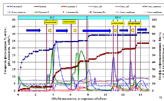
Рис. 1. Фильтрационные характеристики модели неоднородного пласта из карбонатного кернового материала (исходная газовая проницаемость первой и второй колонки 0,832 и 0,341 мкм 2 )
