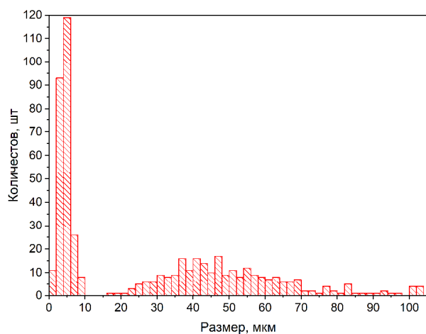
Рис. 2. Гистограмма распределения базальтовых волокон по размерам
