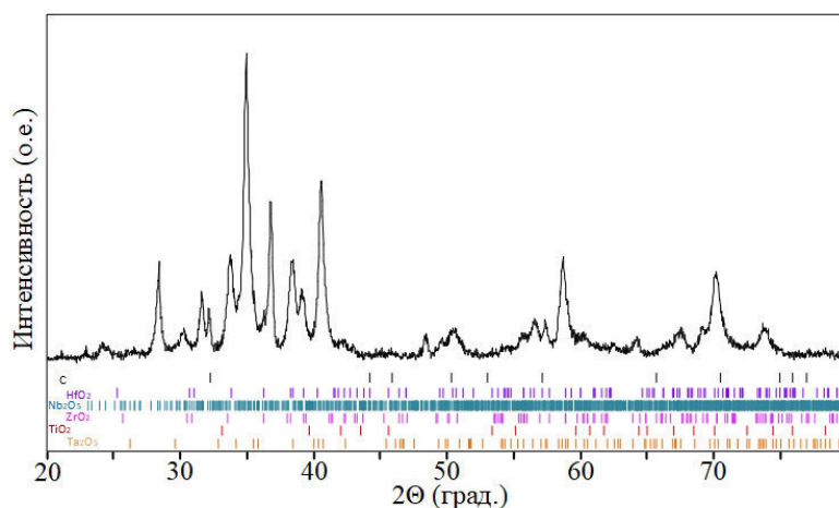
Рис. 1. Типичная картина рентгеновской дифрактометрии
