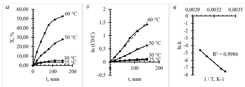
Рис. 4. Кинетические кривые (а); графическое определение константы скорости (б), энергии активации (в)
