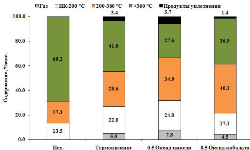
Рис. 1. Фракционный состав термического и каталитического крекинга в присутствии соединений никеля и кобальта
