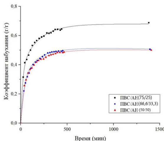
Рис. 2. Залежність коефіцієнта набухання гідрогелевих гранул складу ПВС/АН від часу в дистильованій воді при 37 °C
