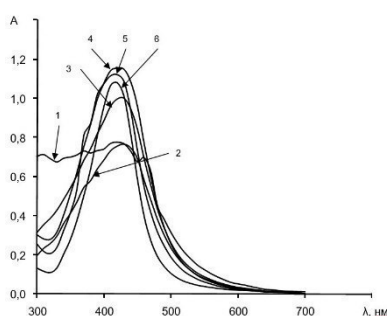
Рис. 3. Спектры поглощения частиц серебра в полиметакрилатной матрице полученные термическим восстановлением. T=140-150 °C, 5 мин (1), 10 мин (2), 15 мин (3), 20 мин (4), 25 мин (5), 30 мин (6)
