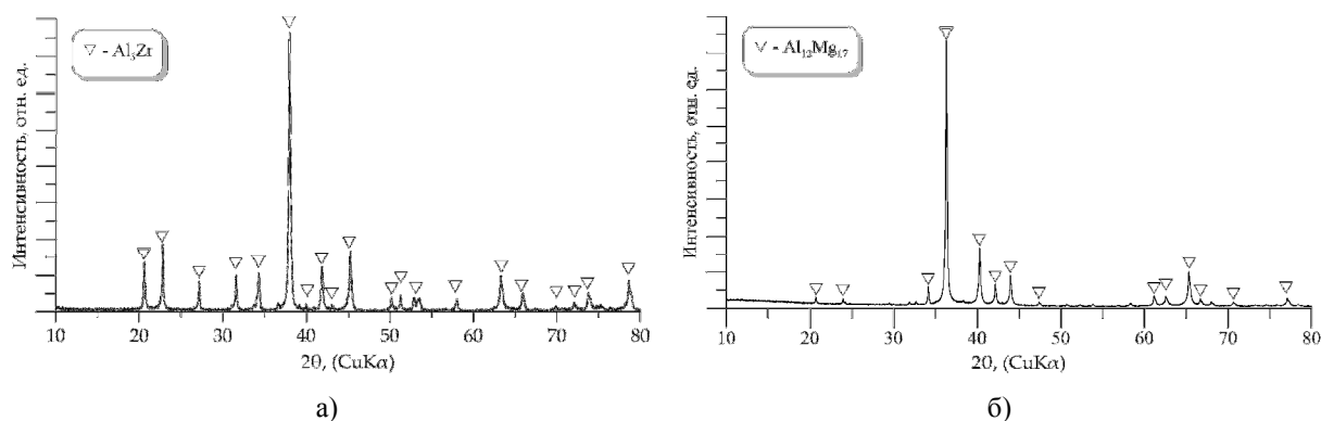
Рис. 1. Дифрактограммы порошковых материалов систем Al-Zr (а) и Al-Mg (б)
