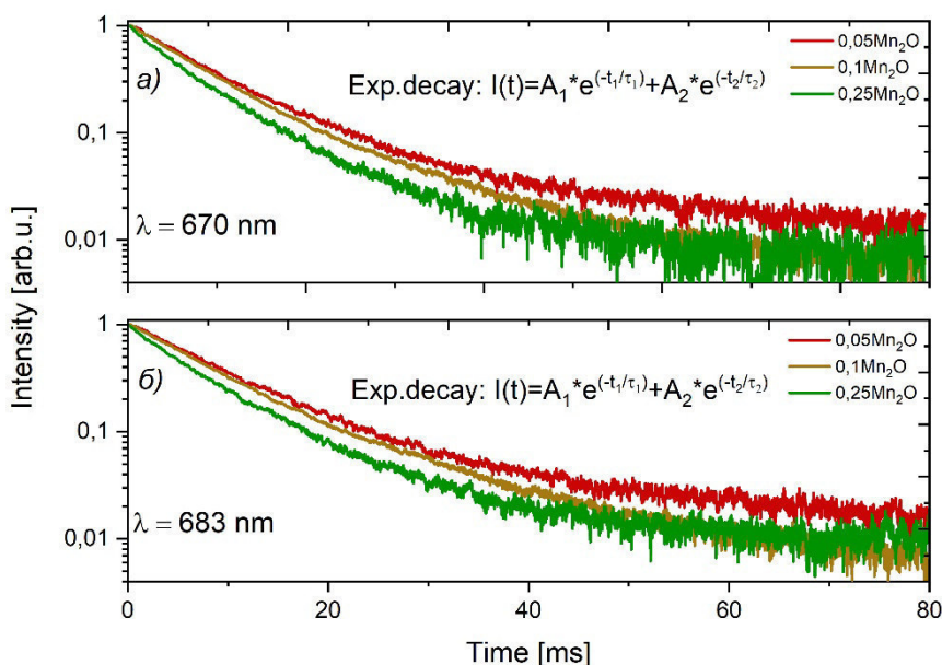
Рис. 2. Кинетика затухания люминесценции литий-германатных стекол (а) при \lambda_{em} = 670 нм и стеклокерамики (б) при \lambda_{em} = 683 нм с различным содержанием MnO_2
