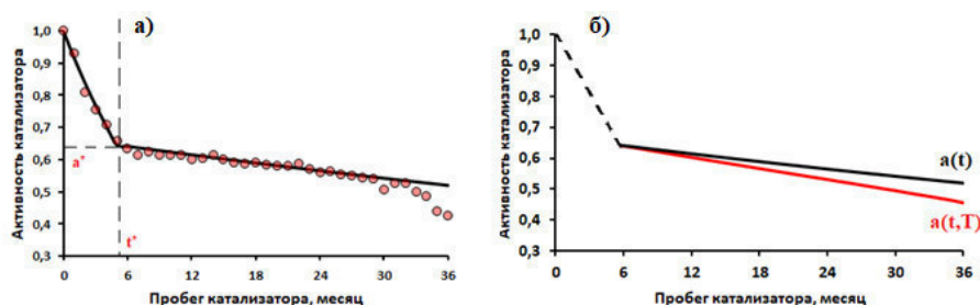
Рис. 2. Функция дезактивации, описывающая экспериментальные данные (а), сравнение функции дезактивации без учета влияния температуры и с ее учетом (б)
