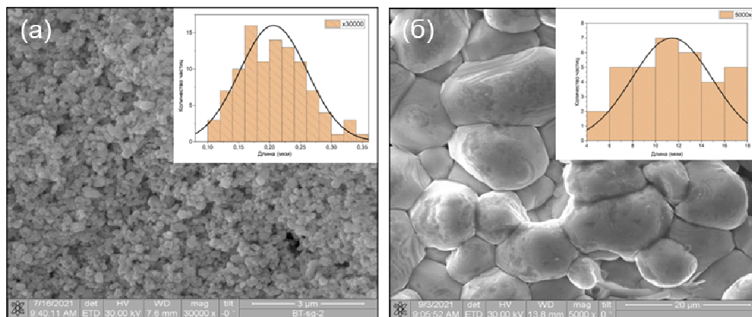
Рис. 1. Микрофотография а) порошка, б) керамики титаната бария
