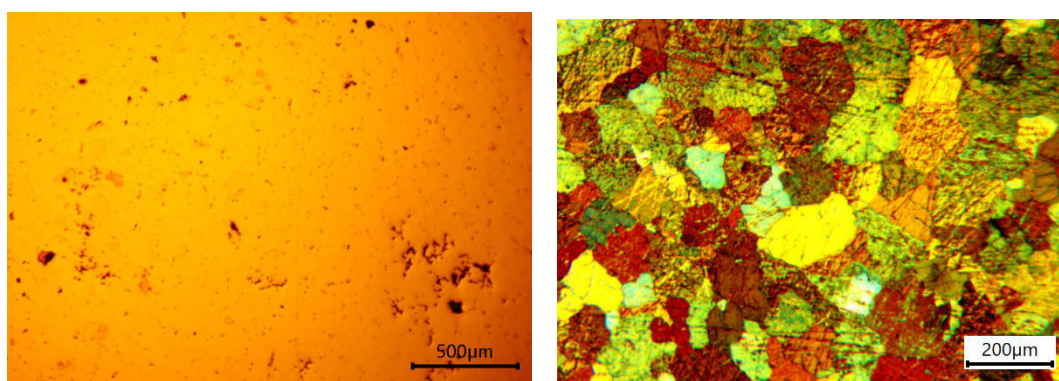
Рис. 1. Оптическое изображение исходного сплава в естественном свете (а); в поляризованном свете (б)
