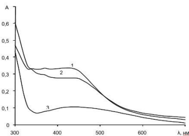
Рис. 2. Спектры поглощения частиц серебра в полиметакрилатной матрице полученные фотохимическим восстановлением. Время фотооблучения ПММ- \text{Ag}^+ : 0,5 мин (1); 3,5 мин (2); 7 мин (3)
