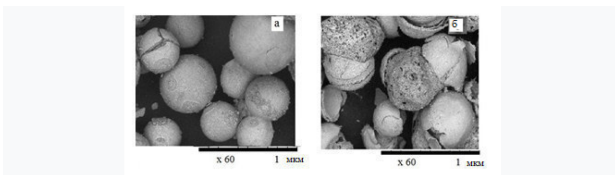
Рис. 1 Микрофотографии образцов (а – ступенчатая термообработка, б – отжиг при 800 °С)
