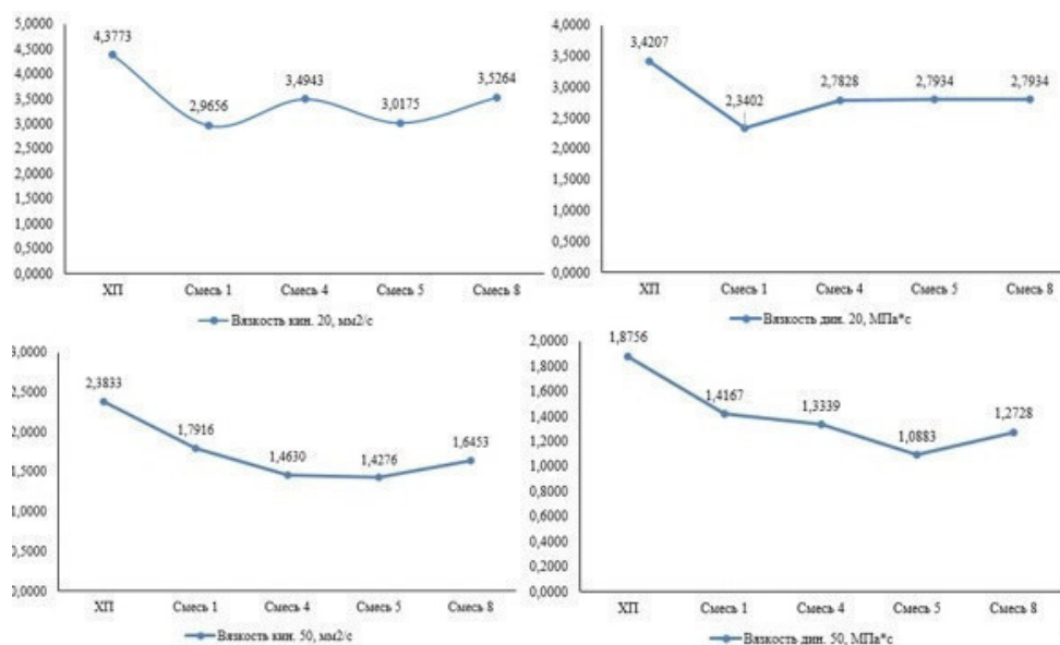
Рис. 2. Изменение кинематической и динамической вязкости (20 и 50 °C) исследуемых образцов в сравнении с холостой пробой
