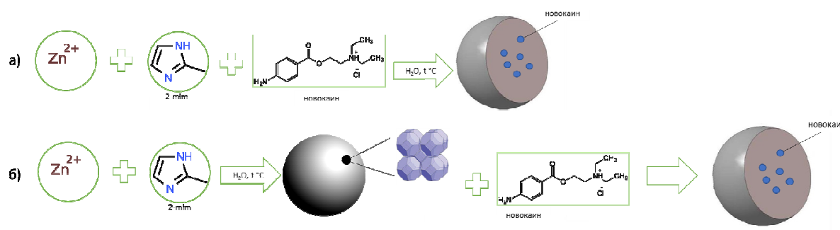
Рис. 2. Схема синтеза лекарственной системы ZIF-8/новокаин: а) одностадийный синтез и б) двухстадийный синтез материала
