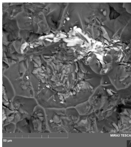
Рис. 1. РЭМ изображение интерметаллида Al-Er на поверхности разрушения сплава AlMg_5 + Er
