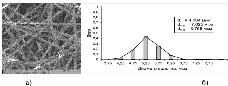
Рис.1. а) СЭМ-изображение скаффолда на основе ПЛ/ХФ ( C=10\% ); б) распределение диаметра волокон полученного материала
