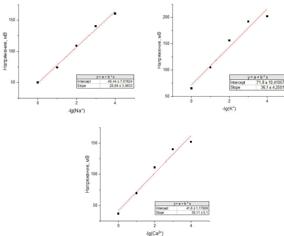
Рис. 1. Калибровочный графики для \text{Ca}^{2+} (a), \text{K}^+ (b), \text{Na}^+ (c)
