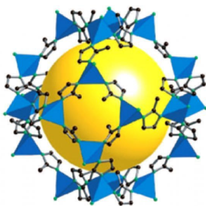
Рис. 1. Кристалічна структура ZIF-8. Чорні і зелені точки позначають атоми вуглецю і азоту відповідно. Сині тетраедри позначають іони цинку. Тут виключені всі атоми водню. Жовта сфера позначає найбільшу сферу Ван-дер-Ваальса, включену в центральну пору ZIF-8
