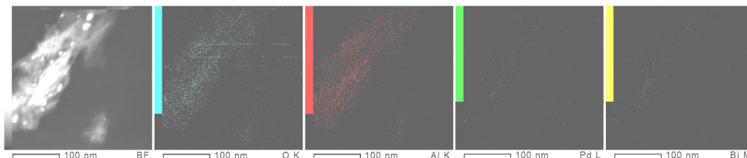
Рис. 1. Результаты ПЭМ-ЭДС картирования поверхности катализатора
