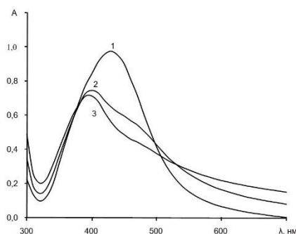
Рис. 1. Спектры поглощения частиц серебра в полиметакрилатной матрице полученные восстановлением аскорбиновой кислотой (1%). Время контакта ПММ- \text{Ag}^+ с раствором аскорбиновой кислоты: 0,5 мин (1); 3,5 мин (2); 7 мин (3)
