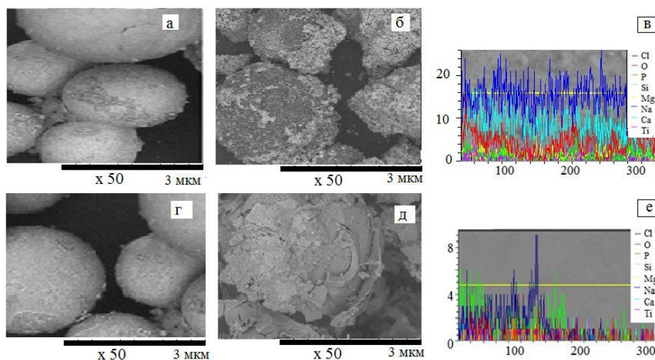
Рис. 2. Микрофотографии поверхности образцов для системы \text{TiO}_2\text{--SiO}_2\text{--P}_2\text{O}_5/\text{CaO} (а, б) и \text{TiO}_2\text{--SiO}_2\text{--P}_2\text{O}_5/\text{MgO} (в, д) до погружения (а, в) и после погружения (б, д) в раствор SBF, распределение элементов по поверхности (е, ф)
