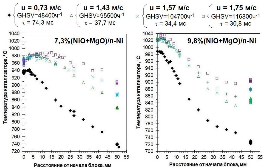
Рис. 1. Температурные профили каталитических блоков при различной линейной скорости подачи реагентов и при \alpha = \text{O}_2/(2 \cdot \text{CH}_4) = 0,3
