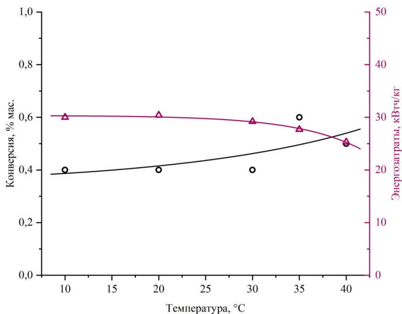
Рис. 2. Зависимость конверсии бензола от температуры реактора при его окислении воздухом в БР
