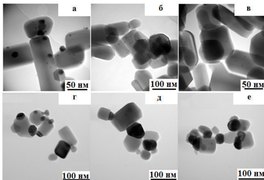
Рис. 1. ПЭМ-изображения наночастиц ZnO-Ag: а) 1 ат.%Ag; б) 0,5 ат.%Ag; в) 0,1 ат.%Ag; г) 12 ат.%Ag; д) 28 ат.%Ag; е) 45 ат.% Ag
