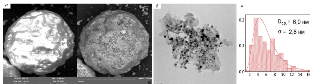
Рис. 2. Микрофотографии СЭМ (а) и ПЭМ (б) исследования поверхности. Гистограмма распределения частиц по размерам (в), где D_{cp} – средний размер частиц, \sigma – СКО
