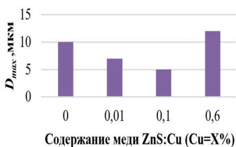
Рис. 2. Распределение диаметров частиц на образцах цинсульфидного люминофора
