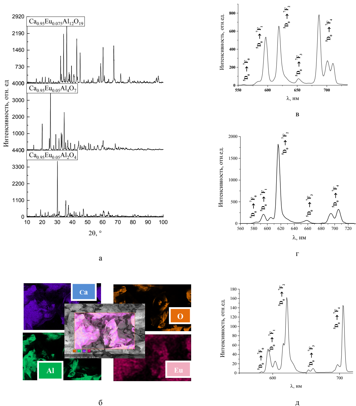
Рис. 1. Дифрактограми люмінофорів з максимальною інтенсивністю свєчення (а); Результати мікрорентгеноспектрального аналізу для \text{Ca}_{0.95}\text{Eu}_{0.05}\text{Al}_2\text{O}_4 (б); Спектри люмінесценції з максимальною інтенсивністю свєчення (в, г, д)
