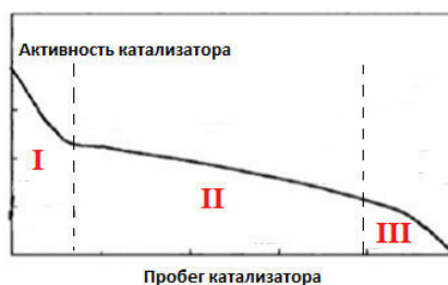
Рис. 1. Типичный вид динамики дезактивации катализатора
