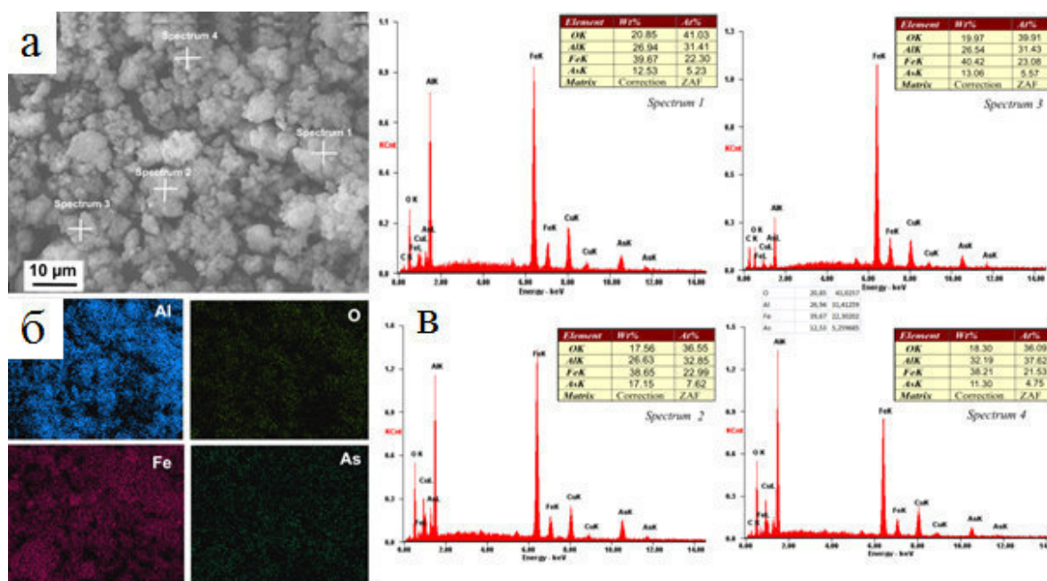
Рис. 1. а) СЭМ-изображения, б) картирование СЭМ-изображений, в) элементный анализ в точках наноструктур AlOOH/Fe после сорбции мышьяка
