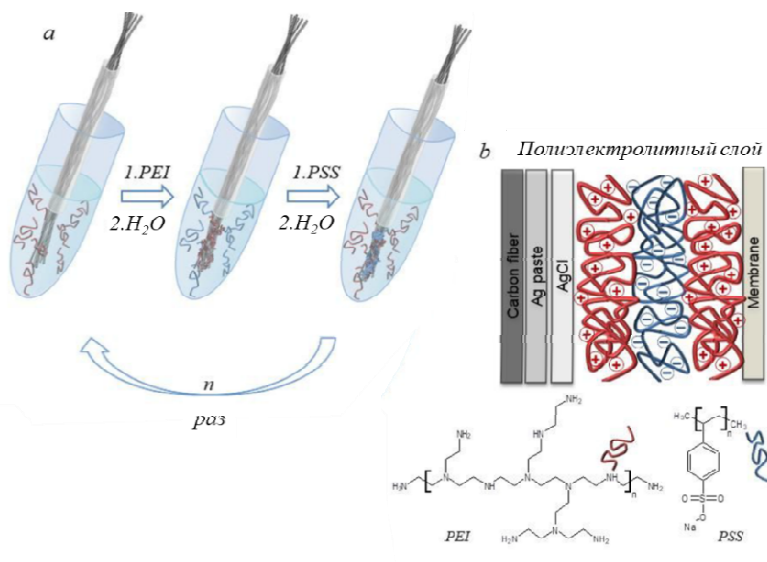
Рис. 1. Модификация углеродного волокна послойной сборкой полиэлектролита (а), общая схема ионоселективного электрода (б)
