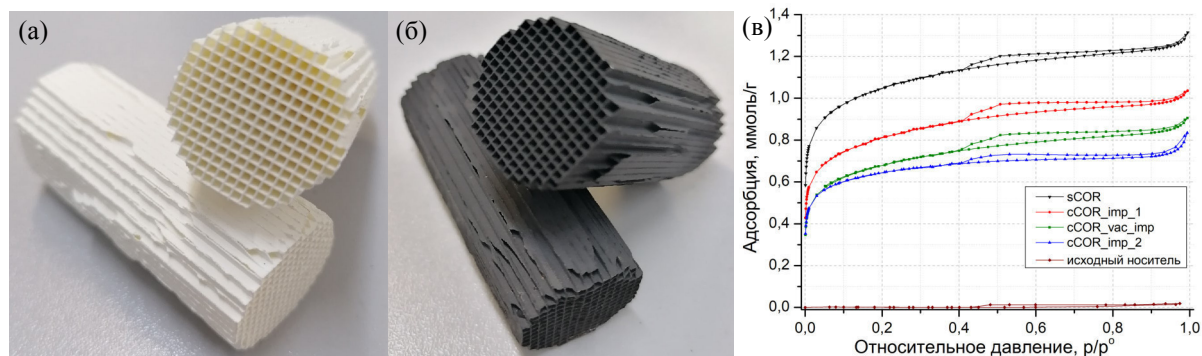
Рис. 1. Внешний вид керамического носителя (а), катализатора на его основе (б) и изотермы адсорбции-десорбции азота для образцов носителя и катализаторов (в)
