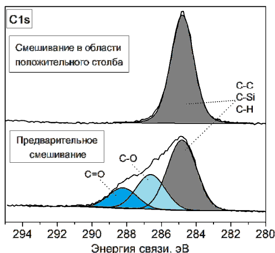
Рис. 1. C1s область РФЭ спектра покрытий, полученных при различном способе подачи ГМДСО
