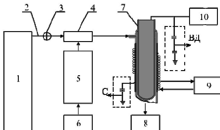
Рис. 1. Схема экспериментальной установки с плазмохимическим реактором
