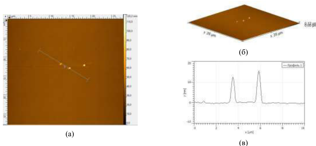
Рис. 1. АСМ изображение поверхности стекла К-208 (а), 3D изображение (б) и профиль по выделенной линии (в)
