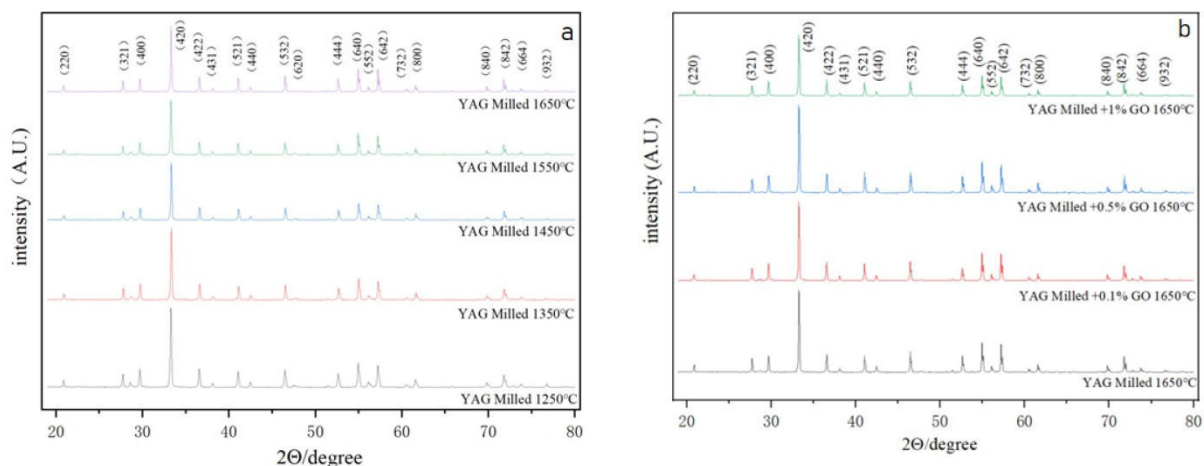
Рис. 1. Дифрактограми образів кераміки (а) отожженні при температурах 1250-1650 °С; (б) с концентрацією оксиду графена 0-1 мас. %
