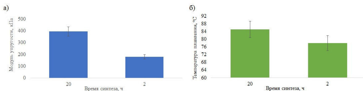
Рис. 1. Влияние времени синтеза на модуль упругости и температуру плавления материала ФК-ПВС (10%)
