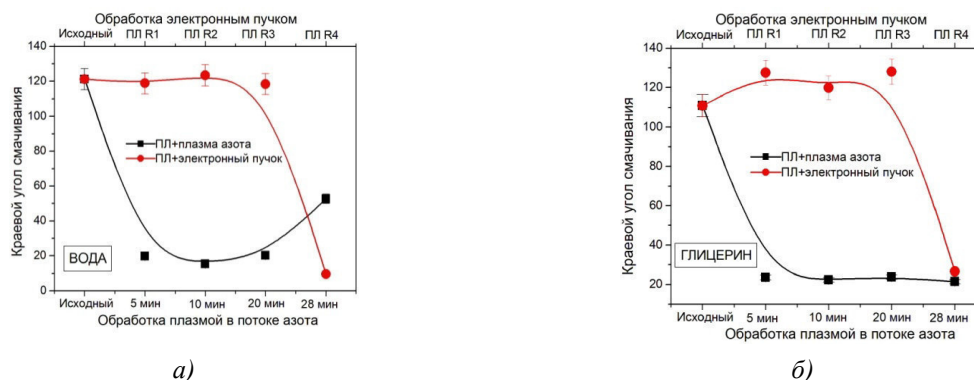
Рис. 1. Краевой угол смачивания, модифицированных скаффолдов на основе ПЛ плазмой азота и электронным пучком при смачивании водой (а) и глицерином (б)
