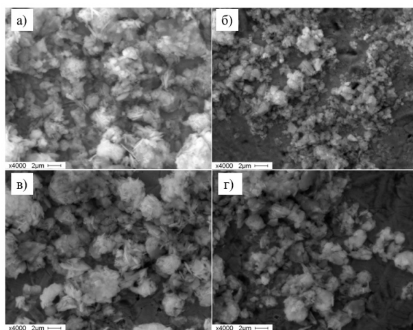
Рис. 2. Морфологія поверхні композиційних матеріалів ФК-ПВС до і після заморожування, при різному часі синтезу: а) синтез 20 годин до заморожування, б) синтез 20 годин після заморожування, в) синтез 2 годин до заморожування, г) синтез 2 годин після заморожування
