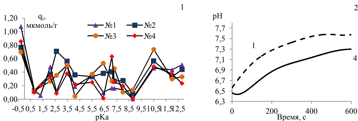
Рис. 1. 1 - Распределение центров адсорбции индикаторов на поверхности композитов на основе нитрида кремния. 2 - Кинетические кривые изменения pH водных суспензий композитов
