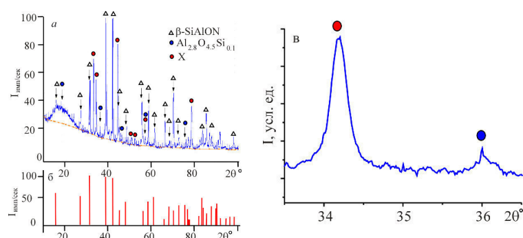
Рис. 3. Дифрактограмма образца, полученного плазмохимическим методом, с использованием Co_{K\alpha} излучения (а), штрих диаграмма \beta -SiAlON состава Si_5AlON_7 (б) из базы данных MatchCrystalImpact и фрагмент рентгенограммы с линией Si_{0.1}Al_{2.8}O_{4.5}
