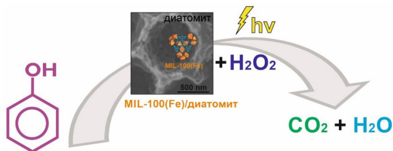
Рис. 2. Схема фотоокисления фенола в реакции Фентона в присутствии MIL-100(Fe)/диатомит
