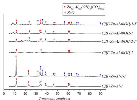
Рис. 1. Дифрактограммы полученных образцов
