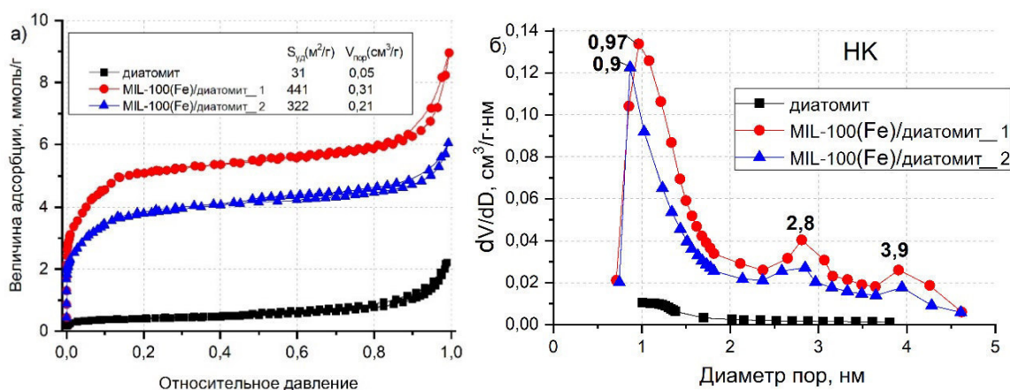
Рис. 1. Изотермы адсорбции-десорбции азота для исследуемых образцов (а) и соответствующие дифференциальные распределения пор по размерам (метод Horward-Kawazoe) (б)
