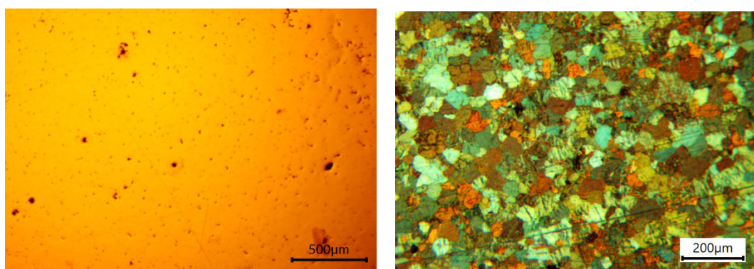
Рис. 2. Оптическое изображение сплава с частицами нанодиама в естественном свете (а); в поляризованном свете (б)
