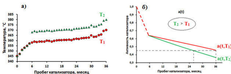
Рис. 3. Сравнение профилей температур T_1 и T_2 (а), динамика снижения активности катализатора в течение времени при различной скорости подъема температуры (б)
