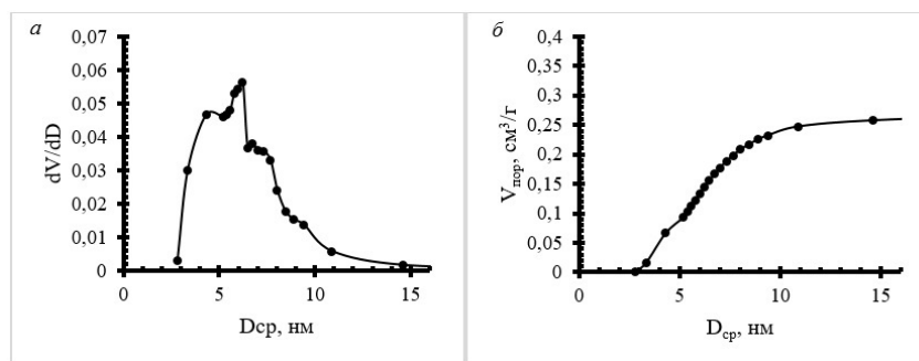
Рис. 3. Дифференциальное (а) и интегральное (б) распределение размеров пор, рассчитанное по методу БДХ
