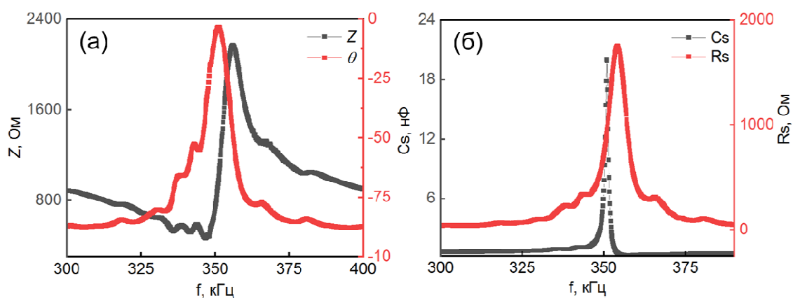
Рис. 1. а) Зависимость импеданса и фазы от частоты, б) зависимости емкости и сопротивления от частоты
