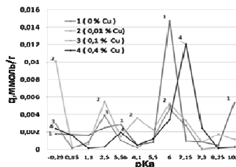
Рис. 3. РЦА на поверхности образцов люминофора ZnS:Cu
