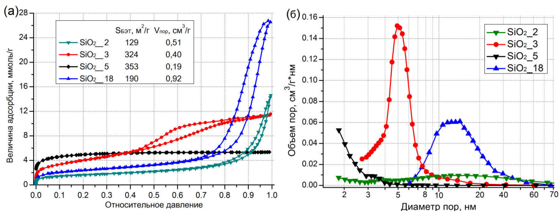
Рис. 2. Изотермы адсорбции-десорбции азота (а) и соответствующие распределения пор по размерам (б) для лабораторных образцов силикагелей, полученных при варьировании pH гелеобразования
