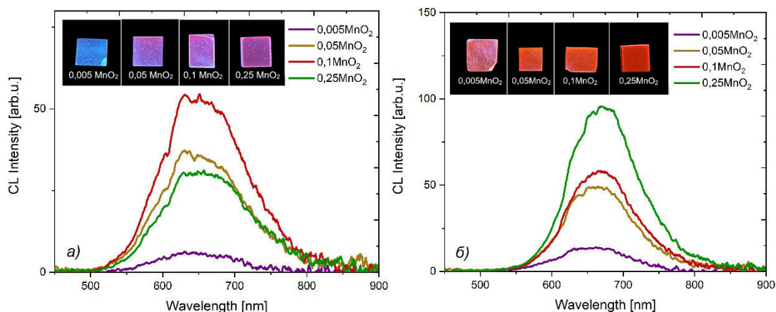
Рис. 1. Спектры импульсной катодолуминесценции литий-германатных стекол (а) и стеклокерамики, отожжённой при 560 °С (б) с различным содержанием MnO_2
