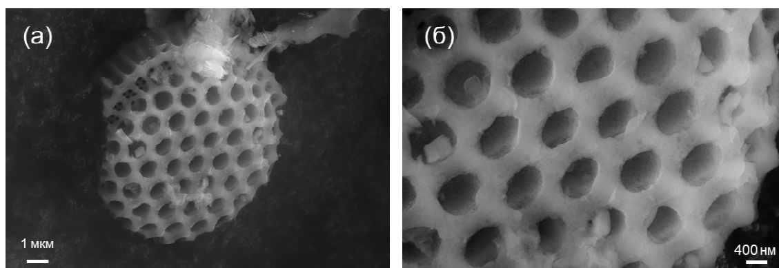
Рис. 1. Результаты сканирующей электронной микроскопии (СЭМ) для исходного диатомита
