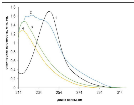
Рис. 2. Спектры поглощения 4-цианофенола ( 5 \cdot 10^{-6} М) в воде без облучения (кр. 1), с добавкой H_2O_2 без облучения (кр. 2), после облучения эксилампой ХеВг (282 нм) в течении 40 мин (кр. 3); в течении 100 мин (кр. 4); в стационарном режиме
