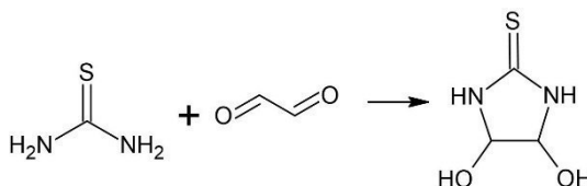
Рис. 1. Схема синтеза ДГИТ
