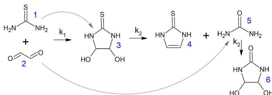
Рис. 3. Схема реакций
