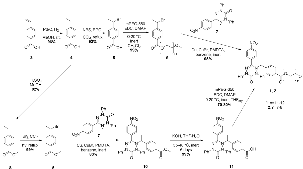
Рис. 1. Схема синтеза пегилированных алкилвердазилов
