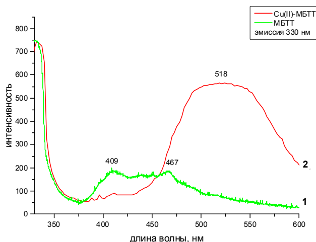
Рис. 1. Спектр люминесценции органического лиганда (3-метилбензотиазол-2-тионом) (1) и координационного соединения меди (II) на его основе (2)
