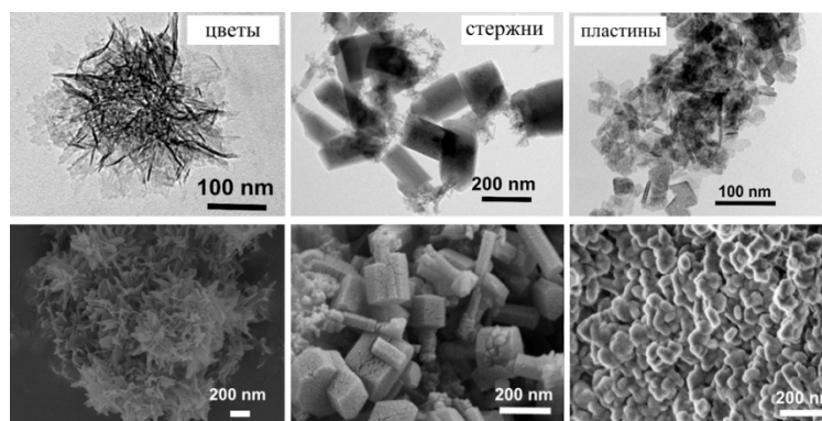
Рис. 1. Электронно-микроскопические изображения наноструктур
