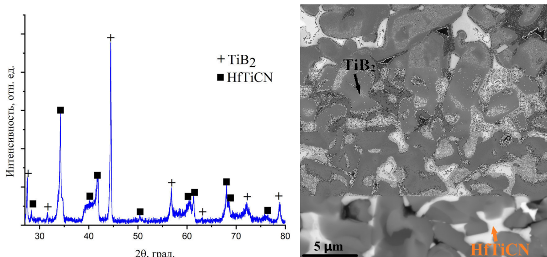
Рис. 1. а) Дифрактограмма продуктов синтеза; б) РЭМ-изображение продуктов синтеза
