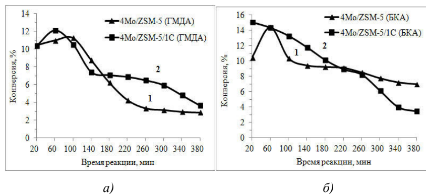
Рис. 1. Изменение конверсии метана со временем работы катализаторов К-1 (а) и К-2 (б), полученных с использованием цеолитов с микро (1) и микро-мезопористой (2) структурой
