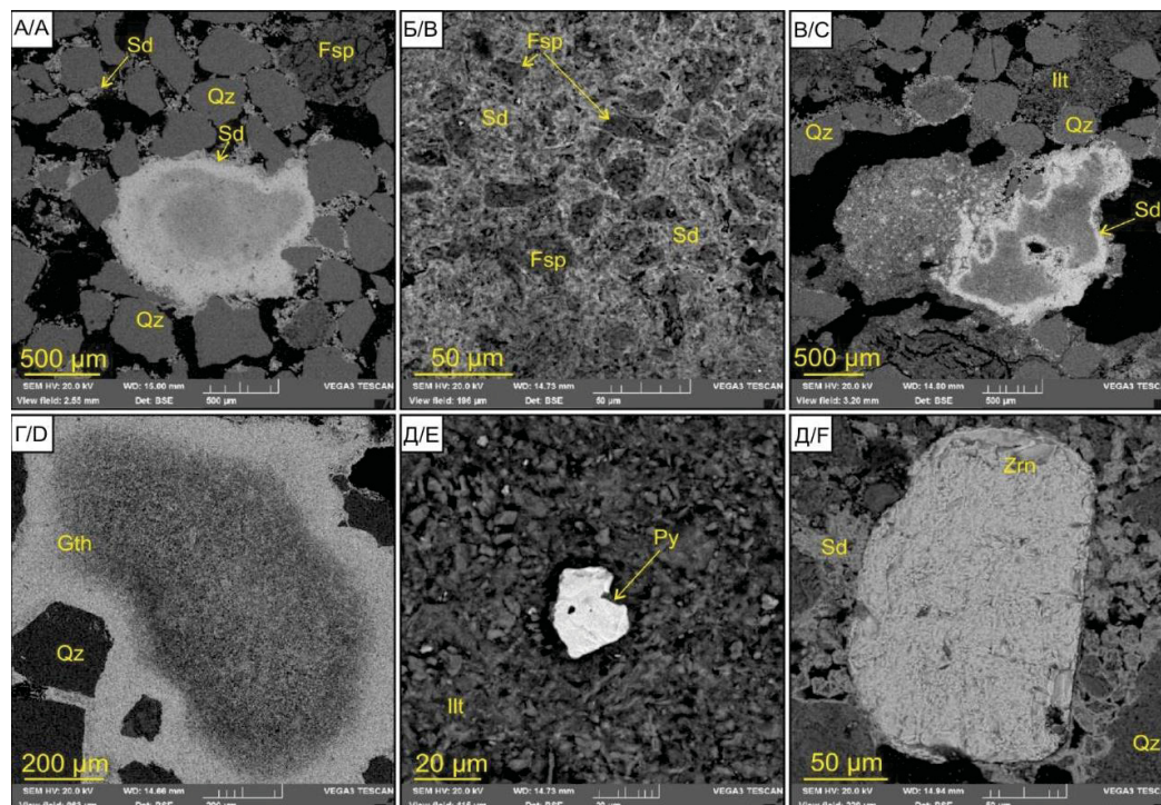
Рис. 3. СЭМ-снимки минералов в железяках кочковской свиты Киреевского проявления: А) сидерит в виде микроконкреций или цемента; Б) сидеритовый цемент железяков; В) пленочные формы сидерита в гравелите; Г) микроконкреции гётита; Д) пирит в иллитовом матриксе; Е) крупный акцессорий циркона среди сидеритового цемента железяка. Gth – гетит, Ill – иллит, Py – пирит, Qz – кварц, Sd – сидерит, Zrn – циркон
