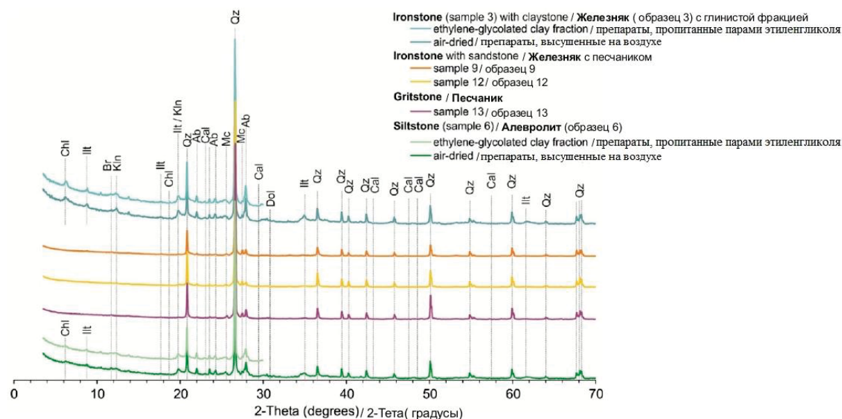
Рис. 4. Рентгеновские дифрактограммы репрезентативных образцов железяков, вмещающих пород и их глинистых фракций. Ab – альбит, Br – брусит, Cal – кальцит, Chl – хлорит, Dol – доломит, Ill – иллит, Kln – каолинит, Mc – микроклин, Qz – кварц
