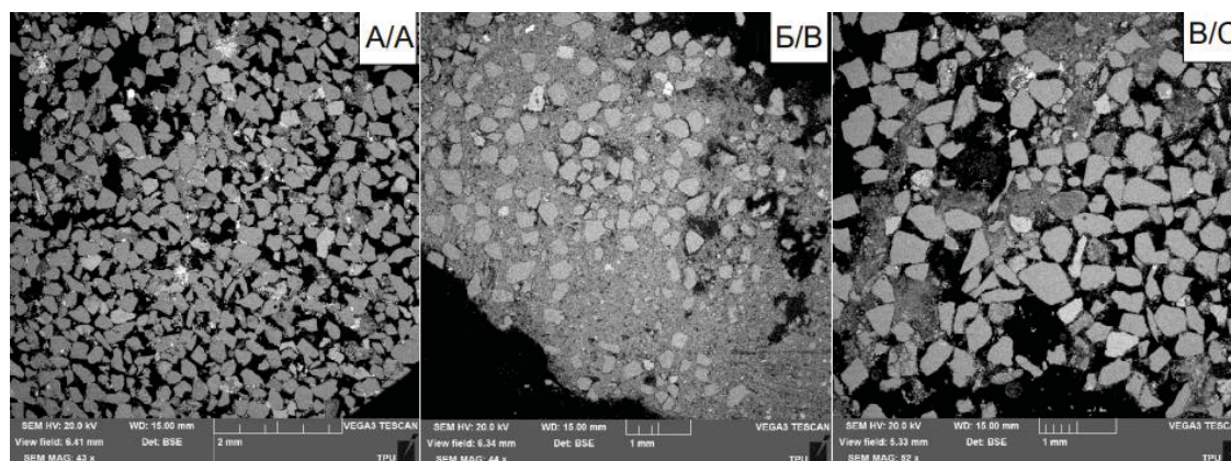
Рис. 2. СЭМ-снимки образцов в кочковской свите Киреевского проявления (А) песчаник среднезернистый, слабоцементированный (Б) алевропесчаник с глинистыми стяжениями (В) железяк мелко-среднезернистый
