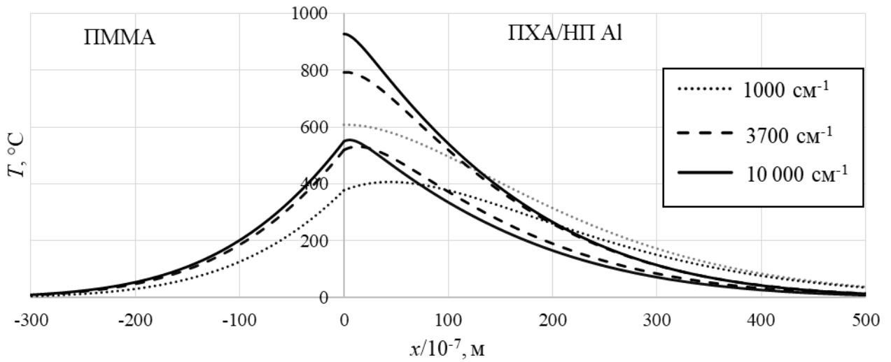
Рисунок 4.2 – Температурные профили нагрева двухслойной системы ПММА – ПХА/НП Аl для \mu = 1000 \text{ см}^{-1} , 3700 \text{ см}^{-1} , 10\,000 \text{ см}^{-1}
