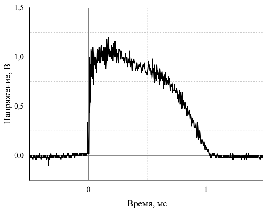
Рисунок 2.4 – Кинетика импульса излучения используемого в работе лазера
