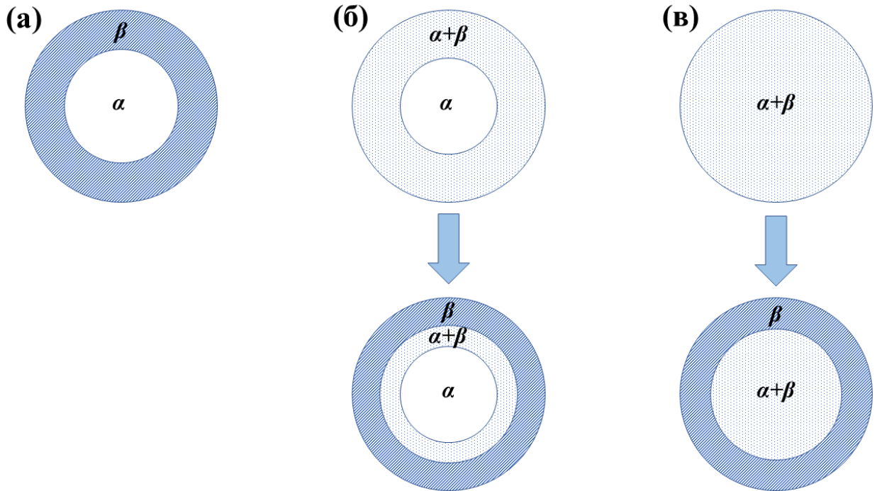
Рисунок 26 – Модель кинетики гидрирования. (а) модель без двухфазной ( \alpha + \beta ) области (непрерывно движущаяся граница); (б) модель с определенной шириной двухфазной области \alpha + \beta ; (в) модель полной двухфазной ( \alpha + \beta ) области на начальной и поздней стадиях соответственно [41].
