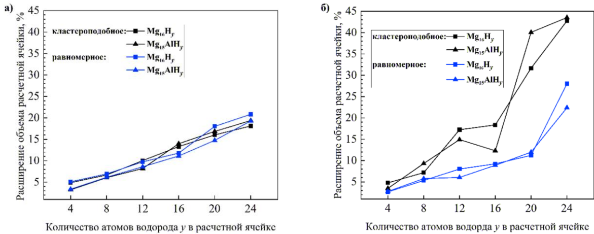
Рисунок 30 – Расширение объема расчетной ячейки в зависимости от количества атомов водорода y в релаксированной ГЦК \text{Mg}_{16-x}\text{Al}_x\text{H}_y (а) and ОЦК \text{Mg}_{16-x}\text{Al}_x\text{H}_y (б) ( x = 0, 1 ).
