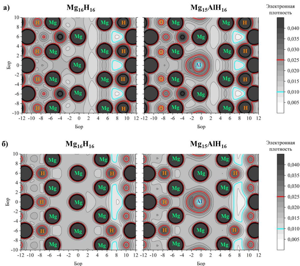
Рисунок 34 – Распределение электронной плотности в рассмотренной плоскости а) (110) и б) ( \bar{1}10 ) \text{Mg}_{16-x}\text{Al}_x\text{H}_{16} , с водородом на расстоянии от алюминия. Красная и светло-голубая изоповерхности соответствуют плотности заряда 0,025 и 0,01 электрон/Бор 3 соответственно. Шкала градаций серого цвета дана в единицах электрон/Бор 3 . Атомы магния обозначены зелеными, атомы алюминия обозначены темно-синими, атомы водорода обозначены оранжевыми.
