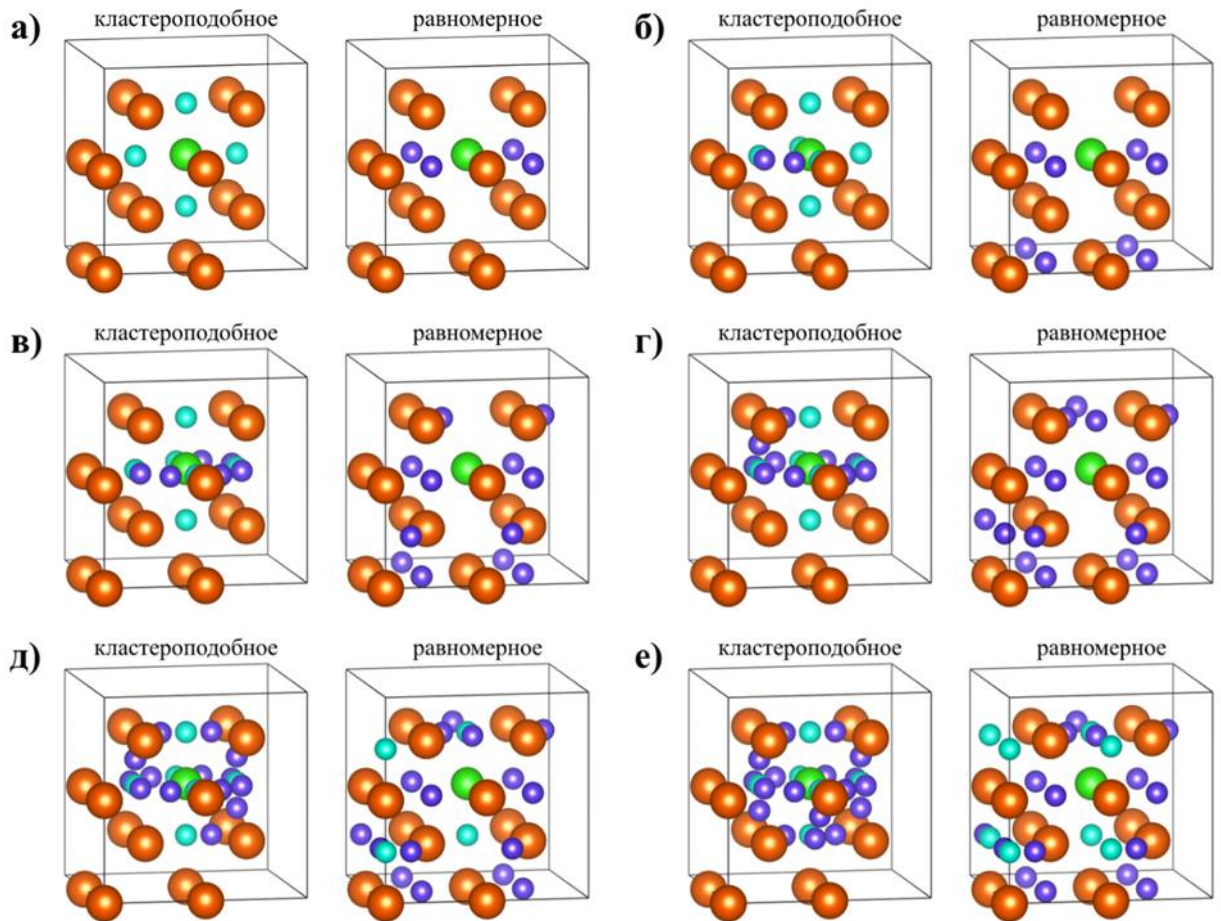
Рисунок 28 – Суперячейки для ОЦК (а) \text{Mg}_{16-x}\text{Al}_x\text{H}_4 , (б) \text{Mg}_{16-x}\text{Al}_x\text{H}_8 , (в) \text{Mg}_{16-x}\text{Al}_x\text{H}_{12} , (г) \text{Mg}_{16-x}\text{Al}_x\text{H}_{16} , (д) \text{Mg}_{16-x}\text{Al}_x\text{H}_{20} , и (е) \text{Mg}_{16-x}\text{Al}_x\text{H}_{24} . x = 0, 1 . Левая колонка – кластер атомов
