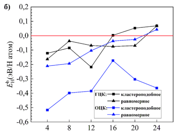
Рисунок 29 – Энергия связи водорода в зависимости от количества атомов водорода y в релаксированных суперячейках \text{Mg}_{16}\text{H}_y (а) и \text{Mg}_{15}\text{AlH}_y (б) с кластерным и равномерным распределением водорода.
