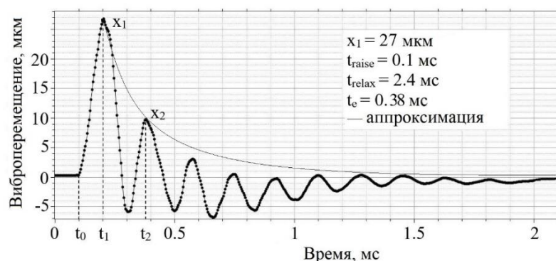
Рисунок 14 – Колебания мембраны газоразрядного излучателя, выведенной из состояния покоя импульсом искрового разряда
