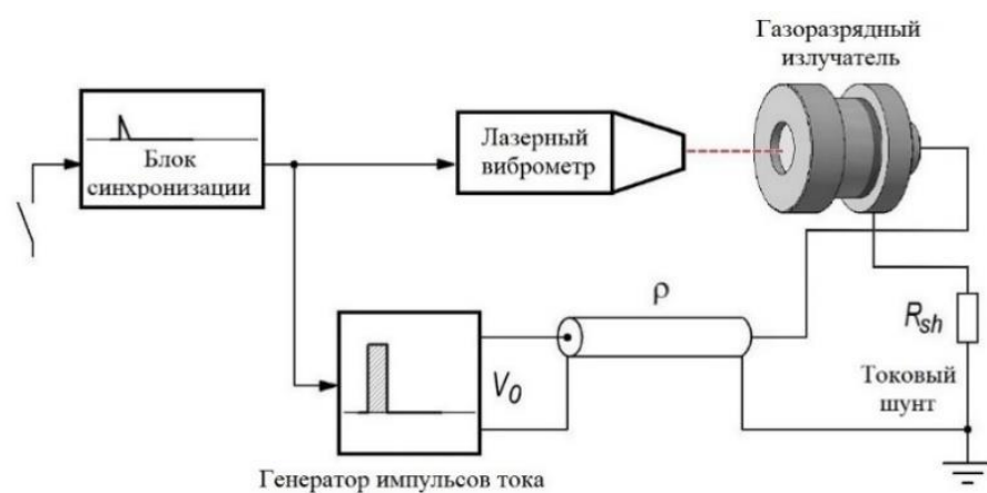
Рисунок 13 – Функциональная схема установки для исследования вибрационных характеристик газоразрядного излучателя
