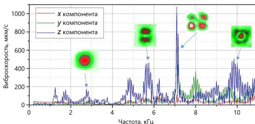
Рисунок 3 – Амплитудно-частотный спектр колебаний пластины ПММА в диапазоне частот от 50 Гц до 10 кГц (а)
