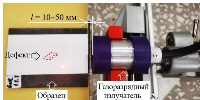
Рисунок 20 – Акустическая стимуляция углепластикового композита с ударным повреждением 15 Дж с использованием газоразрядного излучателя
