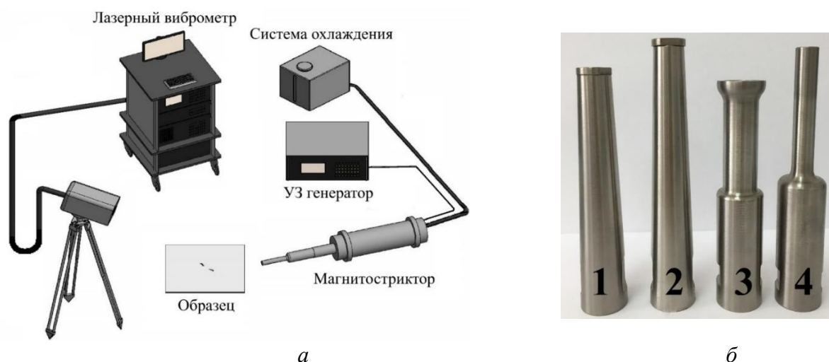
а – схема экспериментальной установки, б – фотография волноводов
