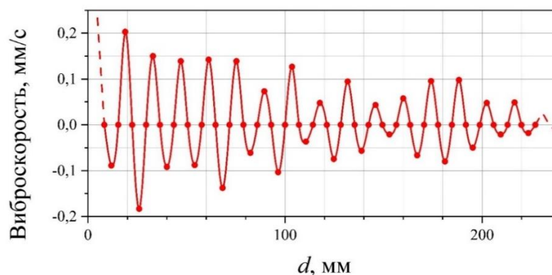
Рисунок 10. Распределение амплитуды виброскорости в воздушной среде на расстоянии d до 340 мм между излучателем и исследуемым объектом на частоте 23 кГц
