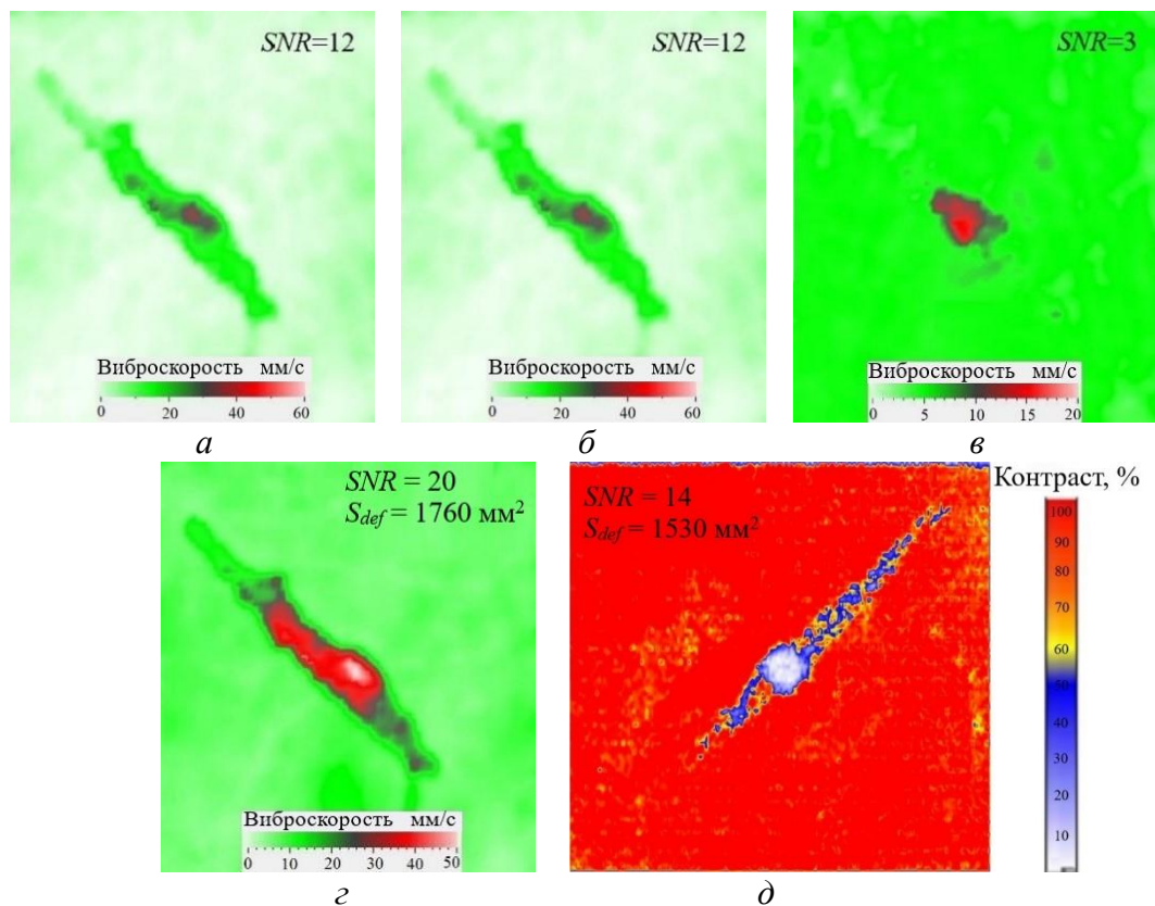
Виброграммы: а – по координате х , б – по координате у , в – по координате z , г – по координатам хуz , д – результаты ультразвукового С -сканирования
