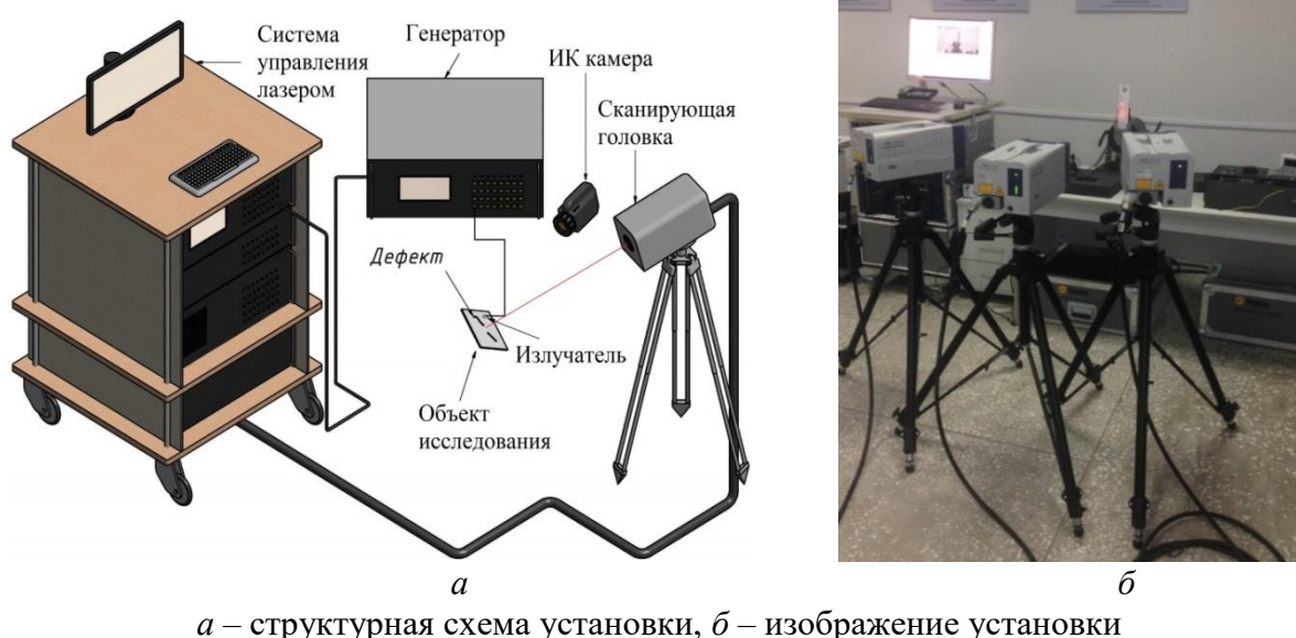
Рисунок 1 – Установка трехкомпонентной СЛДВ при резонансной УЗ стимуляции
