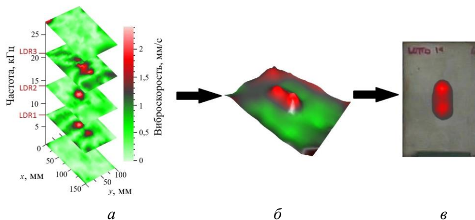
a – анализ амплитудно-частотного спектра колебаний, б – анализ виброграмм на резонансных частотах, в – дефектометрия
