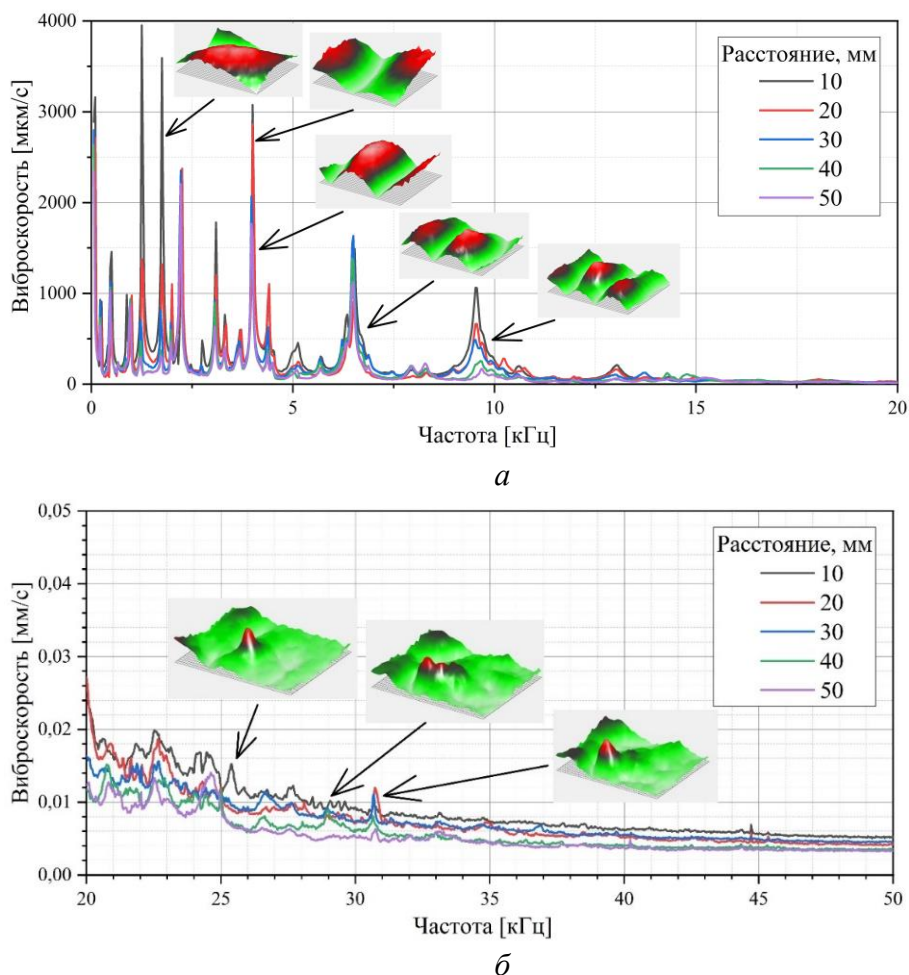
Рисунок 21 – Амплитудно-частотные спектры колебаний углепластика, расстояние излучатель–образец от 10 до 50 мм
