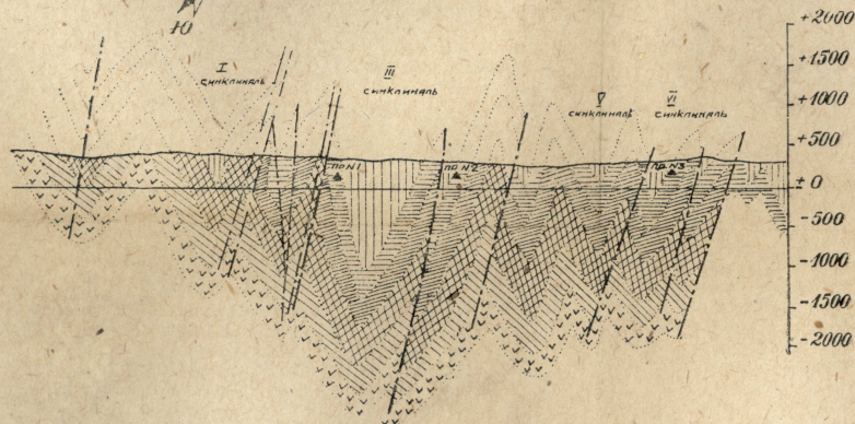
Разрез по линии CD.
