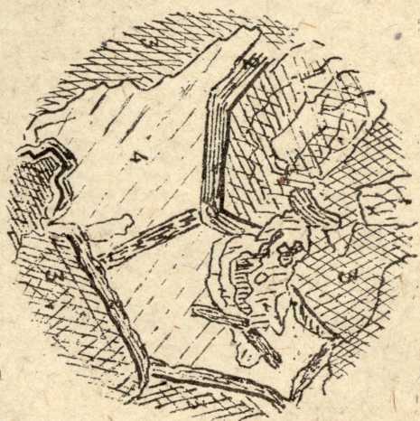
1. Пироксен. 2. Аномальн. гранат. 3. Гранат бурый. 4. Кальцит. Фиг. 3.
