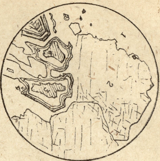
1. Нерудные. 2. Магнетит. 3. Халькопирит. 4. Лимонит. Фиг. 18.
