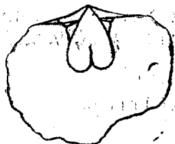
Фиг. 3. Dalmanella sibirica n. sp. Брюшная створка с внутренней стороны.
