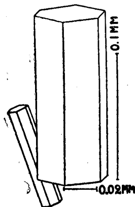
Фиг. 3. Кристалл золота с приросшим другим кристалликом меньшего размера
