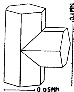
Фиг. 5. Двойник золота
