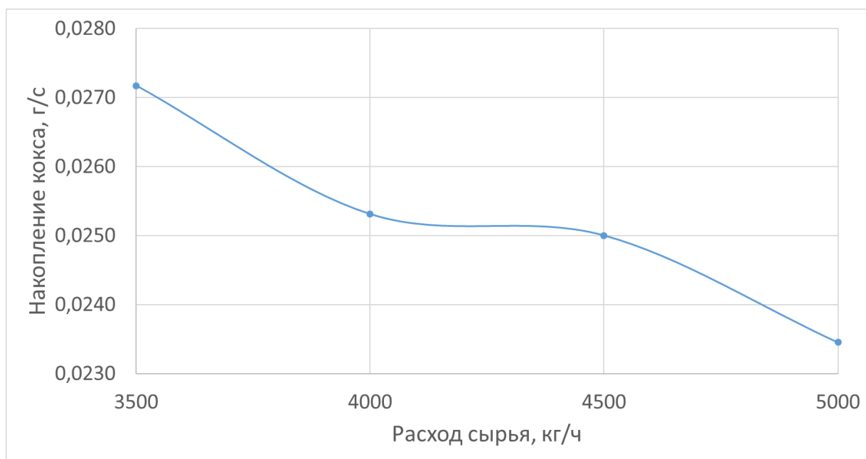
Рисунок 36 – Зависимость скорости накопления кокса от расхода бензиновой фракции
