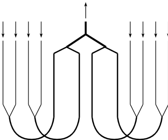
Рисунок 5 – Пример общего вида разветвленного змеевика
