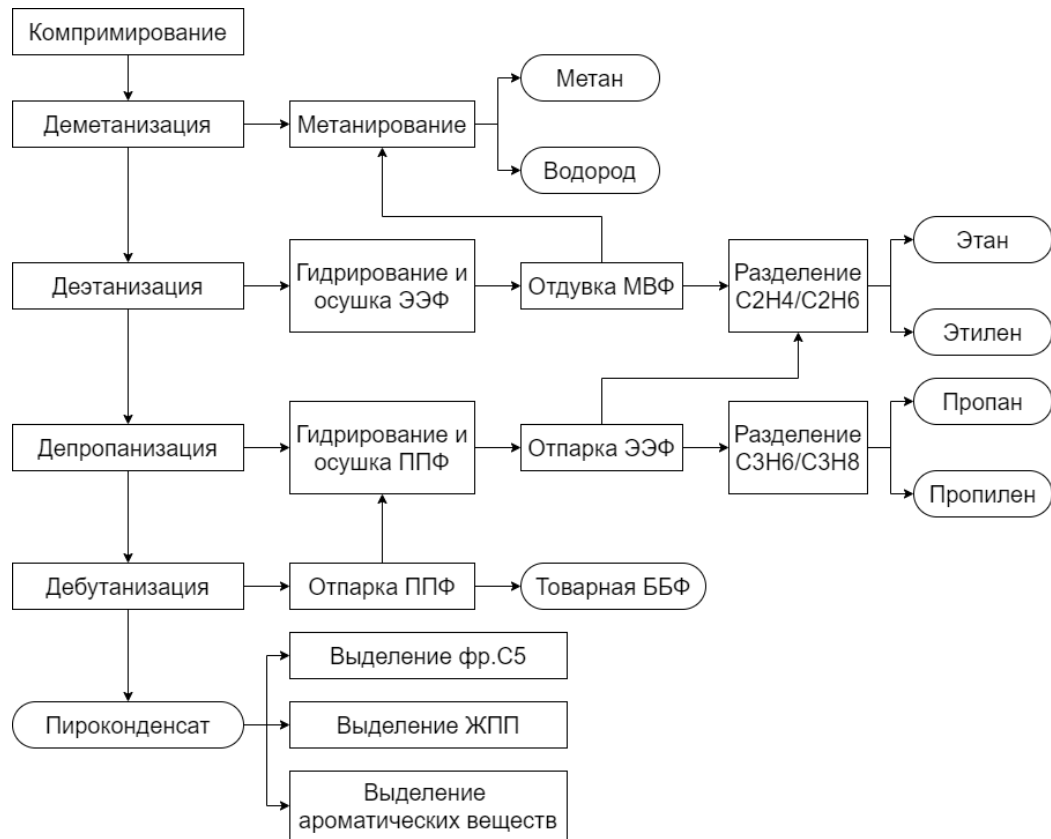
Рисунок 20 – Схема с хвостовым гидрированием
