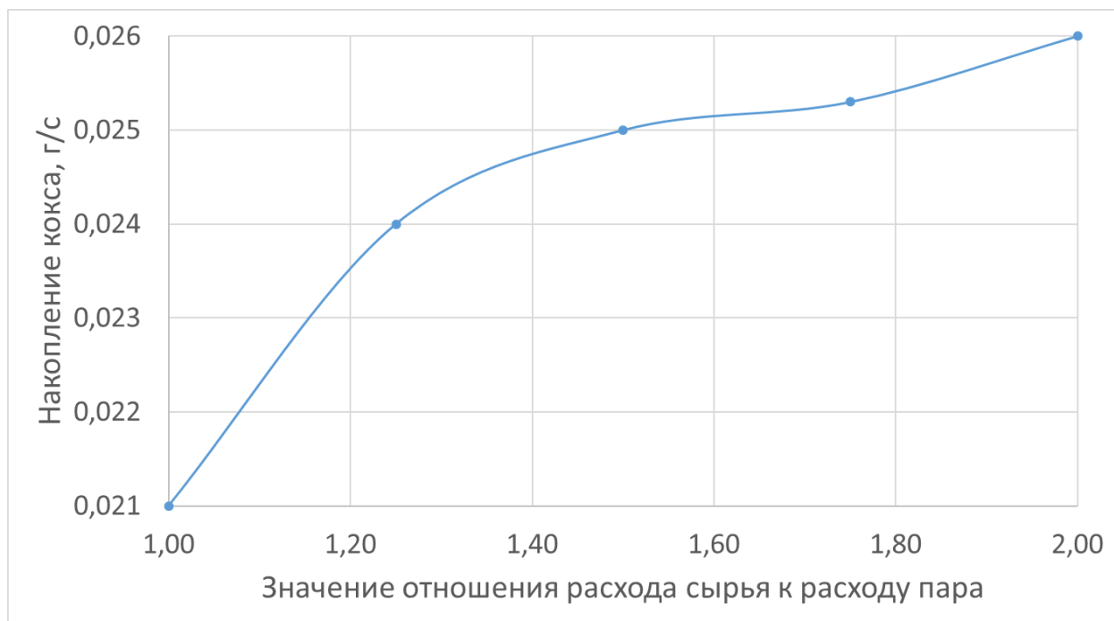
Рисунок 39 – Зависимость скорости накопления кокса от отношения массового расхода сырья к расходу пара
