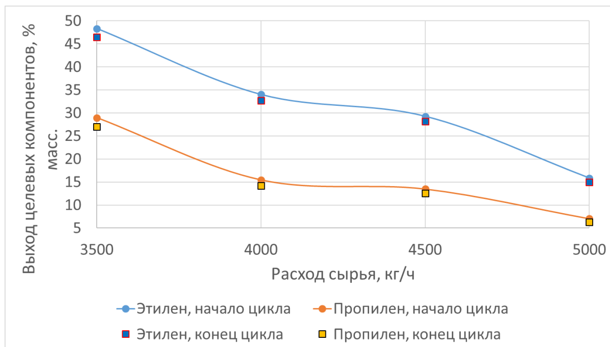
Рисунок 37 – Зависимость выходов этилена и пропилена от расхода сырья
