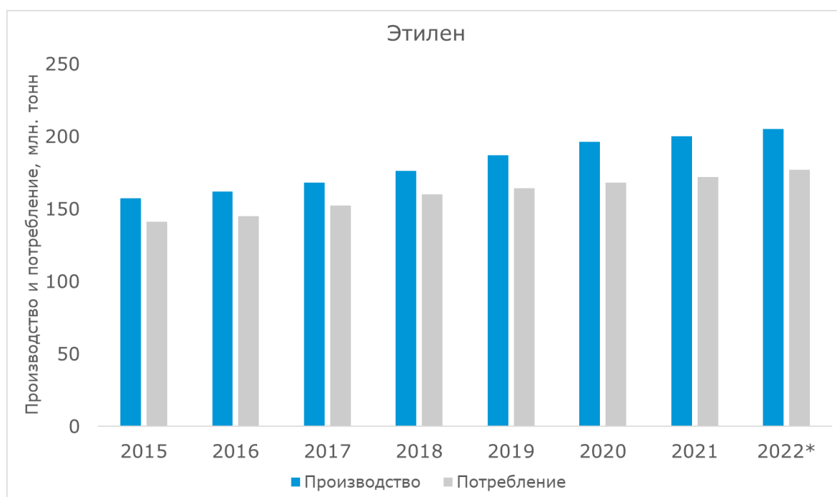
Рисунок 1 – Мировое производство и потребление этилена в период 2015-2022 гг.
