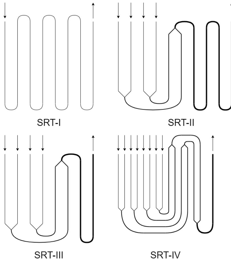
Рисунок 7 – Эволюция змеевиков SRT
