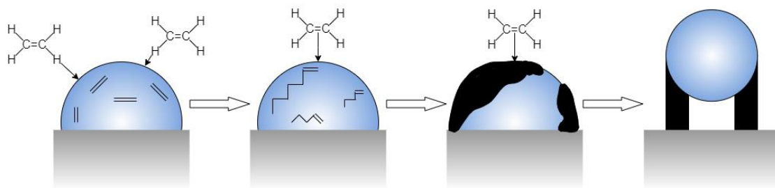
Рисунок 25 – Механизм формирования частицы каталитического кокса [95]
