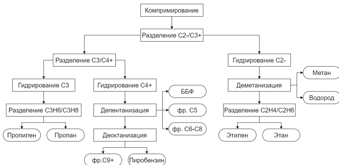
Рисунок 21 - Схема с фронтальным гидрированием
