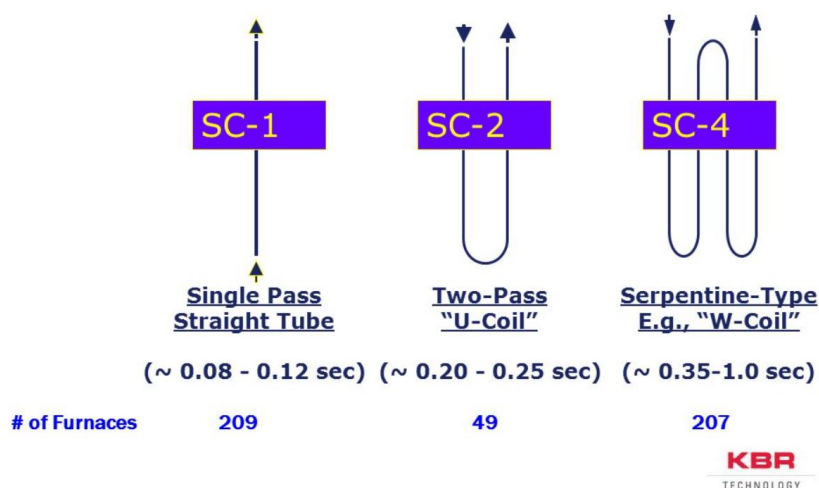
Рисунок 8 – Змеевики серии SC
