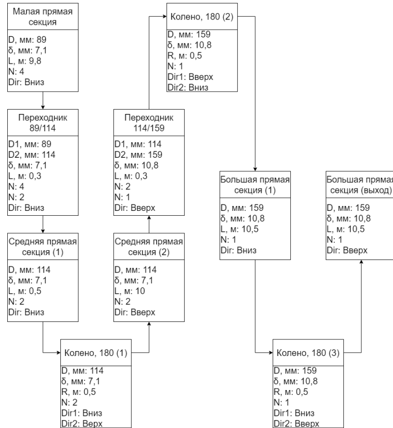
Рисунок 23 – Представление змеевика в виде графа
