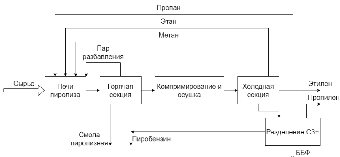
Рисунок 19 – Общее представление секции разделения
