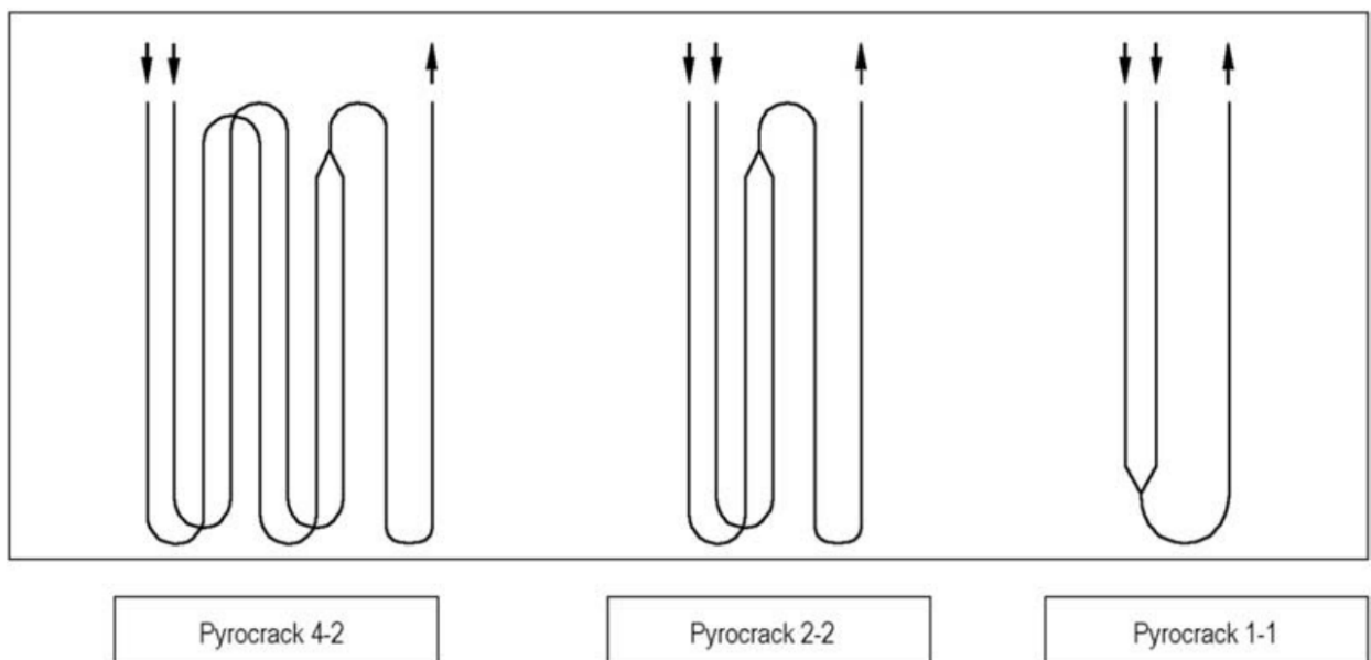
Рисунок 11 – Змеевики серии Pyrocrack
