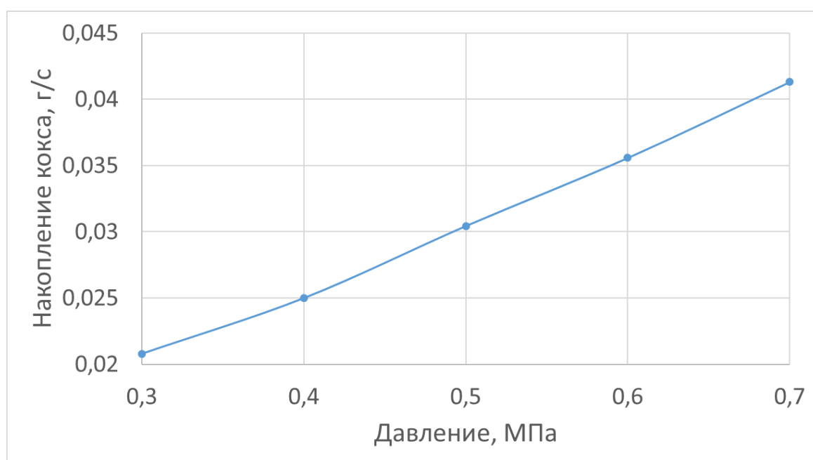
Рисунок 33 – Зависимость скорости накопления кокса от давления сырья
