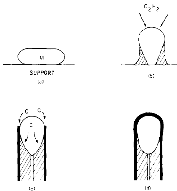
Рисунок 26 – Формирование частицы каталитического кокса [96]. Черная толстая линия обозначает графитовую оболочку, штриховка – аморфный кокс, без окрашивания – частица металла
