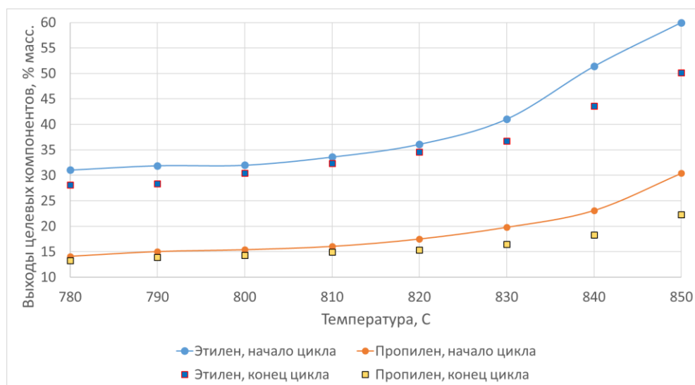
Рисунок 31 – Зависимость выходов этилена и пропилена от температуры паросырьевой смеси
