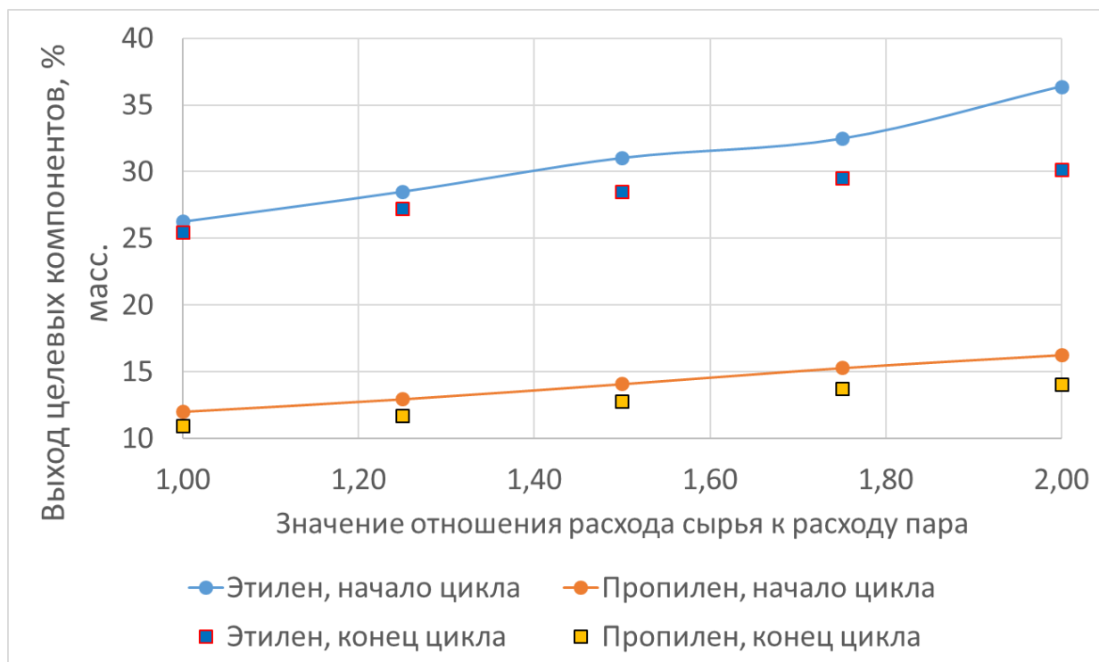
Рисунок 40 – Зависимость выходов этилена и пропилена от соотношения расходов сырья и пара
