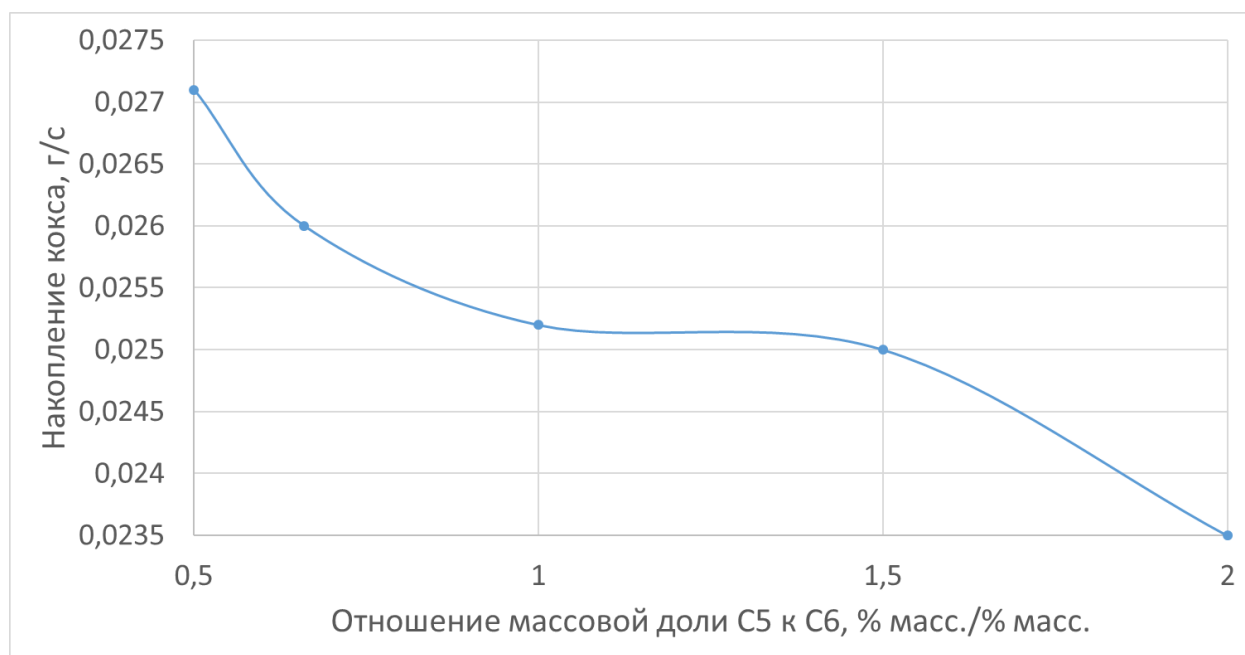
Рисунок 42 – Зависимость накопления кокса от соотношения суммы концентраций изомеров пентана сумму концентраций изомеров гексана
