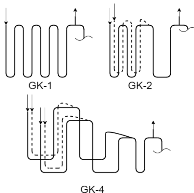
Рисунок 10 – Змеевики серии GK
