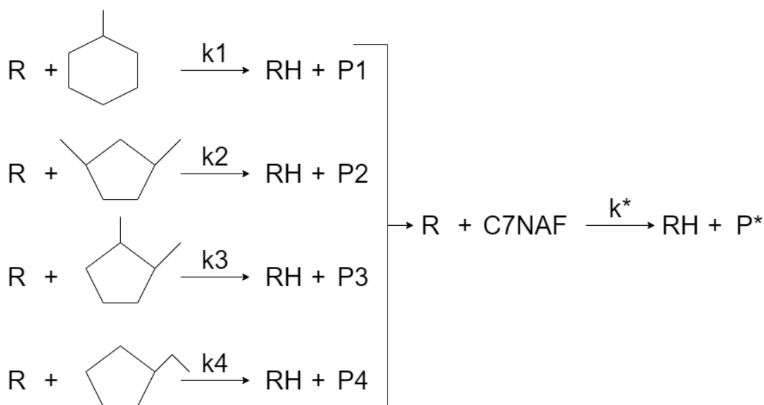
Рисунок 15 – Реакция эквивалентного компонента C7NAF
