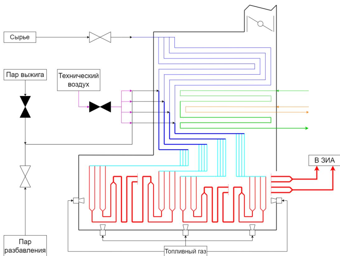
Рисунок 22 – Схема трубчатой печи пиролиза
