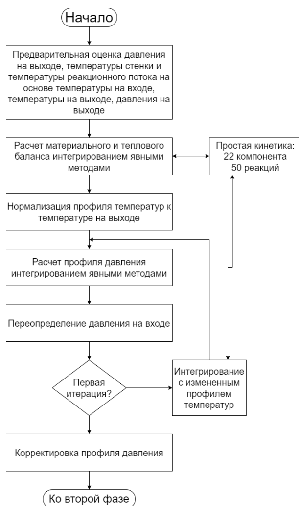
Рисунок 16 – Блок-схема расчета в первой стадии
