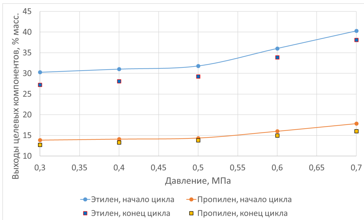
Рисунок 34 – Зависимость выходов этилена и пропилена от давления
