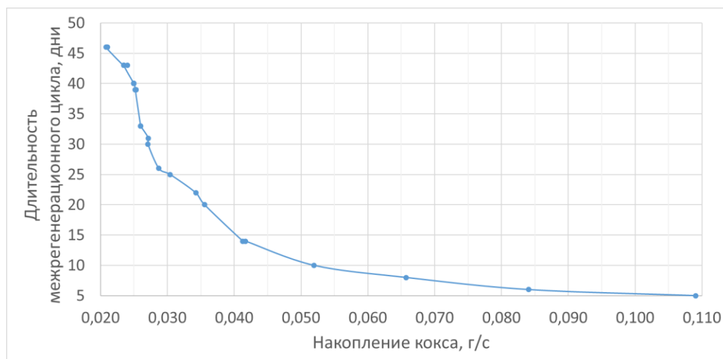
Рисунок 29 – Корреляция между скоростью накопления кокса и длительностью работы печи пиролиза
