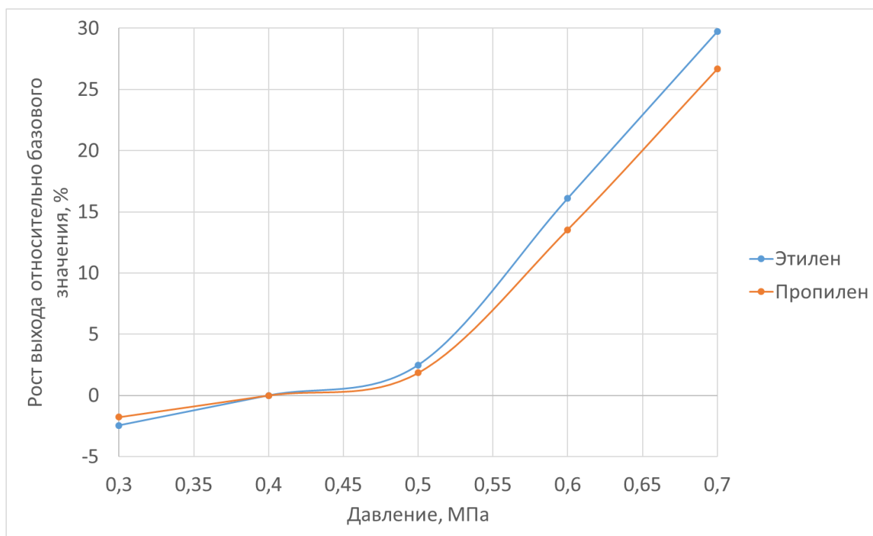
Рисунок 35 – Относительное изменение выходов целевых продуктов при варьировании давления
