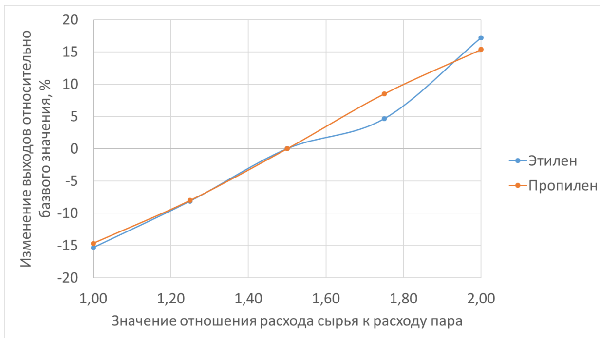
Рисунок 41 – Относительное снижение и рост выходов целевых продуктов при изменении соотношения расходов сырья и пара
