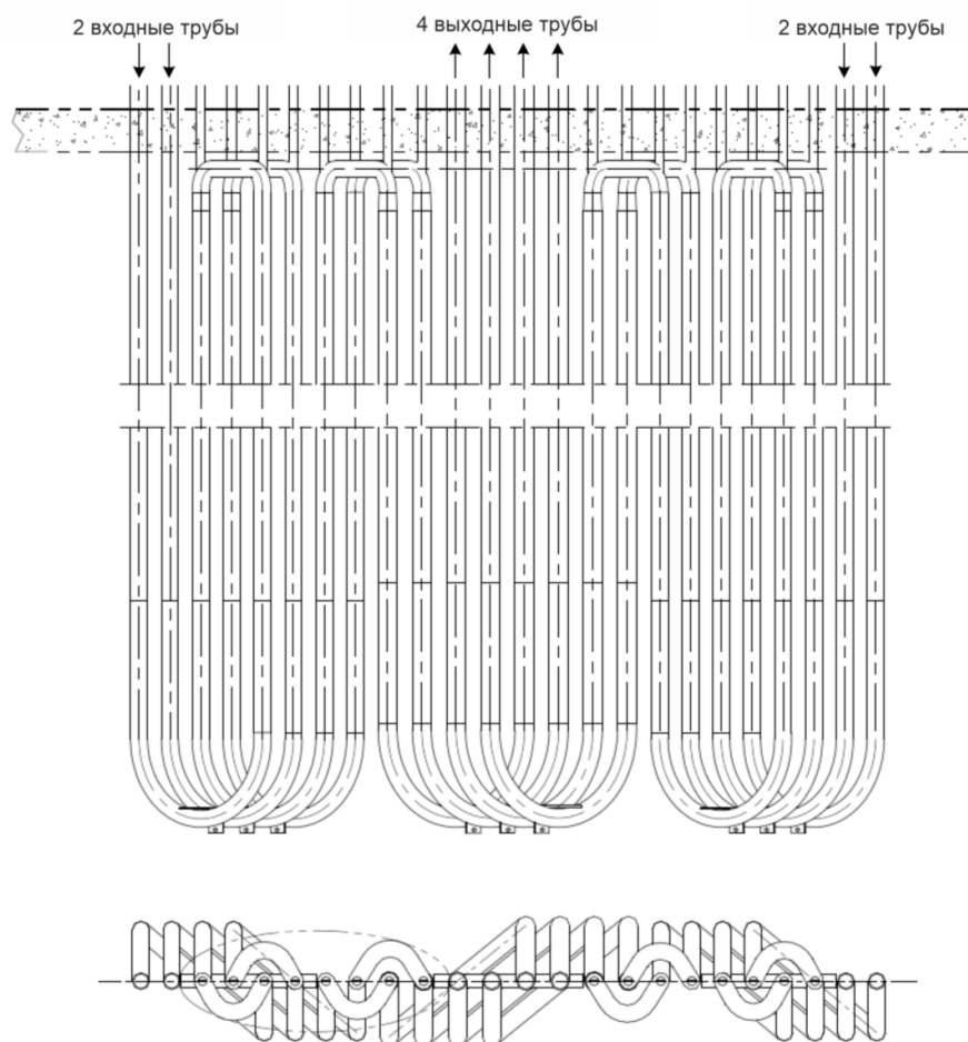
Рисунок 12 – Змеевик PyroCrack 6
