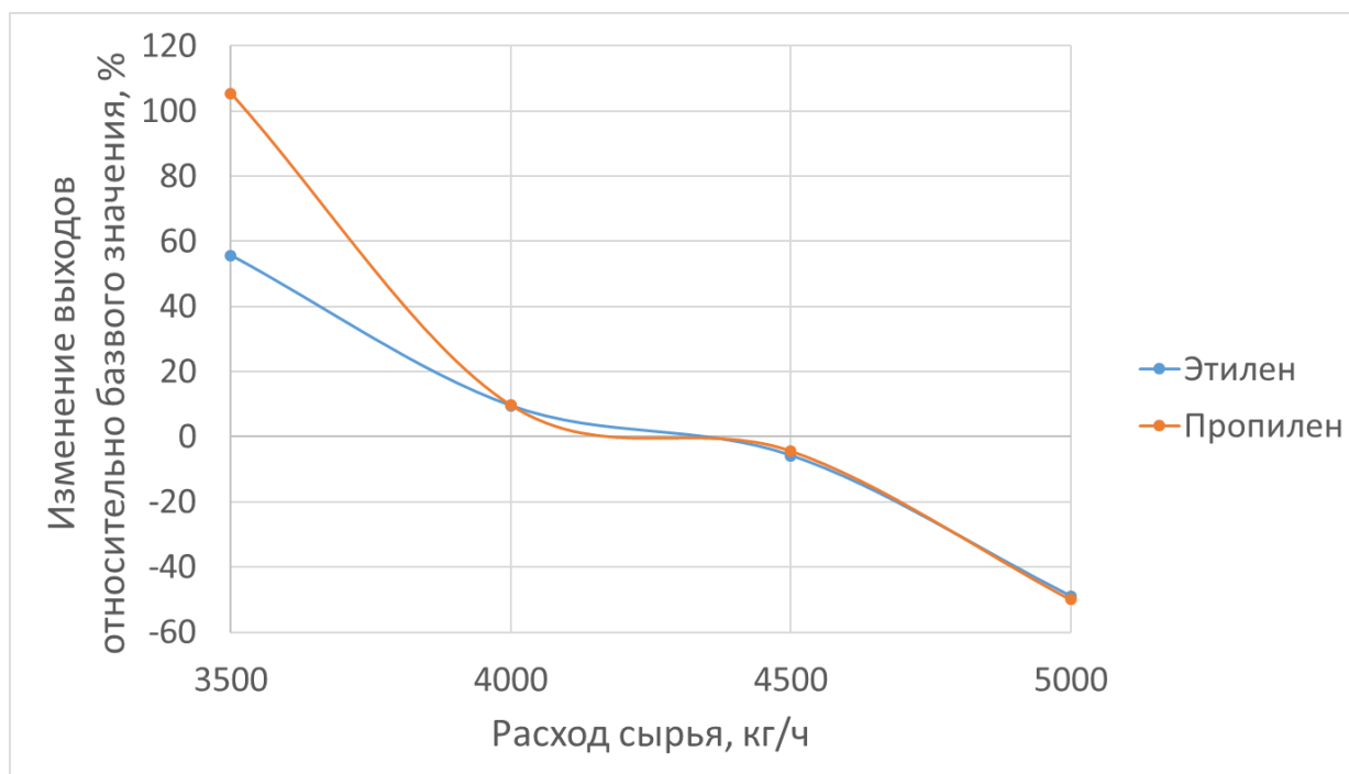
Рисунок 38 – Относительное снижение и рост выходов целевых продуктов при изменении расхода сырья
