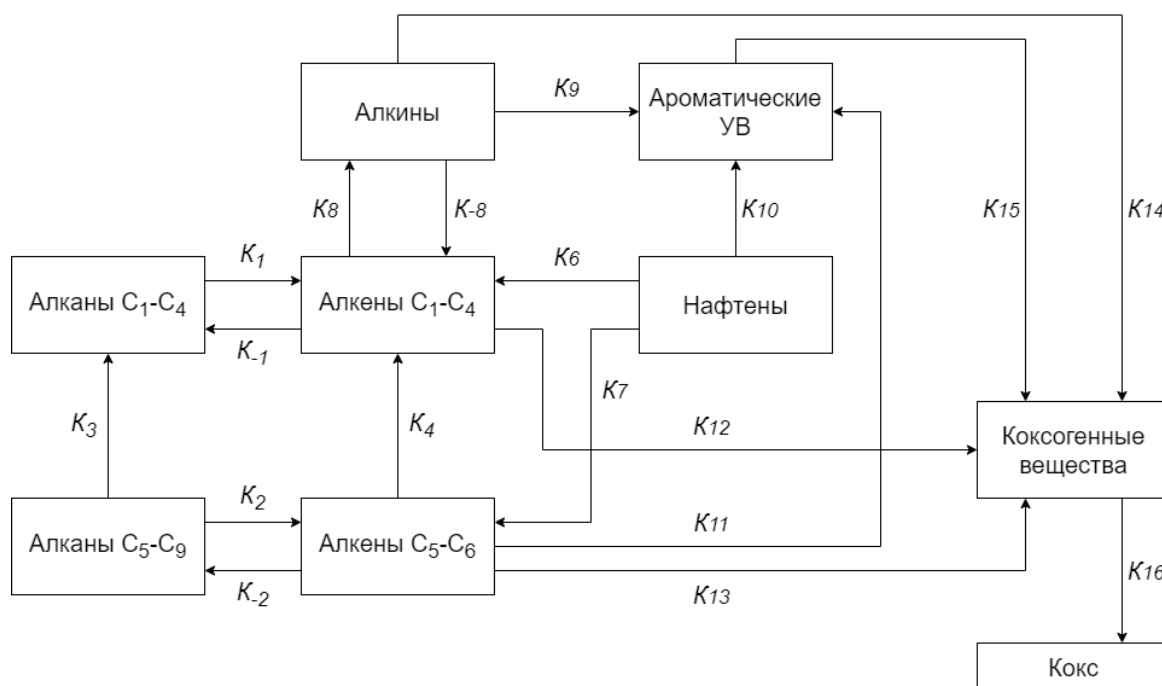
Рисунок 24 – Формализованная схема превращений процесса пиролиза бензиновой фракции
