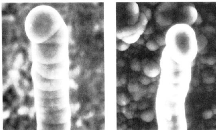
Рисунок 27 – Микрофотография частицы каталитического кокса [97]
