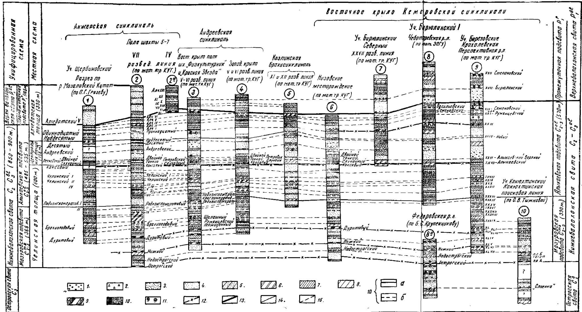
Рис. 1. Параллелизация разрезов нижнебалахонской и верхнебалахонской свит Анжерского и Кемеровского районов. Составили З. Д. Завистовская и Н. М. Белянин. 1 — конгломератовидный песчаник; 2 — пудинговый песчаник; 3 — песчаник крупно- и среднезернистый; 4 — песчаник мелкозернистый, глинистый; 5 — песчаник тонкозернистый, глинистый; 6 — пачки переслаивания песчаника и алевролита; 7 — алевролит; 8 — аргиллит; 9 — углистый аргиллит; 10 — уголь 'а' — пласты рабочие, 'б' — пласты нерабочие; 11 — фауна; 12 — маркирующие горизонты; 13 — стратиграфические границы по унифицированной схеме; 14 — границы толщ по местной схеме Анжерского района; 15 — сопоставление пластов угля. Сокращения: тр. КУГ — трест «Кузбассгеология»; ЗСГУ — Западно-Сибирское геологическое управление.
