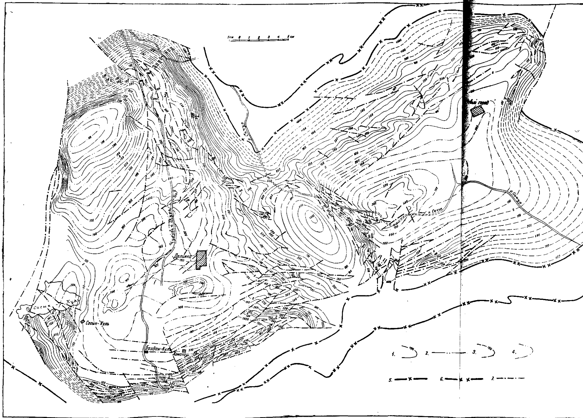
Рис. 2. Структурная карта Карагандинского бассейна. Составила А. А. Булыникова, 1955 г.
