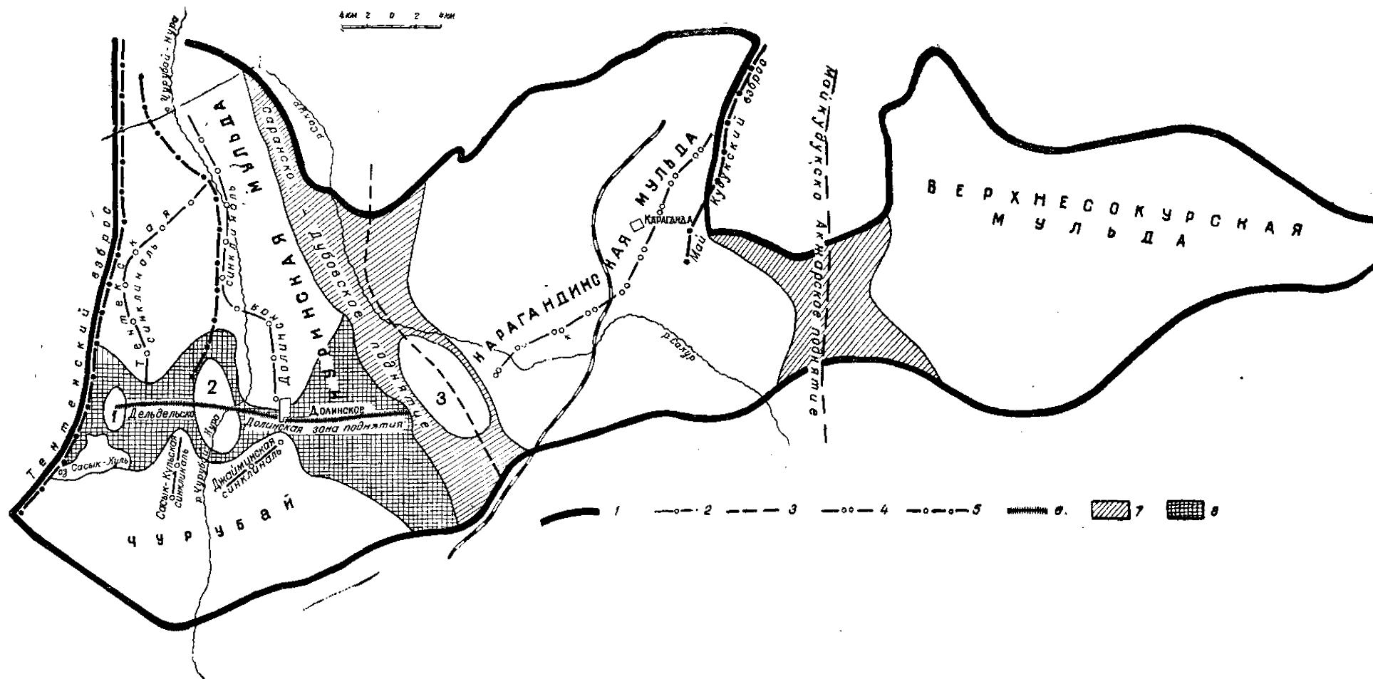
Рис. 1. Схема тектонического районирования Карагандинской впадины.
