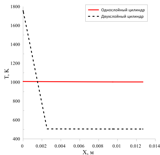
Рис. 5. Распределение температуры в области симметрии для момента времени 100 с
