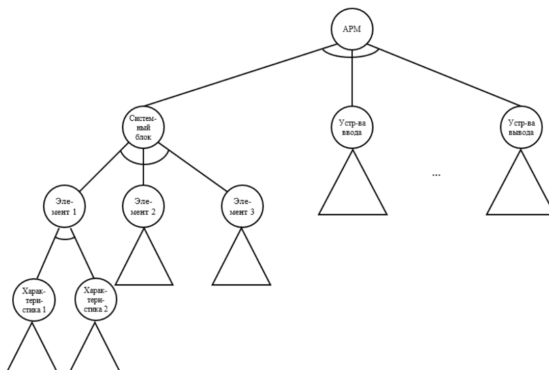
Рис. 2. Дерево И/ИЛИ для представления АРМ (составлено автором)
