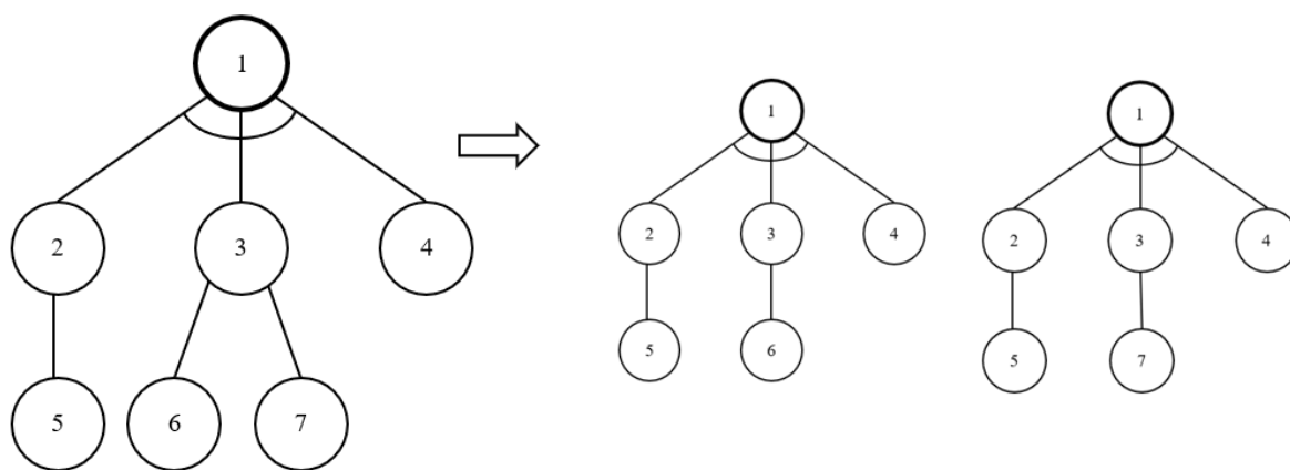
Рис. 1. Пример дерева И/ИЛИ и его вариантов (составлено автором)
