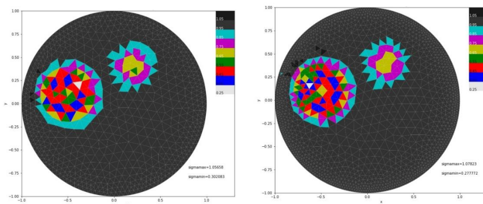
Рис. 1. 2D реконструкция электрической проводимости
