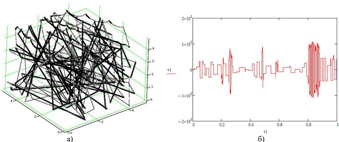
Рис. 1. а) Траектория пробной частицы гелия в выделенном кубе с ребром 5 нм; б) Проекций вектора скорости пробной частицы гелия на ось O y
