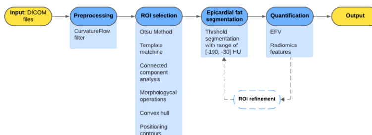
Рис. 2. Схема алгоритма
