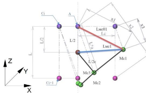
Рис. 2. Характерные точки математической модели сегмента i, i+1 (вид сбоку): (i+1) -ый сегмент (розовый), i -ый сегмент (фиолетовый), i+1 сегмент новое положение (зеленый)
