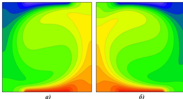
Рис. 2. Поля температур для случая Ra = 10^6 и интенсивности магнитного поля: а) Ha_1 = 100 и Ha_2 = 100 ; б) Ha_1 = 300 и Ha_2 = 100
