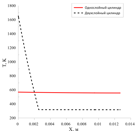
Рис. 4. Распределение температуры в области симметрии для момента времени 20 с
