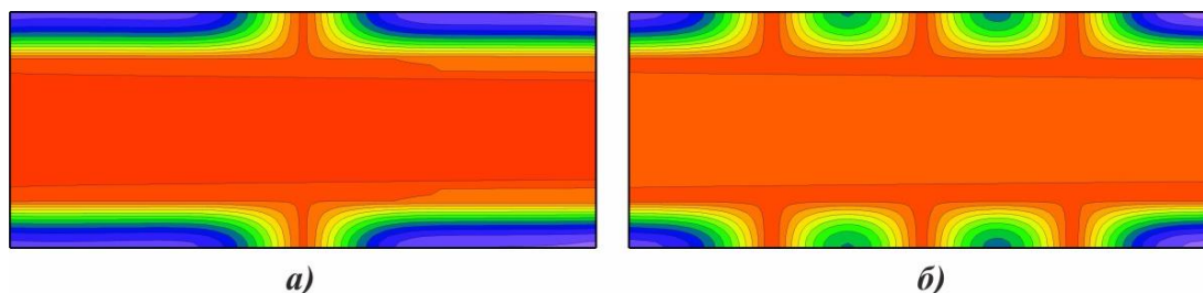
Рис. 2. Распределения температуры в момент времени \tau = 400 для Re = 250 и разного количества ребер
