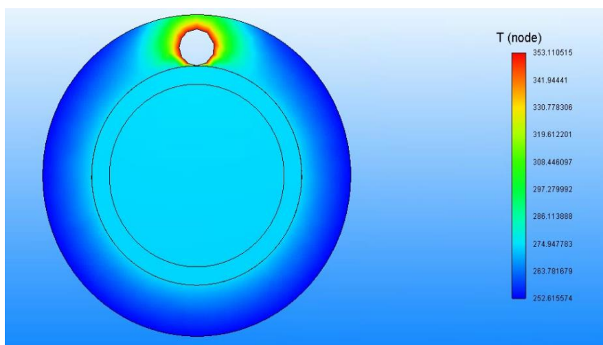
Рис. 2. График распределения температуры в обогреваемом изолированном трубопроводе
