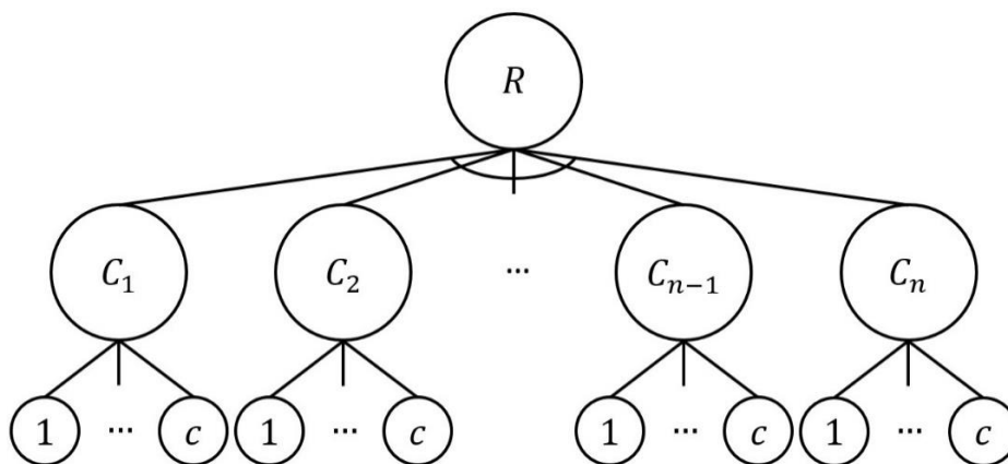
Рис. 2. Структура дерева И/ИЛИ по формуле R = c^n
