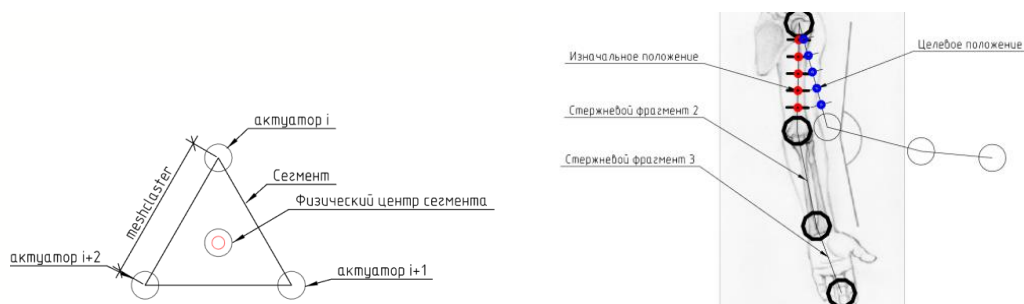
Рис. 1 Математическая модель манипулятора: а) поперечное сечение, б) вид сбоку с 6-ю центрами сегментов
