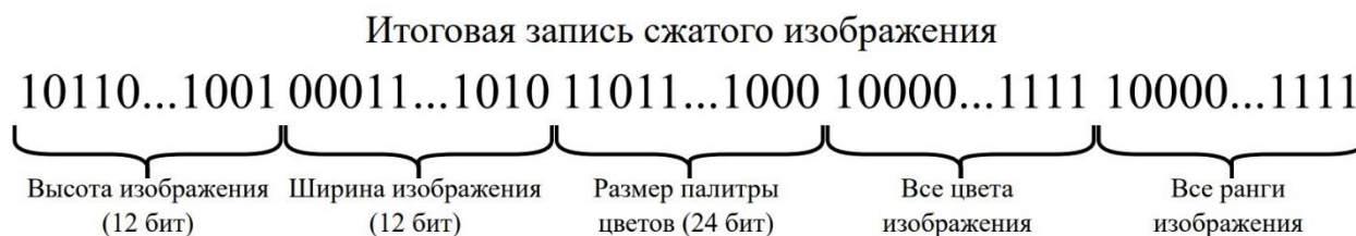
Рис. 3. Структура записываемой строки (пример)
