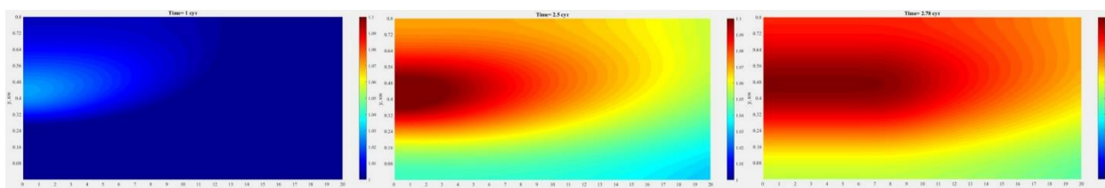
Рис. 5. Распределение концентрации биомассы микроорганизмов X (мг/л) с использованием высоконагружаемого биофильтра
