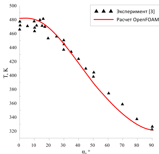
Рис. 3. Распределение температуры на стенке в момент времени t = 4 с
