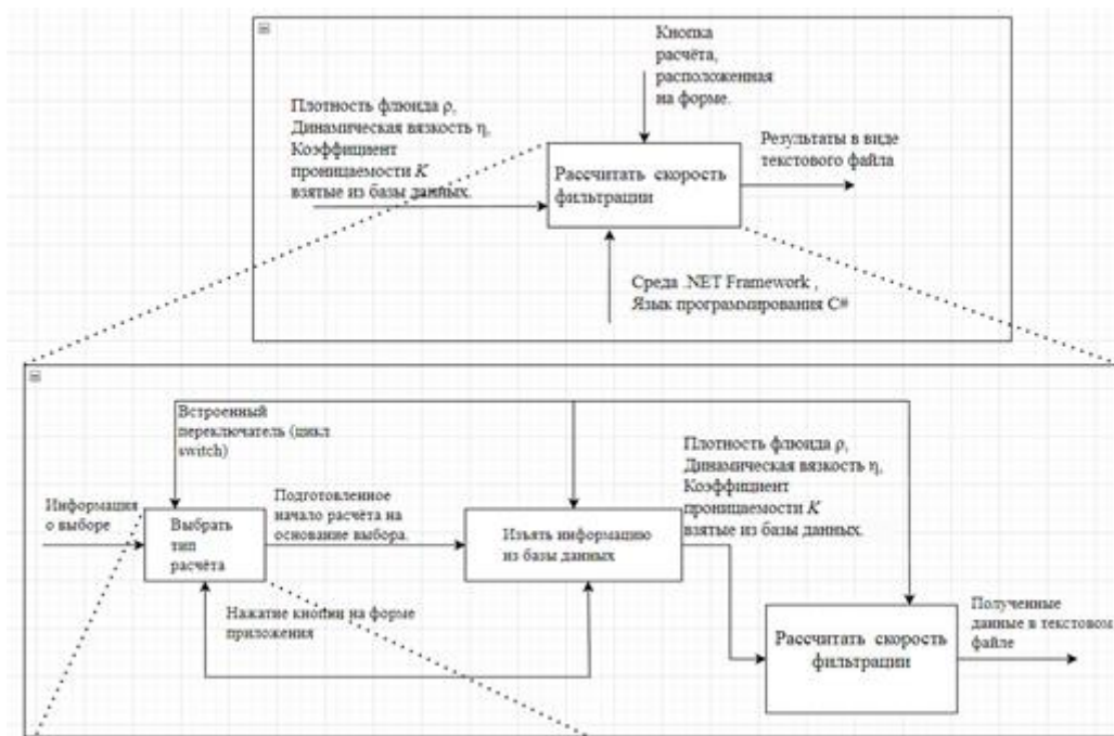
Рис. 1. Описание одного из процессов в нотации IDEF0
