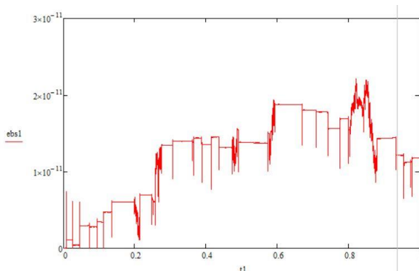
Рис. 2. Относительная погрешность полной механической системы для 1 частицы газа
