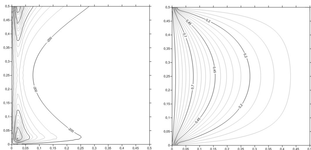
Рис. 3. Вихрь и линии тока для плоского течения
