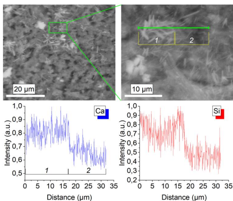
Рис. 1. Электронно-микроскопический снимок цементного камня
