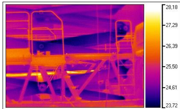
Рис. 4. Термограмма испытаний
