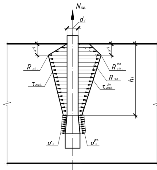
Рис. 3. Расчетная схема напряжений в бетоне в стадии I
