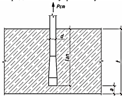
Рис. 1. Схема анкеровки гибкой связи в бетон: d – диаметр гибкой связи; L1 – длина конического участка анкерного уширения; L2 – длина анкерного уширения; l_{\text{ан}} – глубина анкерования гибкой связи в бетон; a – защитный слой; t – толщина бетонного слоя
