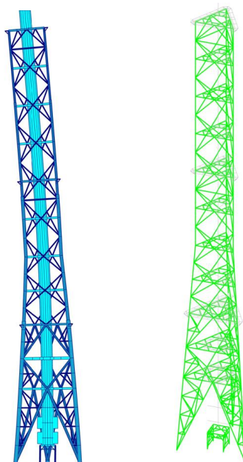
Рис. 2. Первая форма собственных колебаний и результаты поэлементной проверки элементов существующего каркаса
