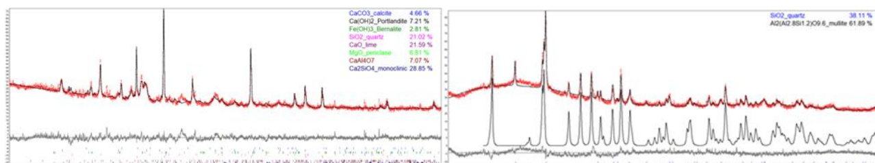
Рис. 1. Рентгенограмма: а) БП4; б) ЗО
