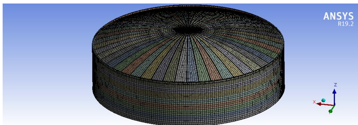
Рис. 1. Конечно-элементная модель резервуара
