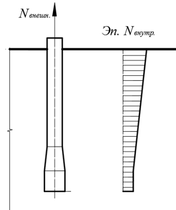
Рис. 2. Расчетная схема внутренних усилий N_{\text{внутр.}} в композитном стержне при увеличении внешней силы N_{\text{внешн.}}
