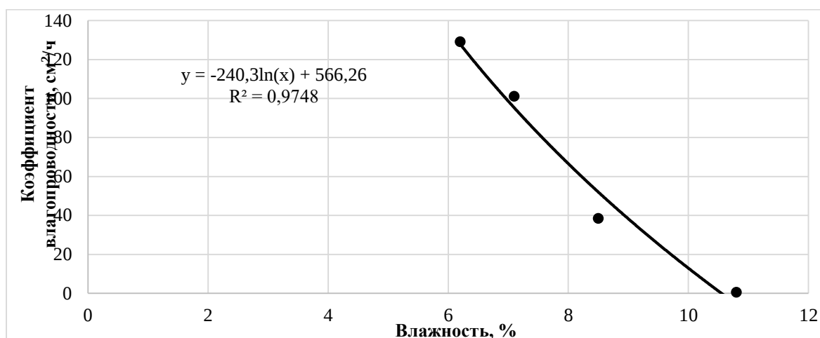
Рис. 1. Зависимость коэффициента влагопроводности песка мелкого от его влажности (при плотности 1,74 г/см³)
