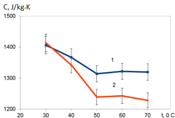
Рис. 3. Зависимость удельной теплоемкости от температуры: связующее 1 – БК-2055, 2 – СКМС-30АРК
