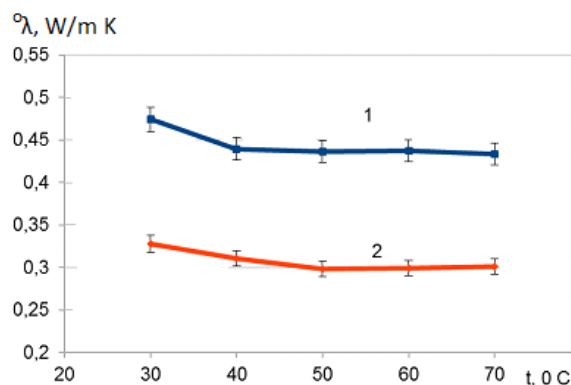
Рис. 2. Зависимость коэффициента теплопроводности от температуры: связующее 1 – БК-2055, 2 – СКМС-30АРК
