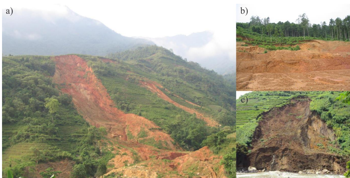
Рис. 2. Фотографии оползней: в коммуне Финнган (а), в центре района Батсат (b), в коммуне Мьонгхум (с). Фото Ч.К. Нгуена
