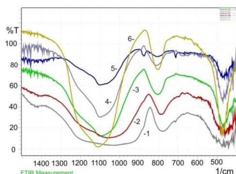
Рис. 4. Фрагменты спектров ИК-поглощения: 1 – техническое силикатное стекло; 2 – плавённый кварцит; 3 – оптическая «кварцевая» трубка; 4 – оптическое «кварцевое» стекло; 5 – кварцевая пластина; 6 – наноразмерный диоксид кремния, полученный методом магнетронного распыления
