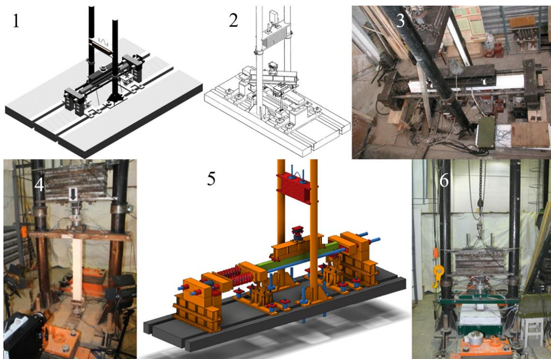
Рис. 9. Экспериментальные стенов на базе копровой установки: 1 – косоое внецентренное кратковременное динамическое растяжение; 2 – кратковременное динамическое кручение с изгибом; 3 – косоое внецентренное кратковременное динамическое сжатие; 4 – кратковременное динамическое сжатие колонн; 5 – продольное статическое обжатие с кратковременным динамическим поперечным воздействием; 6 – испытания на продавливание при действии кратковременной динамической нагрузки
