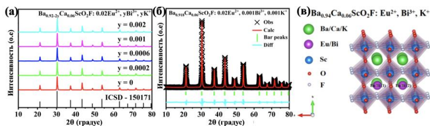
Рис. 1. Рентгеновские дифрактограммы \text{Ba}_{0.92-2y}\text{Ca}_{0.06}\text{ScO}_2\text{F}: 0.02\text{Eu}^{2+}, y\text{Bi}^{3+}, y\text{K}^+ ( y = 0, 0.0002, 0.0006, 0.001 и 0.002 ) люминофора (а), (б). Кристаллическая структура \text{Ba}_{0.94}\text{Ca}_{0.06}\text{ScO}_2\text{F}: \text{Eu}^{2+}, \text{Bi}^{3+}, \text{K}^+ , полученная уточнением Ритвельда (в)
