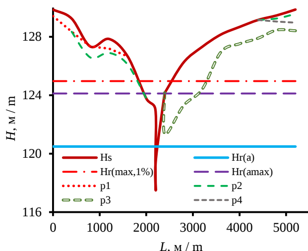
Рис. 5. Поперечный профиль долины р. Бакчар в 87 км от истока; H_s – высотная отметка поверхности водосбора или дна реки; H_r(a) , H_r(max, 1\%) , H_r(amax) – средний годовой, максимальный с обеспеченностью 1 % и средний максимальный уровни воды в р. Бакчар; p – высотная отметка нижней поверхности слоя торфяной залежи с преобладанием торфов верхового сфагново-мочажинного ( p_1 ) и низинных осокового ( p_2 ), травяного ( p_3 ) и березового ( p_4 ) торфов
