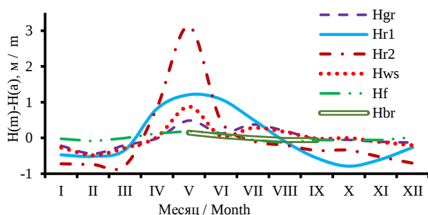
Рис. 3. Внутригодовое изменение отклонений среднемесячных уровней воды H(m) от их среднегодовых значений H(a) ; уровни воды: Hgr – в скважине 89р (с. Каргала; возраст отложений aQ_{IIb} ; средний уровень за 1965–1995 гг. Hgr(a)=99,39 м; отметка устья скважины 109,40 м); Hr1 – уровень воды р. Оби у п. Победа (в среднем за 1967–2015 гг. Hr1(a)=72,76 м); Hr2 – уровень воды р. Шегарки у с. Бабарыкино (в среднем за 1967–2005 гг. Hr2(a)=89,91 м); Hws – расчетный уровень грунтовых вод на водоразделе рек Оби и Шегарки ( Hws(a)=102,00 м при среднем расстоянии водораздела от р. Оби 23,8 км с отметками 115–120 м); Hf – уровень вод на Баксинском болоте (скважина 104, осоково-тростниковый кочкарник; в среднем за 1961–1969 гг. Hf(a)=140,84 м при средней высоте поверхности болота 141,11 м [37]); Hbr – уровень вод на верховом сосново-сфагново-кустарничковом участке Васюганского болота (в среднем за 1998–2008 гг. Hbr(a)=112,13 м [41])
