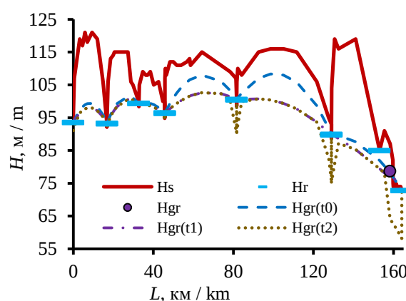
Рис. 4. Профиль АР–ОР (рис. 1, б) и уровни подземных вод в голоцене: H_s – поверхность водосбора или дна рек; H_r – современный среднесезонный уровень речных вод; H_{gr} – современный среднесезонный уровень воды в скважине 63р в с. Мельниково; H_{gr}(t_0) – расчетный среднегодовой уровень подземных вод в среднем за 1967–2005 гг.; H_{gr}(t_1) – расчетный уровень подземных вод при условии, что все болота низинного типа, а их площадь в 1,7 раз больше, чем в настоящее время (ориентировочно 1,5...2,0 тыс. лет назад); H_{gr}(t_2) – расчетный уровень подземных вод при условии, что все болота низинного типа с глубиной не более 0,3 м, а их площадь в 2 раза меньше, чем в настоящее время (ориентировочно 4 тыс. лет назад)
