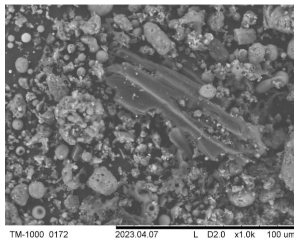
Рис. 2. Микрофотография золошлаковых отходов ТЭЦ-1 Fig. 2. Microphotographs of ash and slag waste CHPP-1
